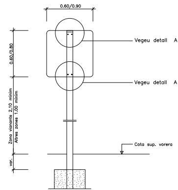
Detall constructiu. Senyal quadrada
