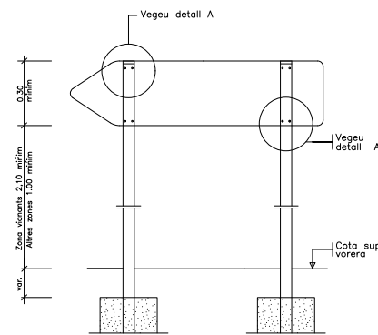
Detall constructiu. Senyal de direcció pròpia
