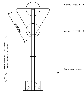
Detall constructiu. Senyal triangular invertida
