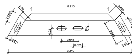
Fabricada en planxa de ferro galvanitzada en calent de 2 mm. d' espesor
