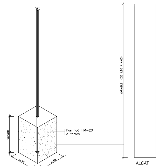
AXONOMÈTRICA
