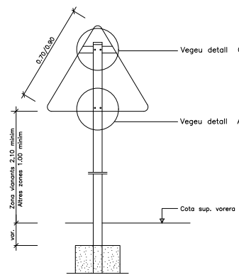
Detall constructiu. Senyal triangular
