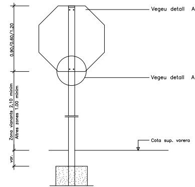
Detall constructiu. Senyal octogonal
