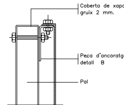
Subjecció amb clau
