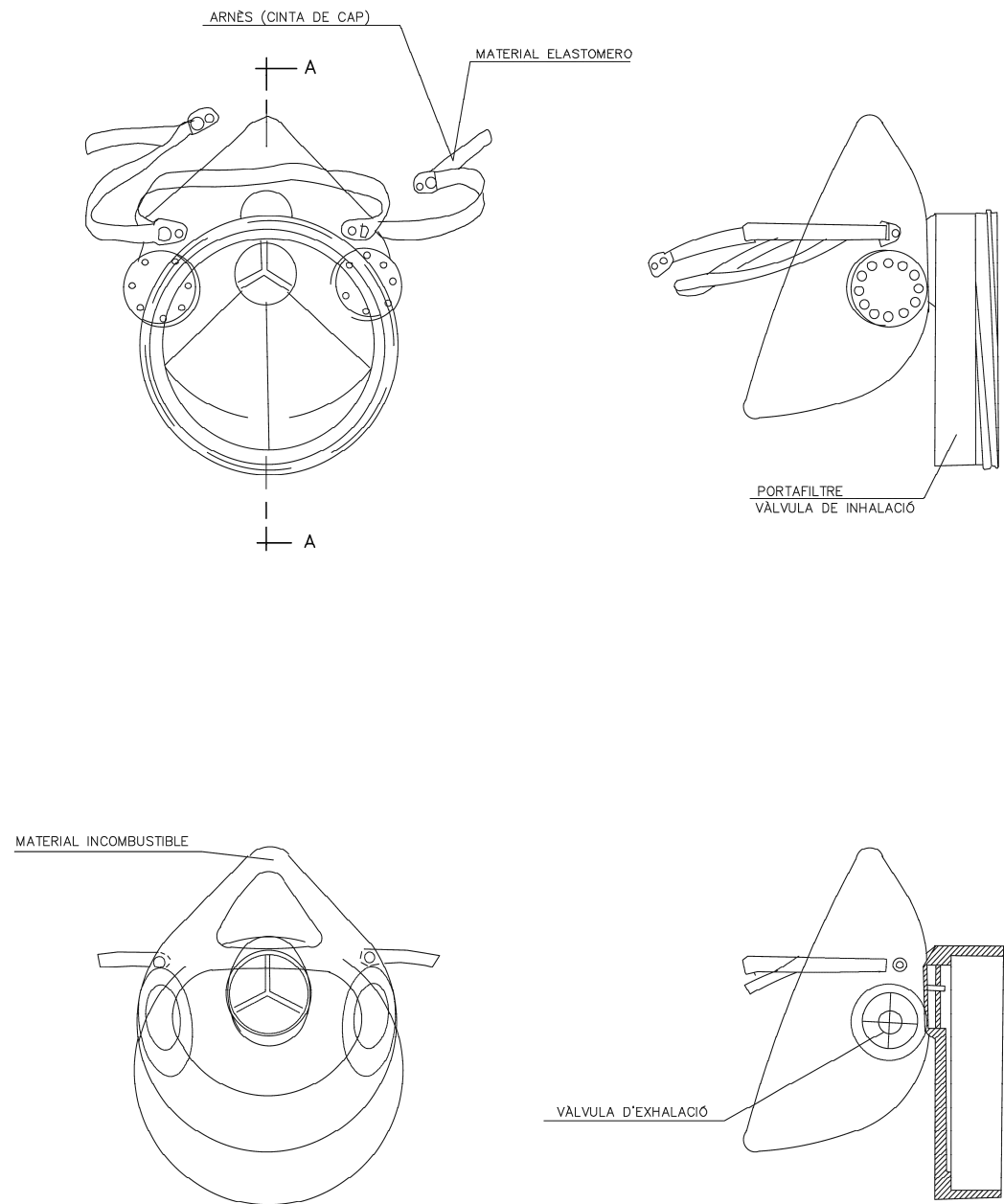
SECCIÓ A-A
