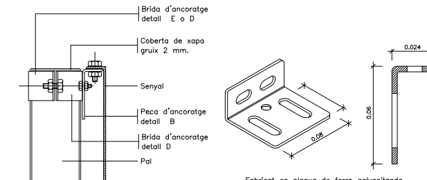
Subjecció amb brida
