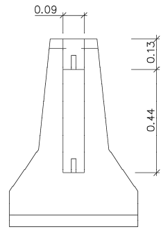
ALÇAT TRANSVERSAL
