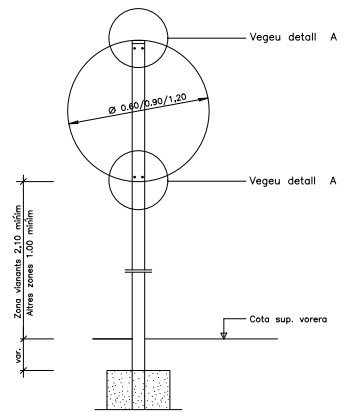
Detall constructiu. Senyal circular
