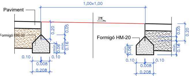
Secció A-A'
