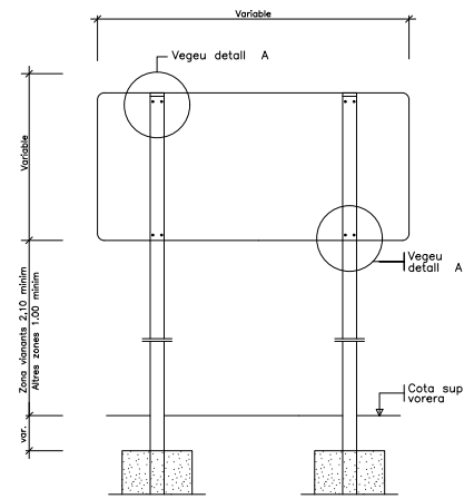
Detall constructiu. Senyal rectangular horitzontal
