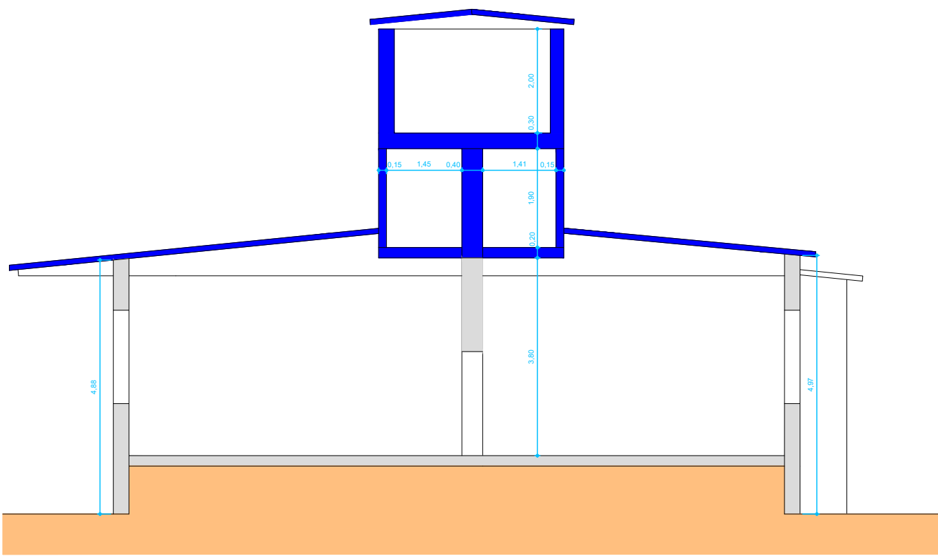
SECCIÓ - ENDERROCS
