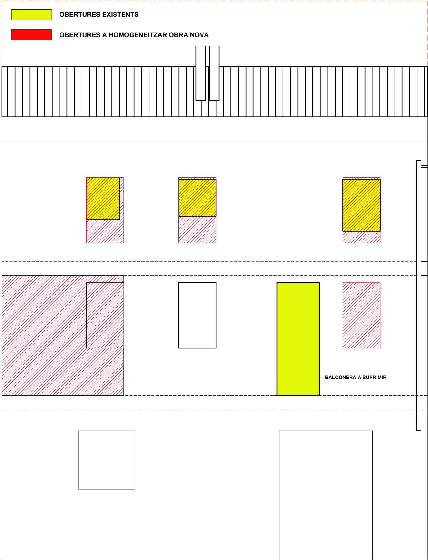
ALÇAT POSTERIOR
