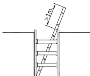
BAIXADA A RASA
