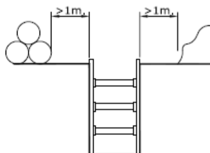
DISTÀNCIA APLECS (rasa apuntalada)
