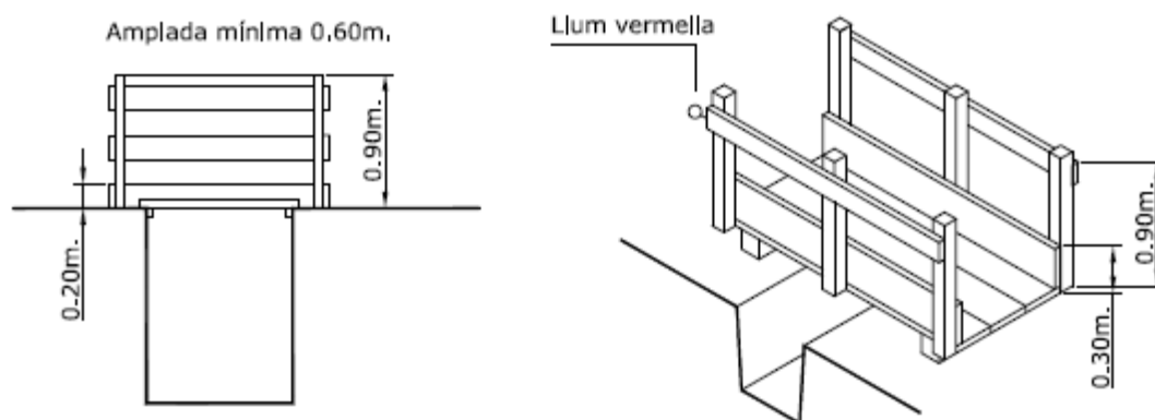
DETALL PASSARELLA VIANANTS
