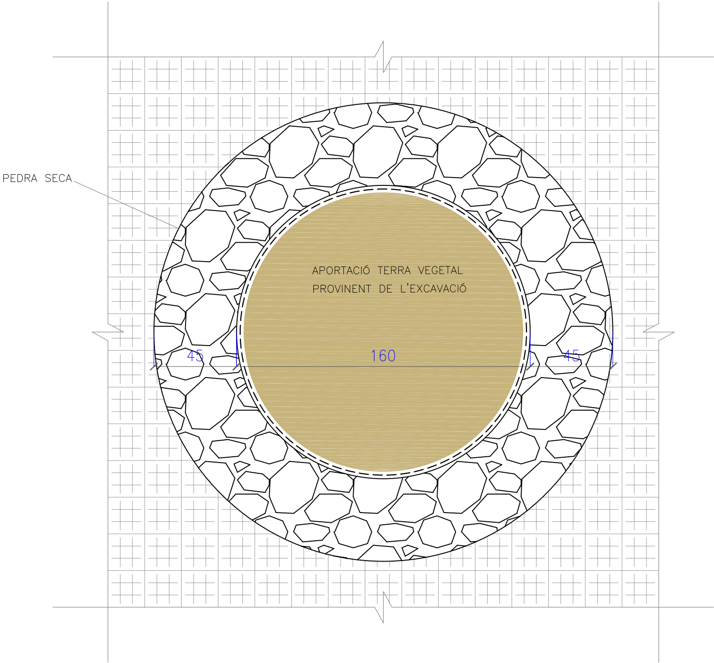
SECCIÓ HORIZONTAL, 1/20
