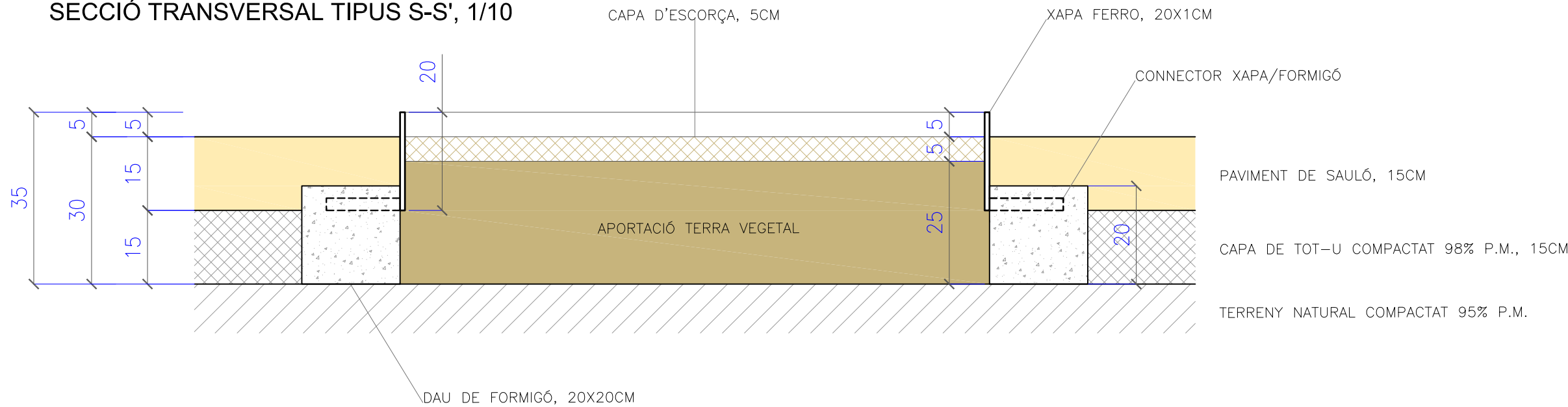
SECCIÓ TRANSVERSAL TIPUS S-S', 1/10
