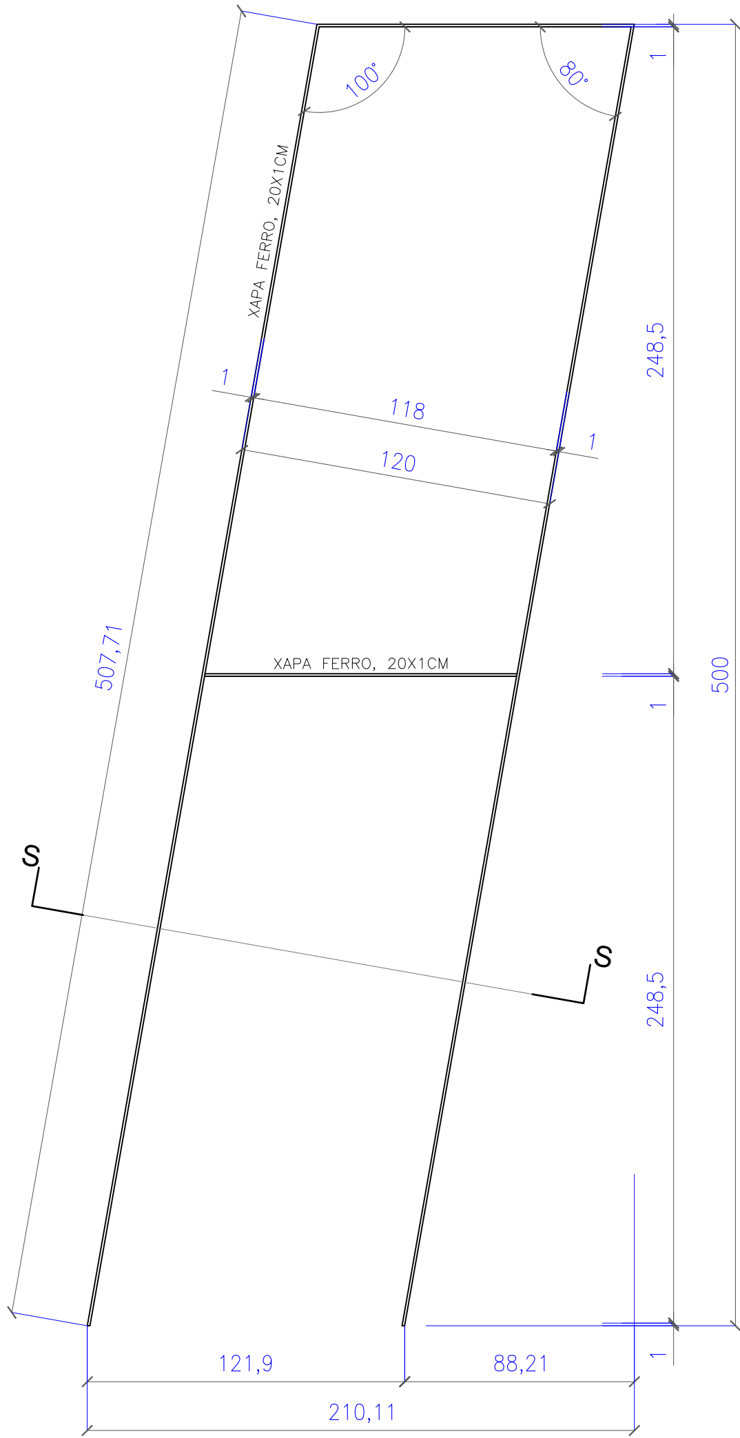
PLANTA, 1/20 JARDINERA TIPUS J-2
