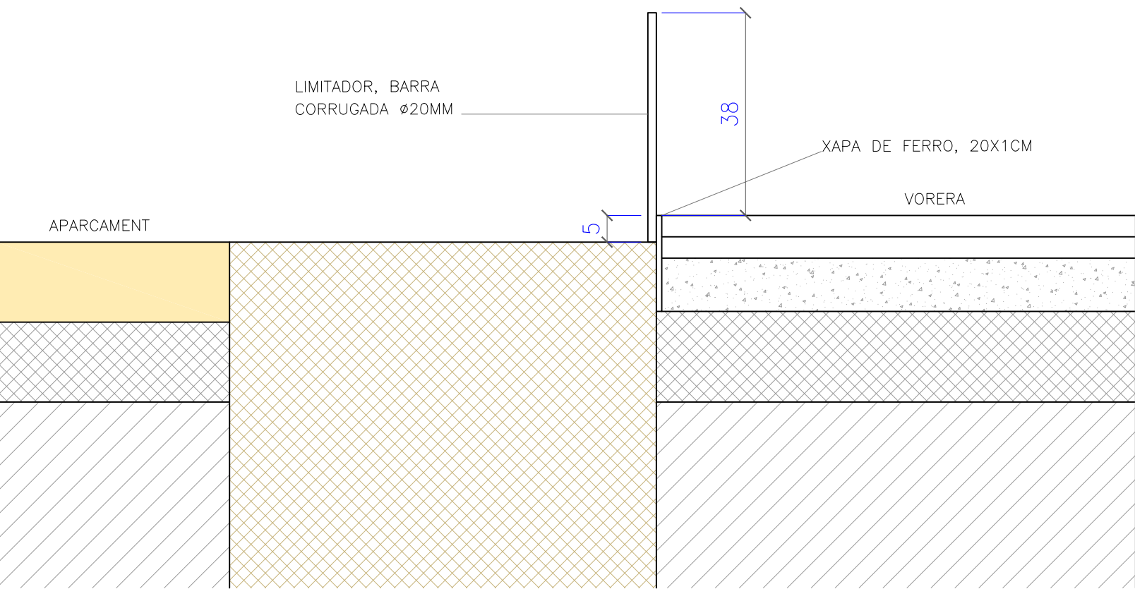
SECCIÓ TRANSVERSAL TIPUS S-S', 1/10
