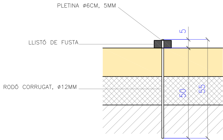
DETALL LLISTÓ DE FUSTA, 1/10
