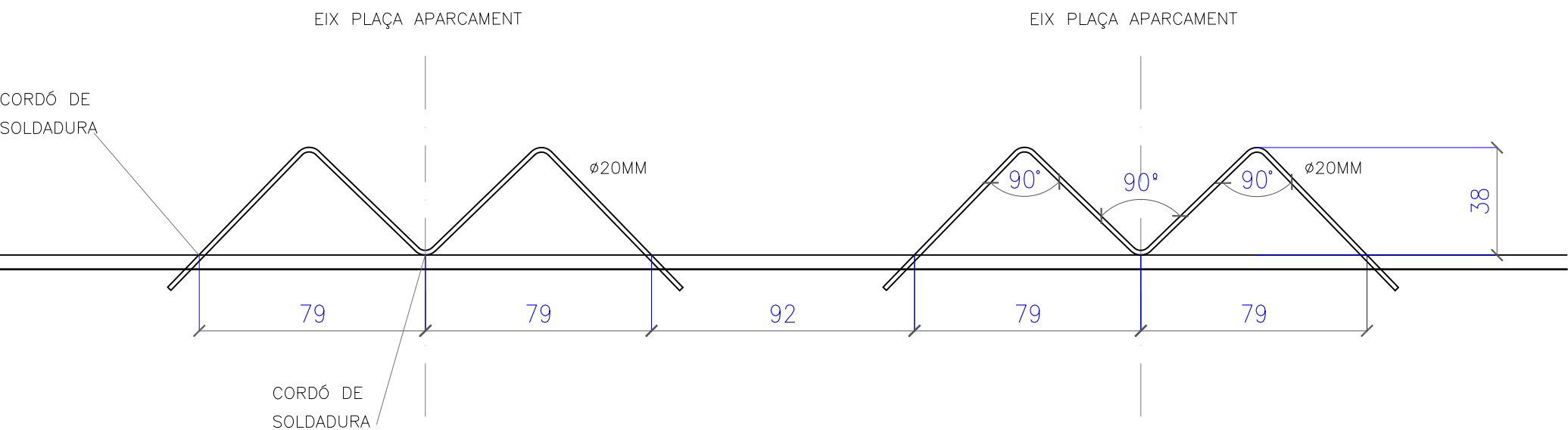
ALÇAT LIMITADORS, 1/20 (VISTA DES DE L'APARCAMENT)
