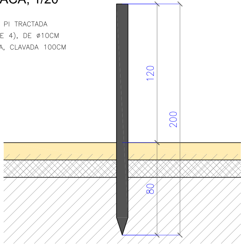
DETALL ESTACA, 1/20
