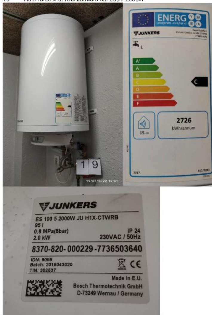
19 Acumulador d'ACS Junkers 95l 230V 2000W
