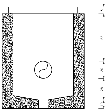
SECCIÓ E-F
