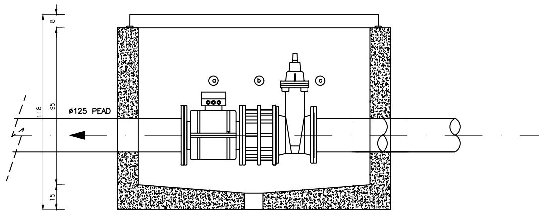
SECCIÓ C-D
