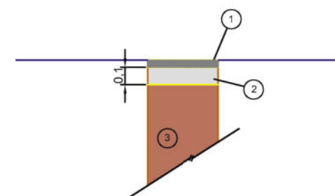
SECCIÓ TIPUS PER REPOSICIÓ DE PAVIMENT AMB LLOSES
