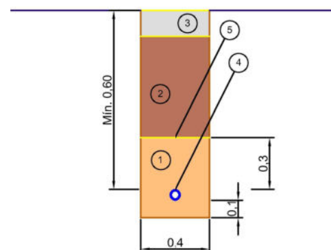
SECCIÓ TIPUS D'EXCAVACIÓ I REBLERT DE RASA
