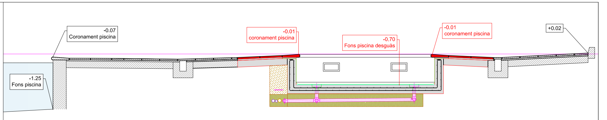
Secció B-B' E/1:50
