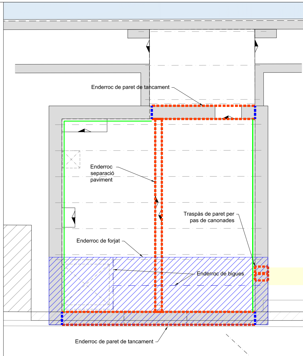
ZONA DEPURADORA E/1:50
