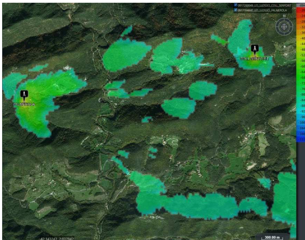
Cobertura LoRaWAN
