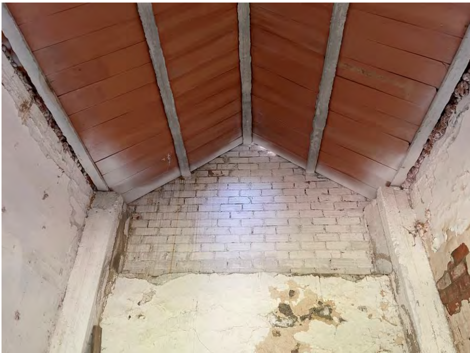
Imatge 14: Vista interior de la capella a la part central del cos nord de bigues de formigó prefabricades i encadellat ceràmic.
