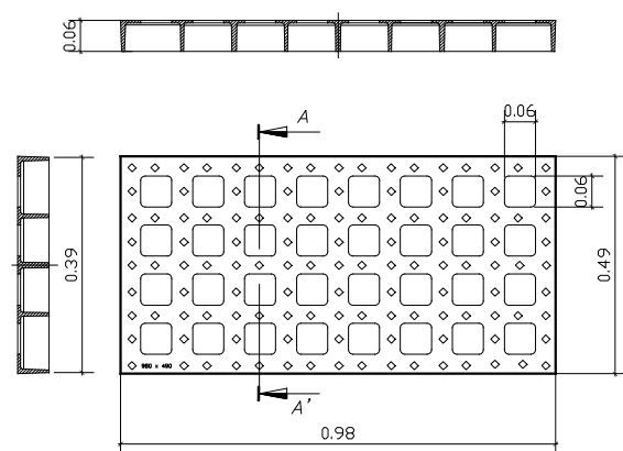
REIXA INTERCEPTORA e: 1/10
