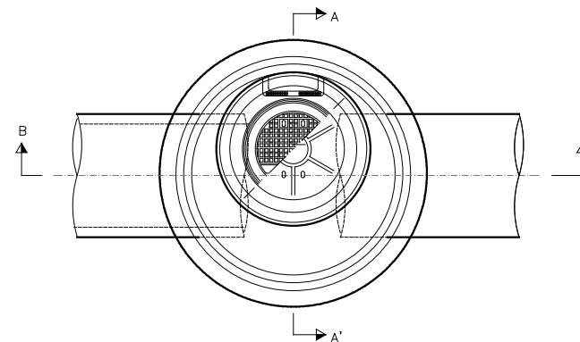
PLANTA POU DE REGISTRE
