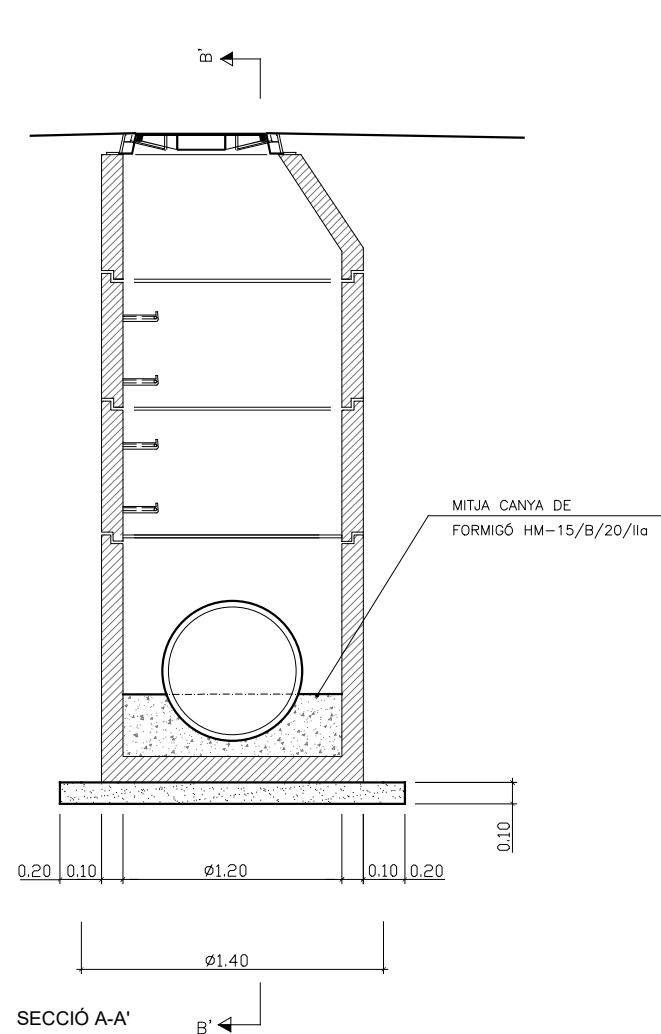
POU DE REGISTRE e: 1/30
