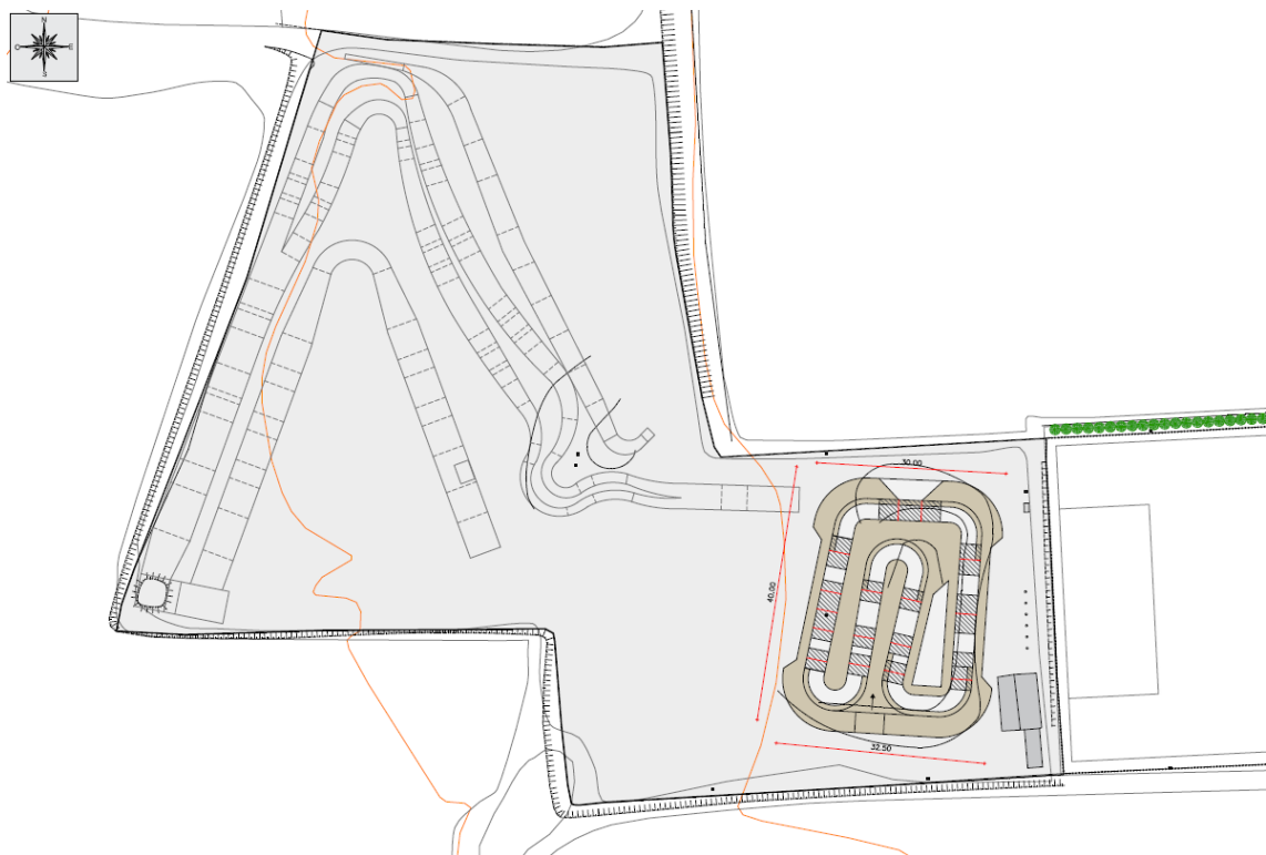
Figura 3. Planta proposta
