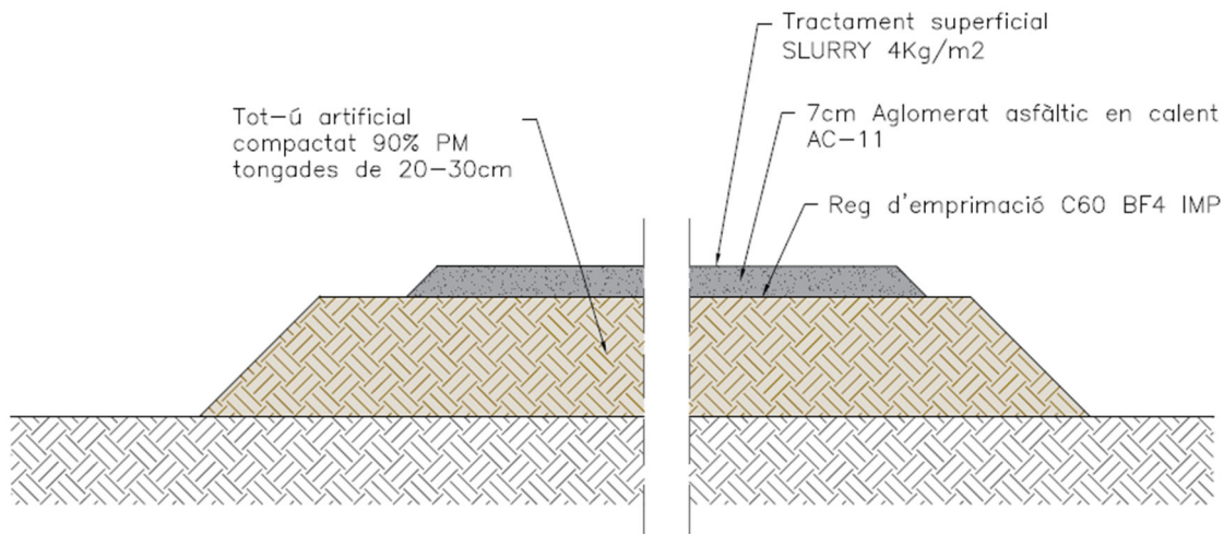
Figura 4. Secció tipus pumptrack
