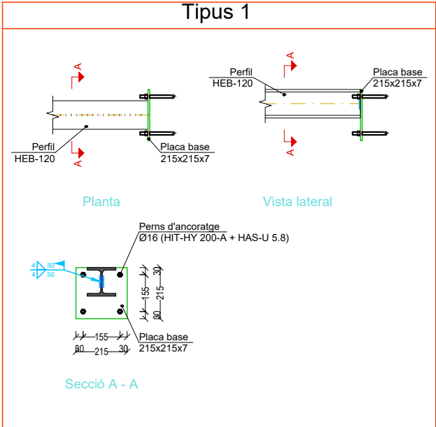
PLACA D'ANCORATGE
