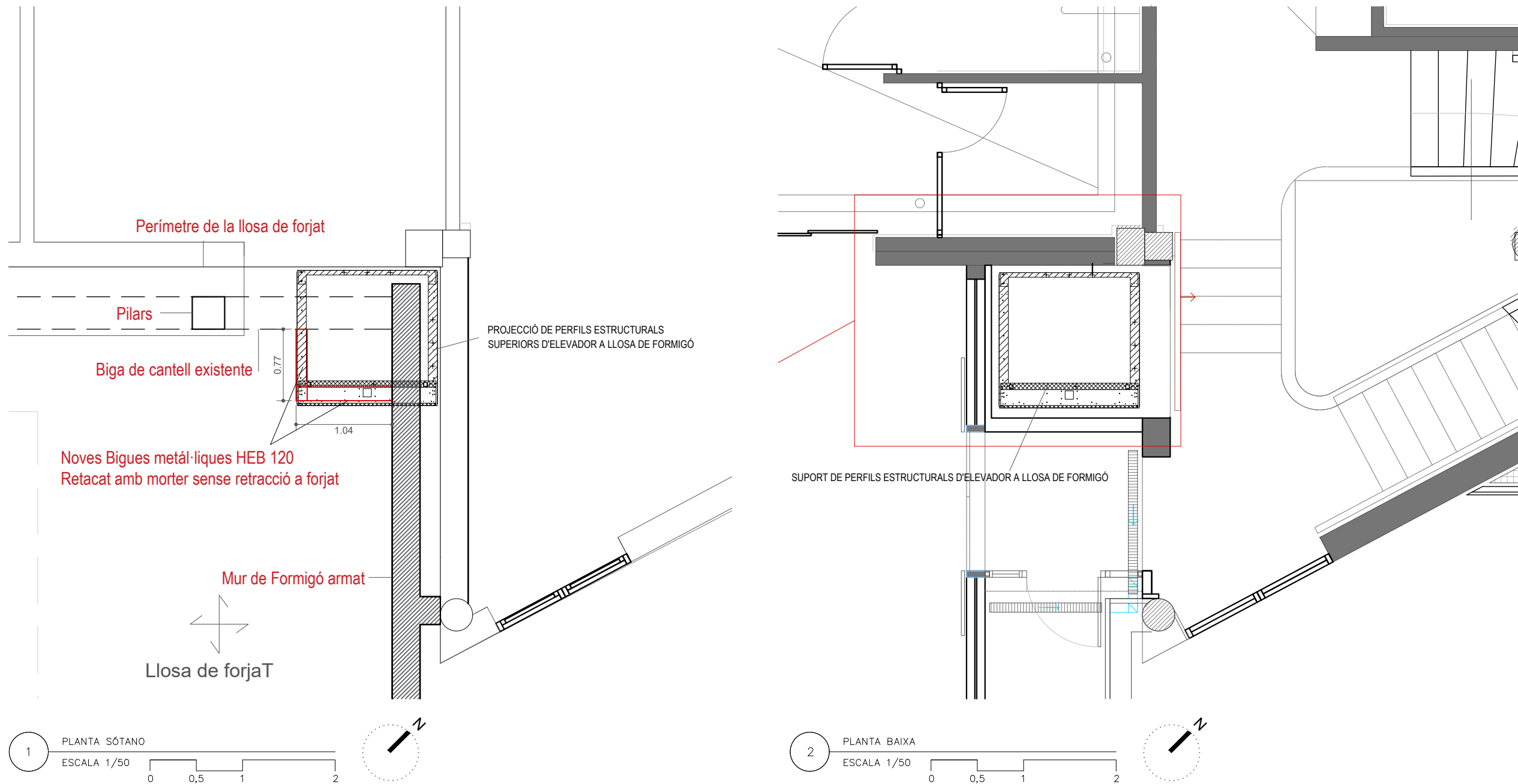
PLANTILLA DE CÀRREGA DE L'ELEVADOR
