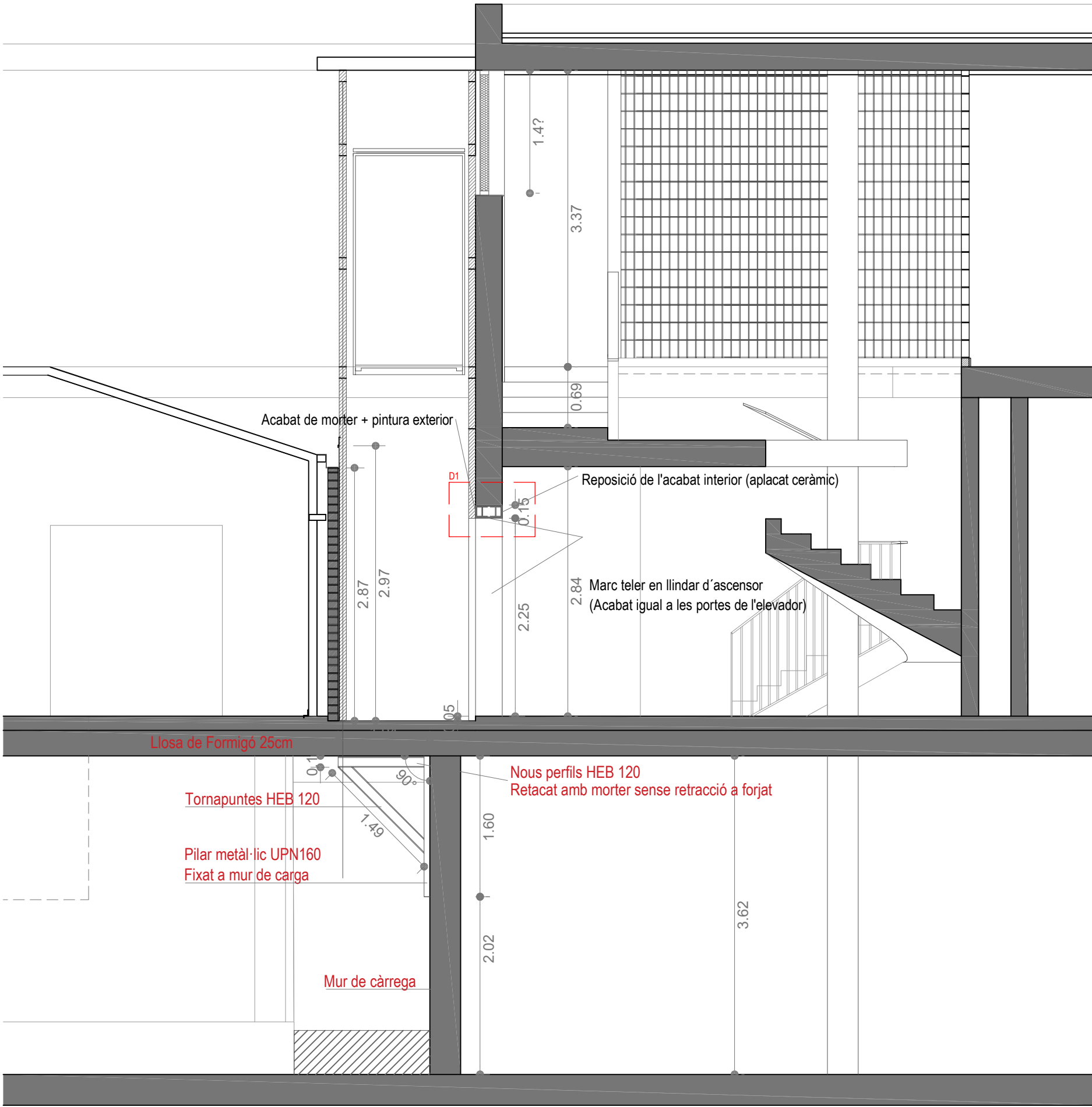
1 SECCIÓ 1B ESCALA 1/50
