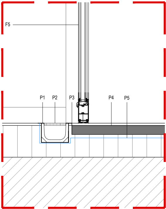
01 Detall 1 AP06 ESCALA 1/10 0 0.1 0.2
