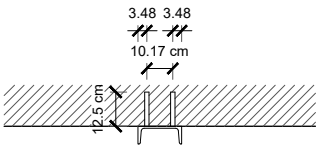
PLANTA UPN-160* E:1/20
