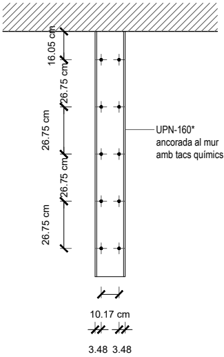
ALÇAT UPN-160* E:1/20
