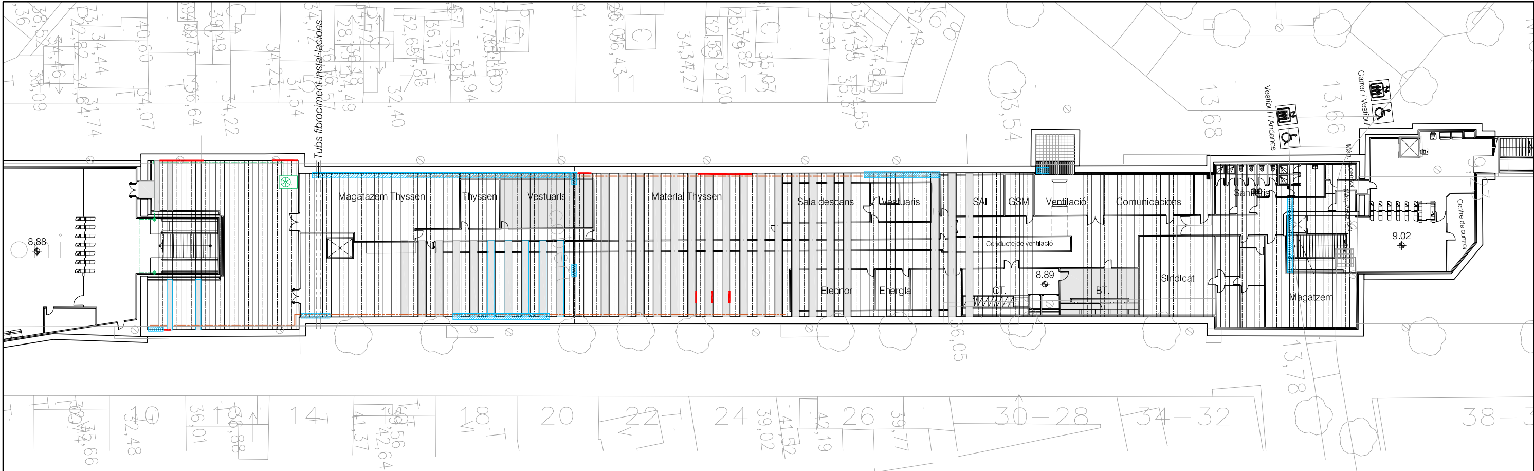
Planta vestíbul Escala 1:400
