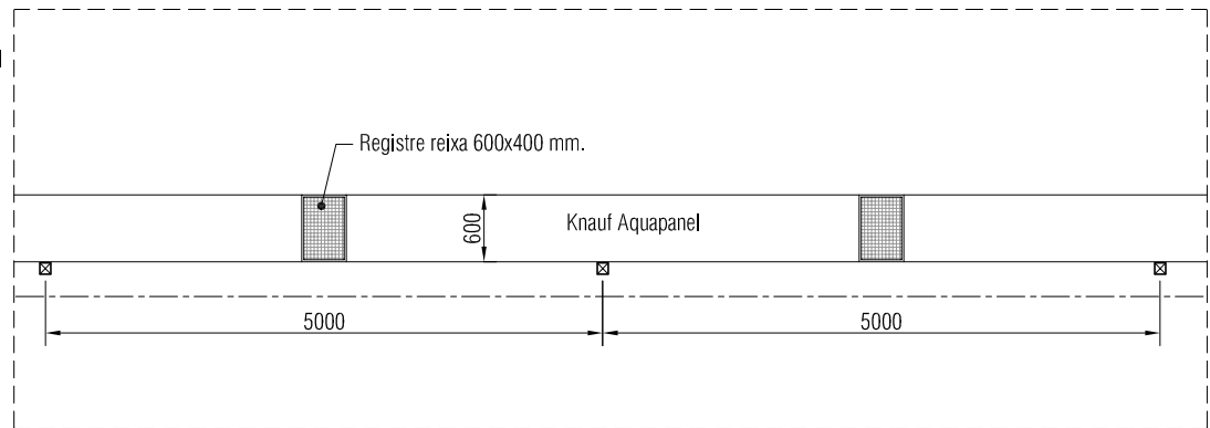
Detall 1 (alçat) Escala 1:75
