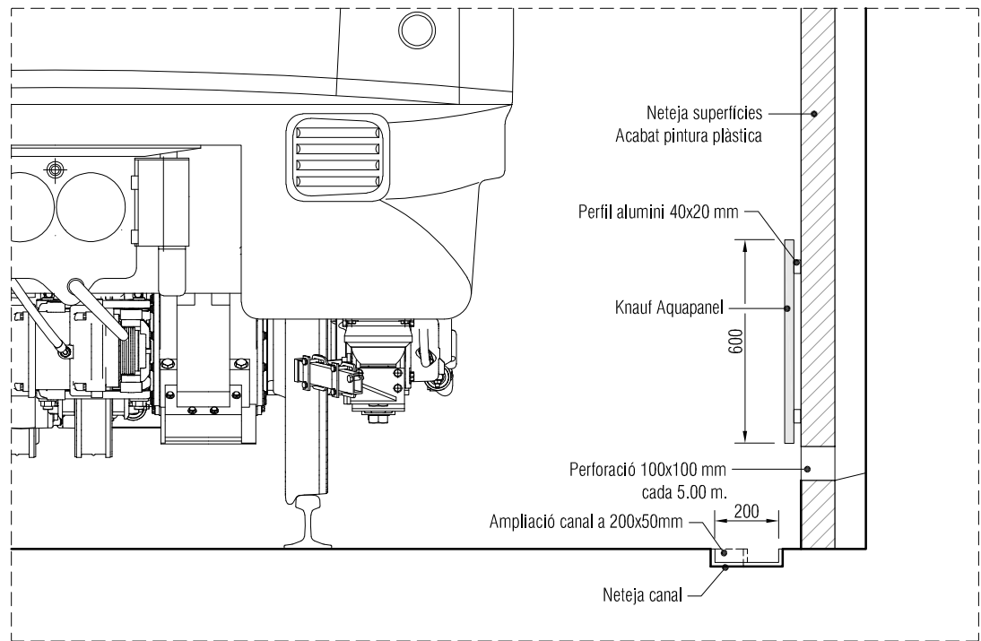
Detall 1 (secció transversal) Escala 1:20
