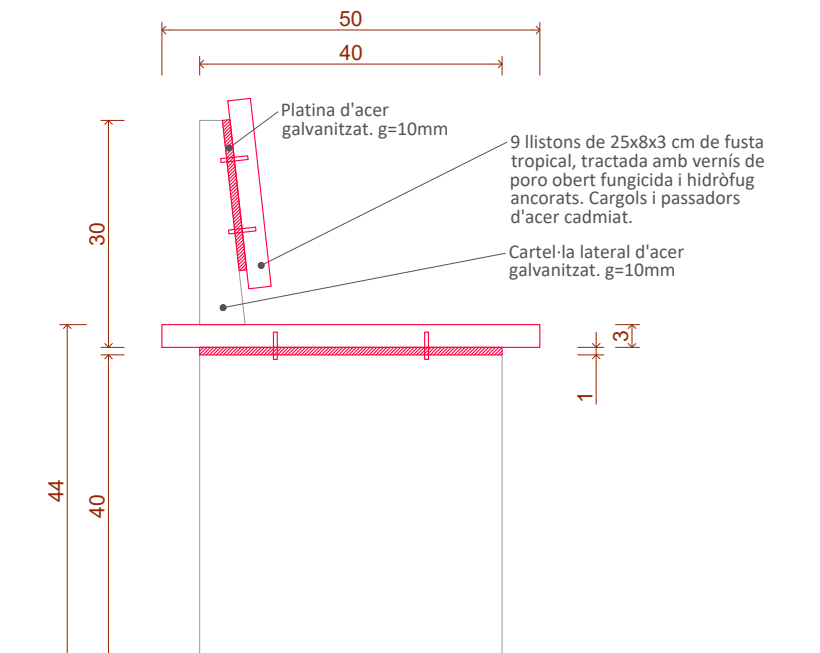
SECCIÓ RASPATLLER (no inclòs a projecte)
