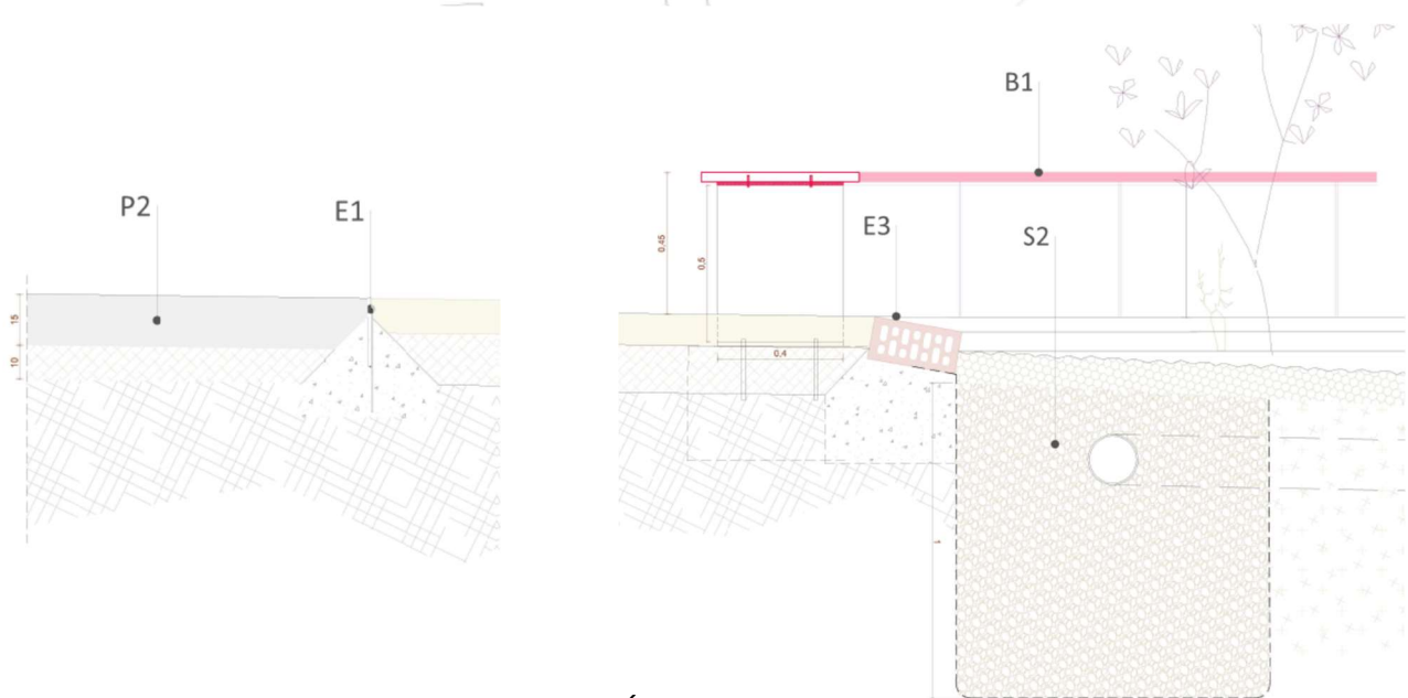
SECCIÓ CONSTRUCTIVA
