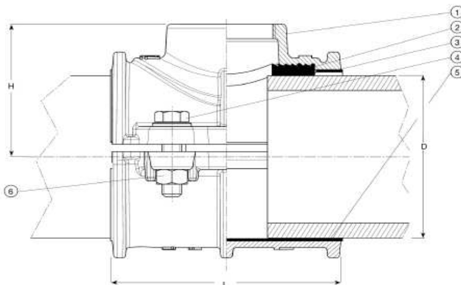
DN 250-300
