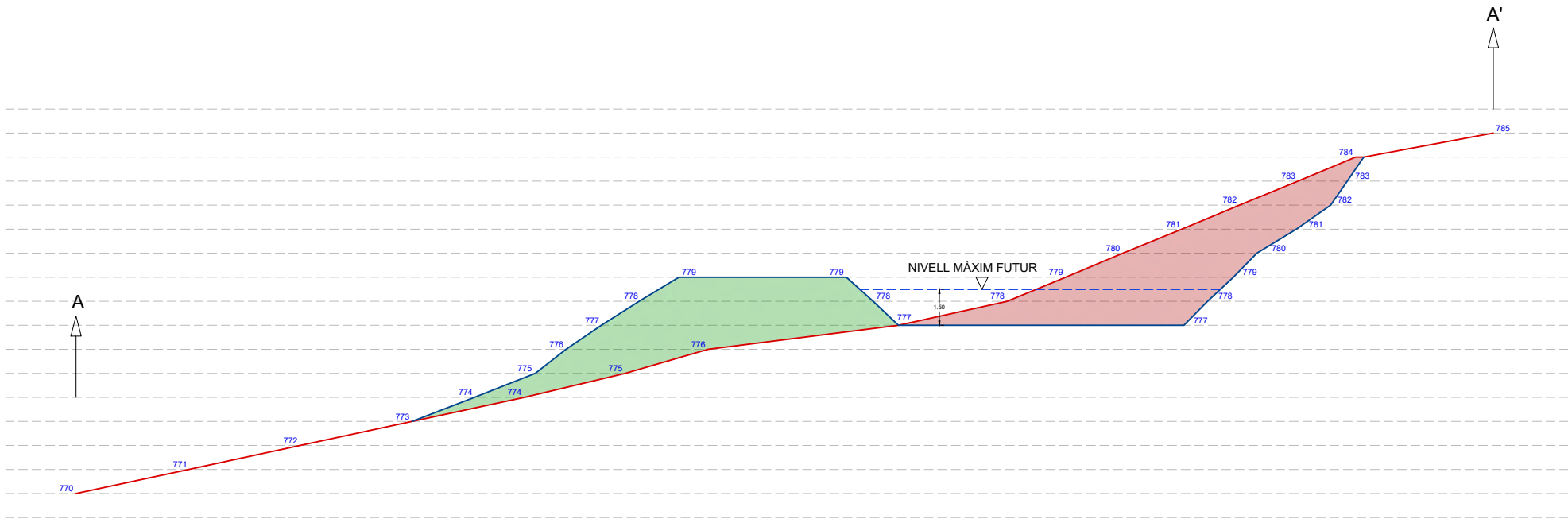
TALL TOPOGRÀFIC A-A' 1:250
