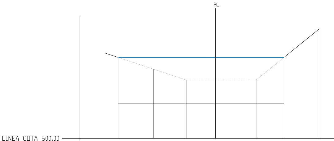
PERFIL TRANSVERSAL 4
