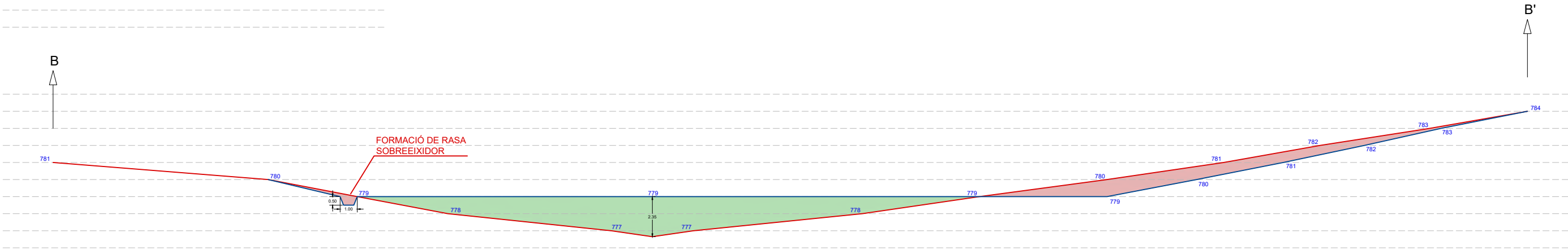
TALL TOPOGRÀFIC B-B' 1:250
