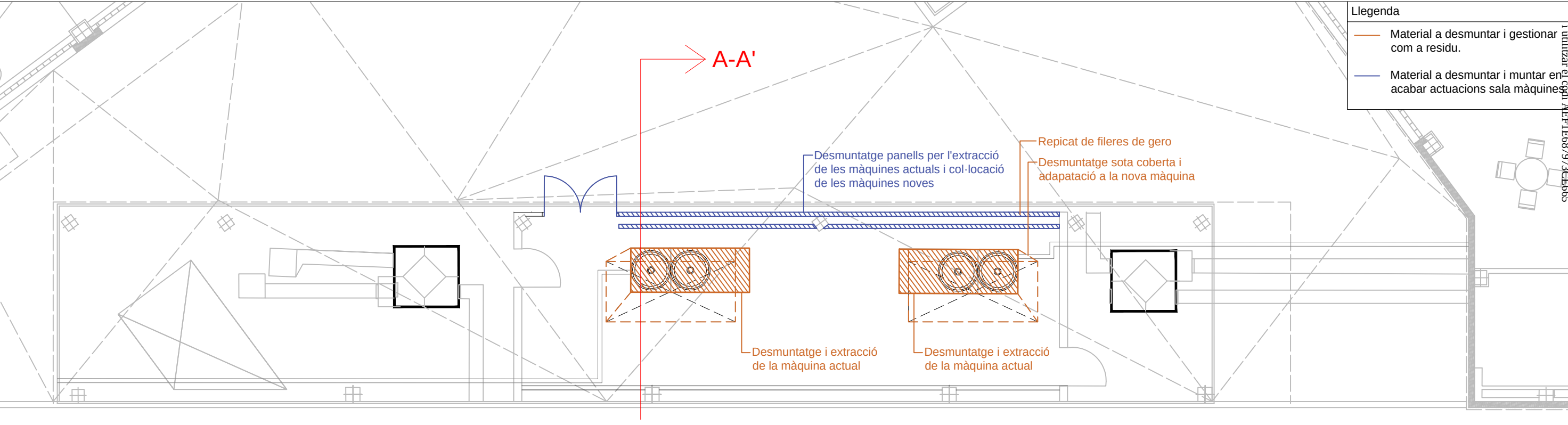
Planta primera - Sala de màquines - Estat actual - Actuacions a realitzar - E: 1/100
