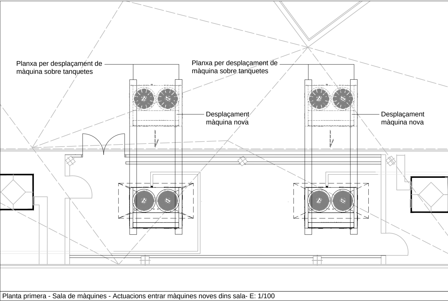
Planta primera - Sala de màquines - Actuacions entrar màquines noves dins sala- E: 1/100
