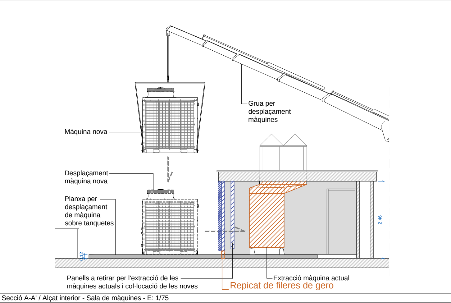
Secció A-A' / Alçat interior - Sala de màquines - E: 1/75
