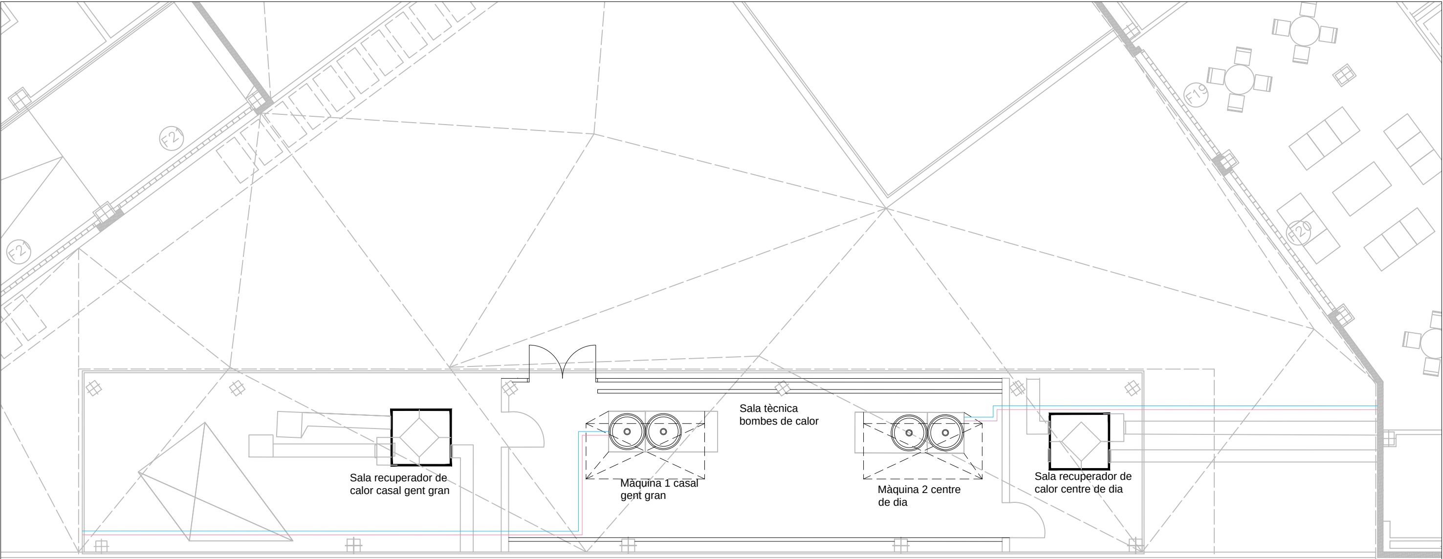
Planta primera - Sala de màquines - E: 1/700
