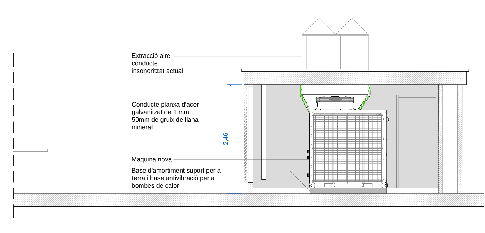
Secció B-B' / Alçat interior - Sala de màquines - E: 1/50
