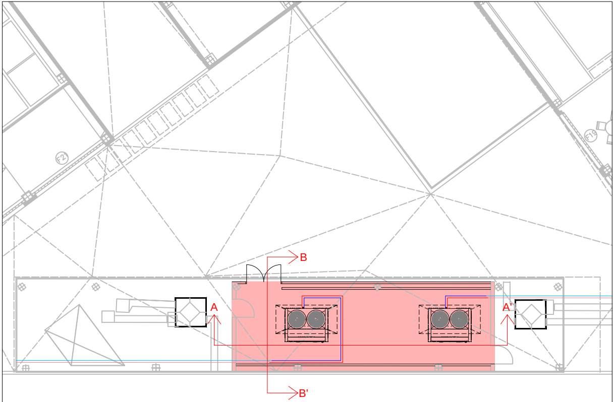
Planta primera - Sala de màquines - E: 1/200
