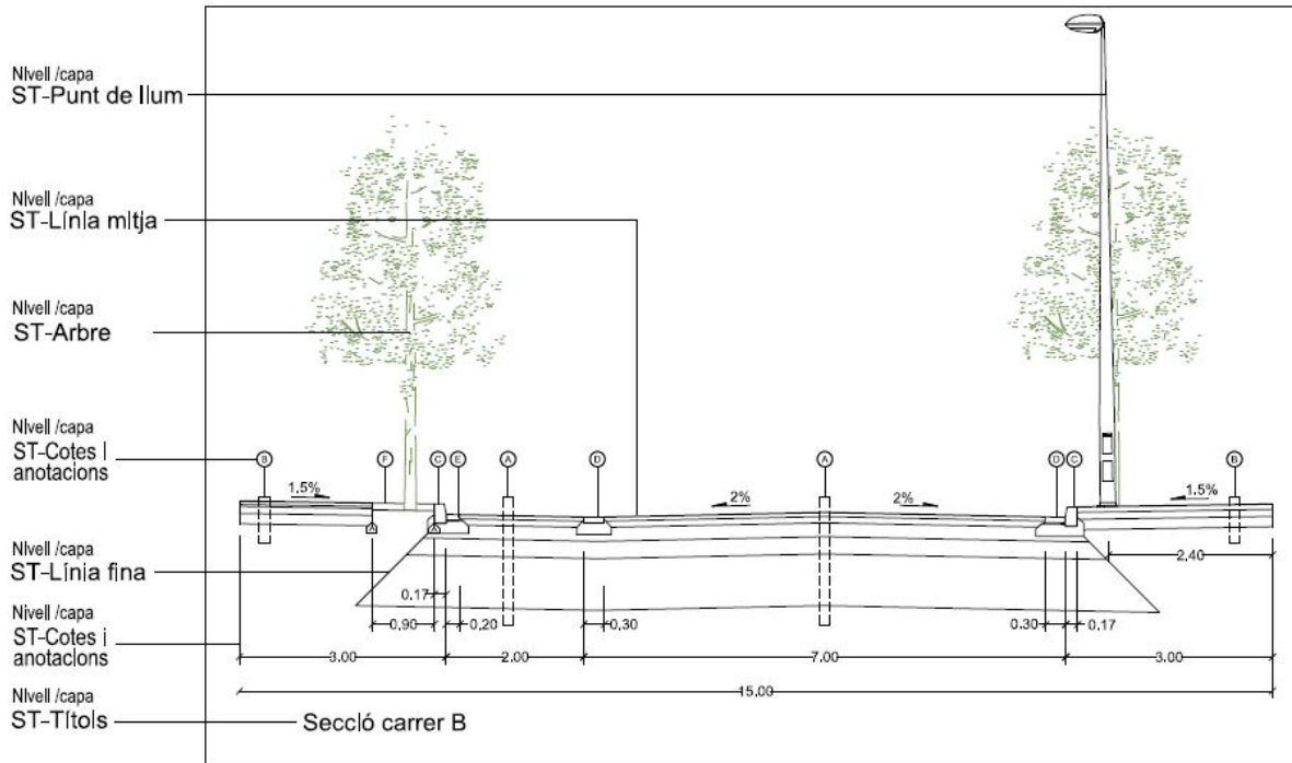
Figura 30. Exemple de llegenda a dibuixar a l'espai model full
