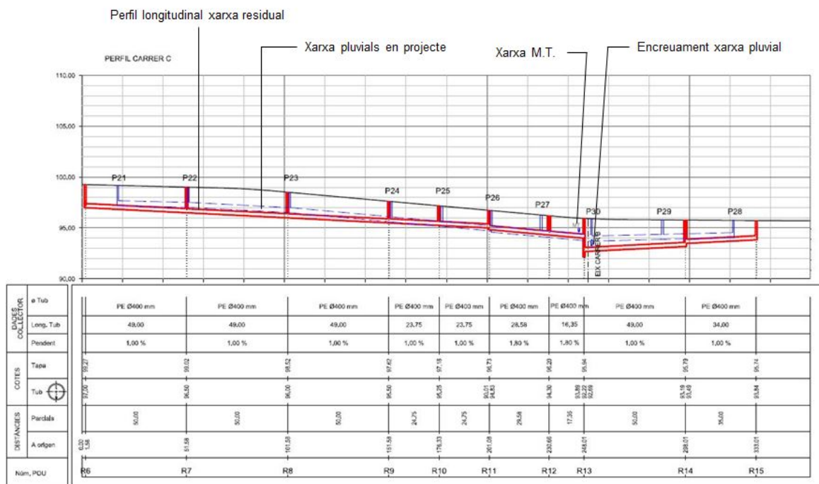
Figura 27. Exemple dels elements a dibuixar a l'espai model de l'arxiu AAAASOOO-12B-Perfils residuals.dgn/dwg
