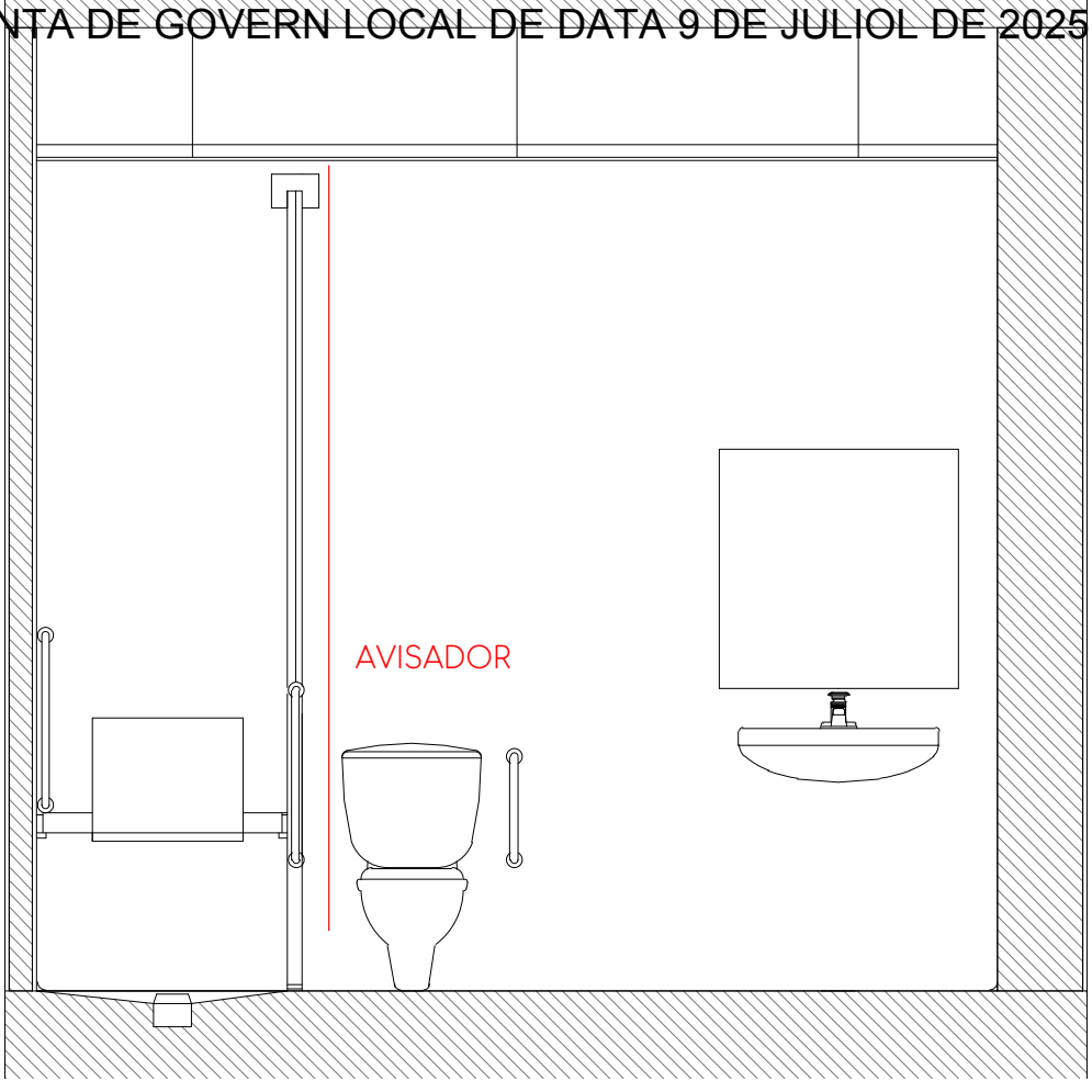
ALÇAT C C'
