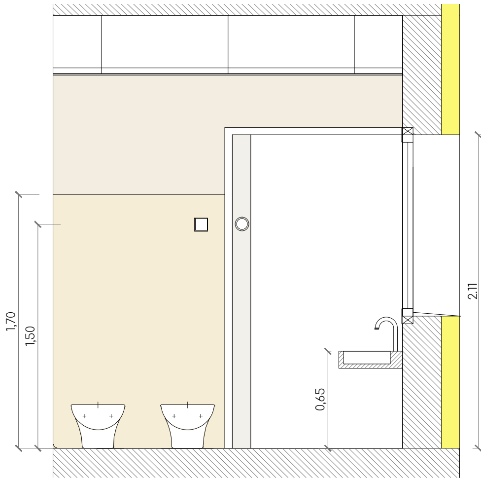
ALÇAT D D'
