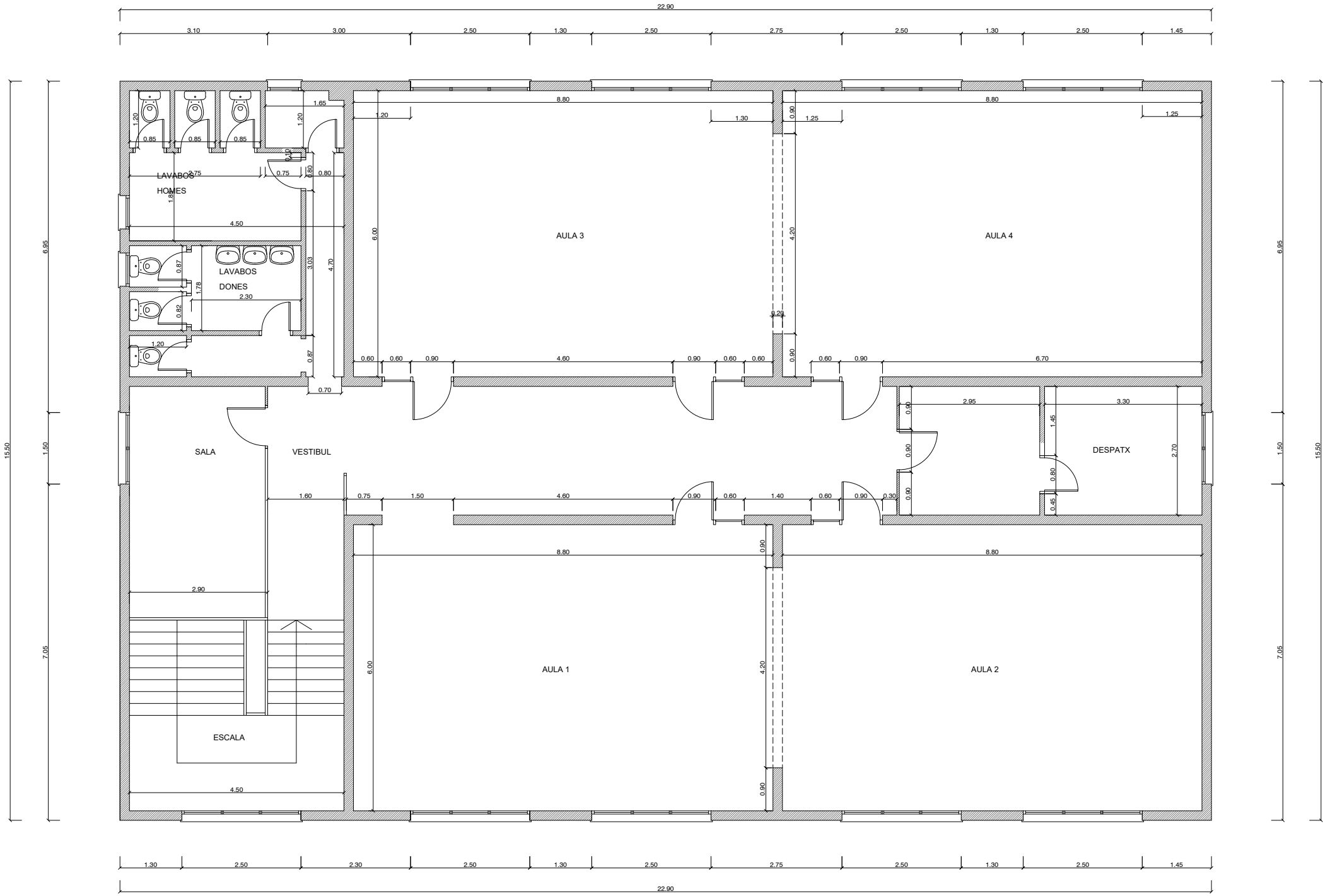
PLANTA PRIMERA
