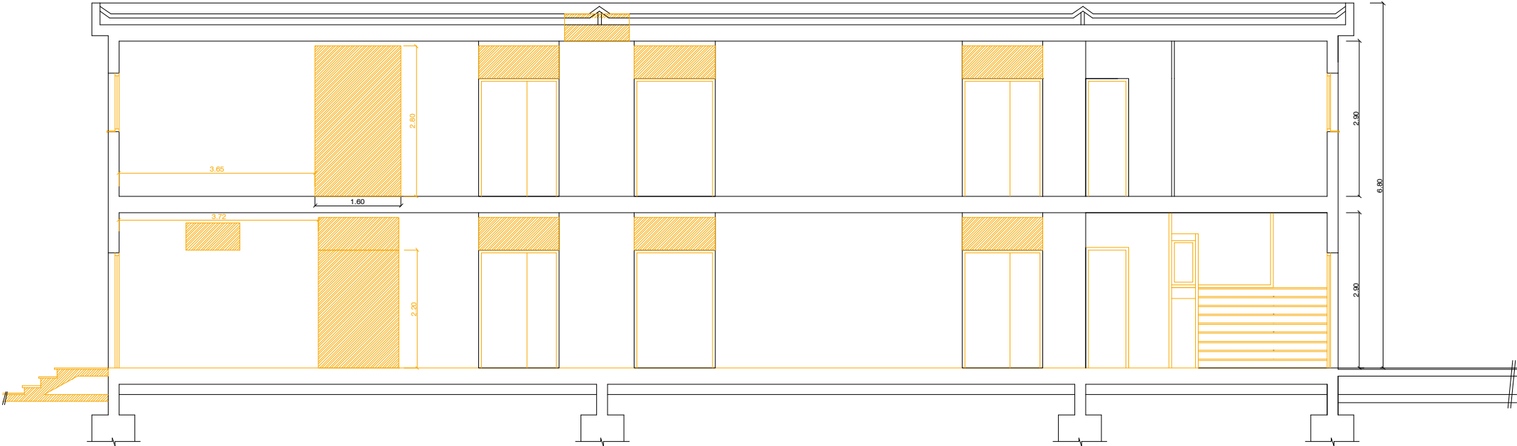
SECCIÓ A-A'
