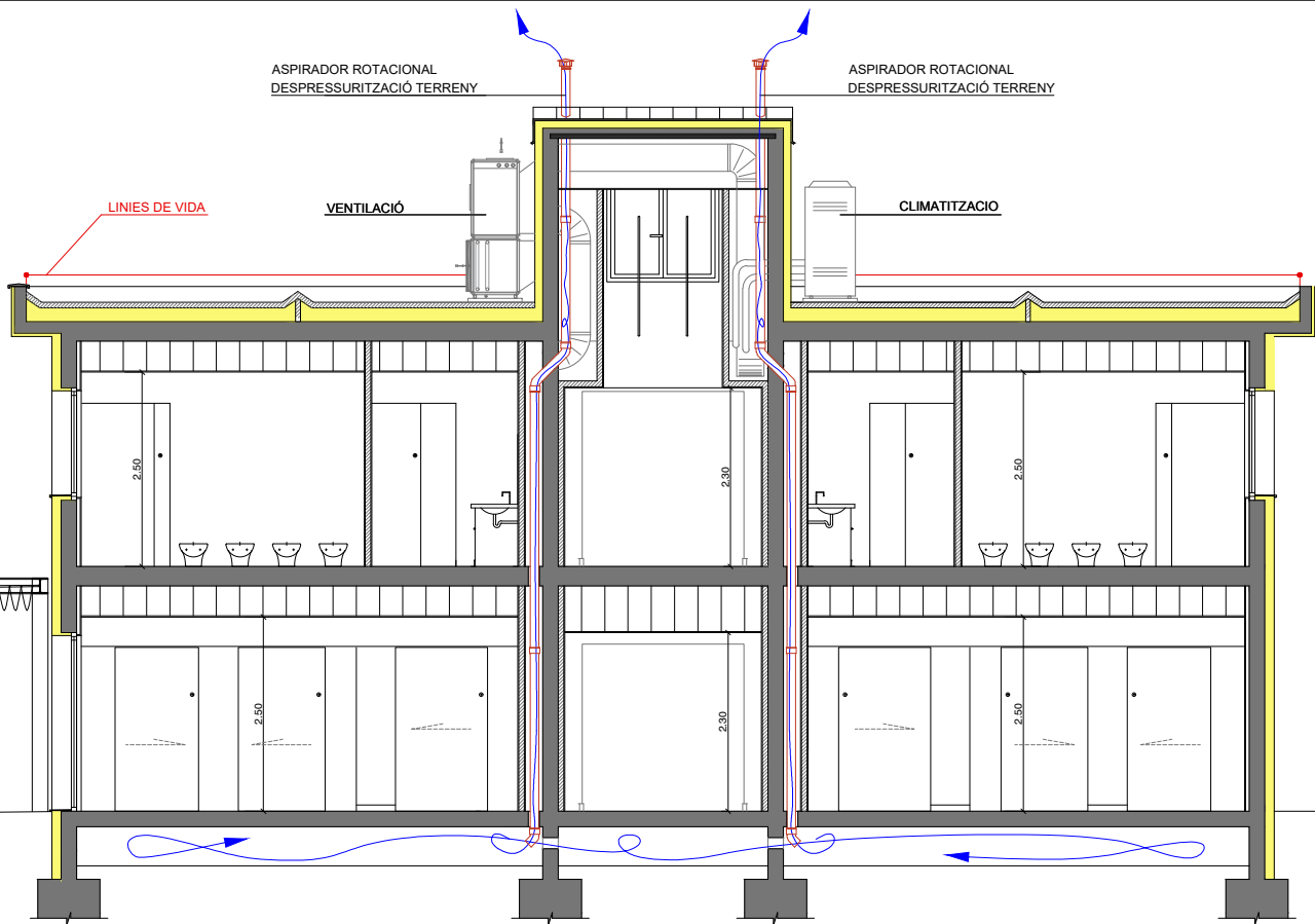
SECCIO F-F'
