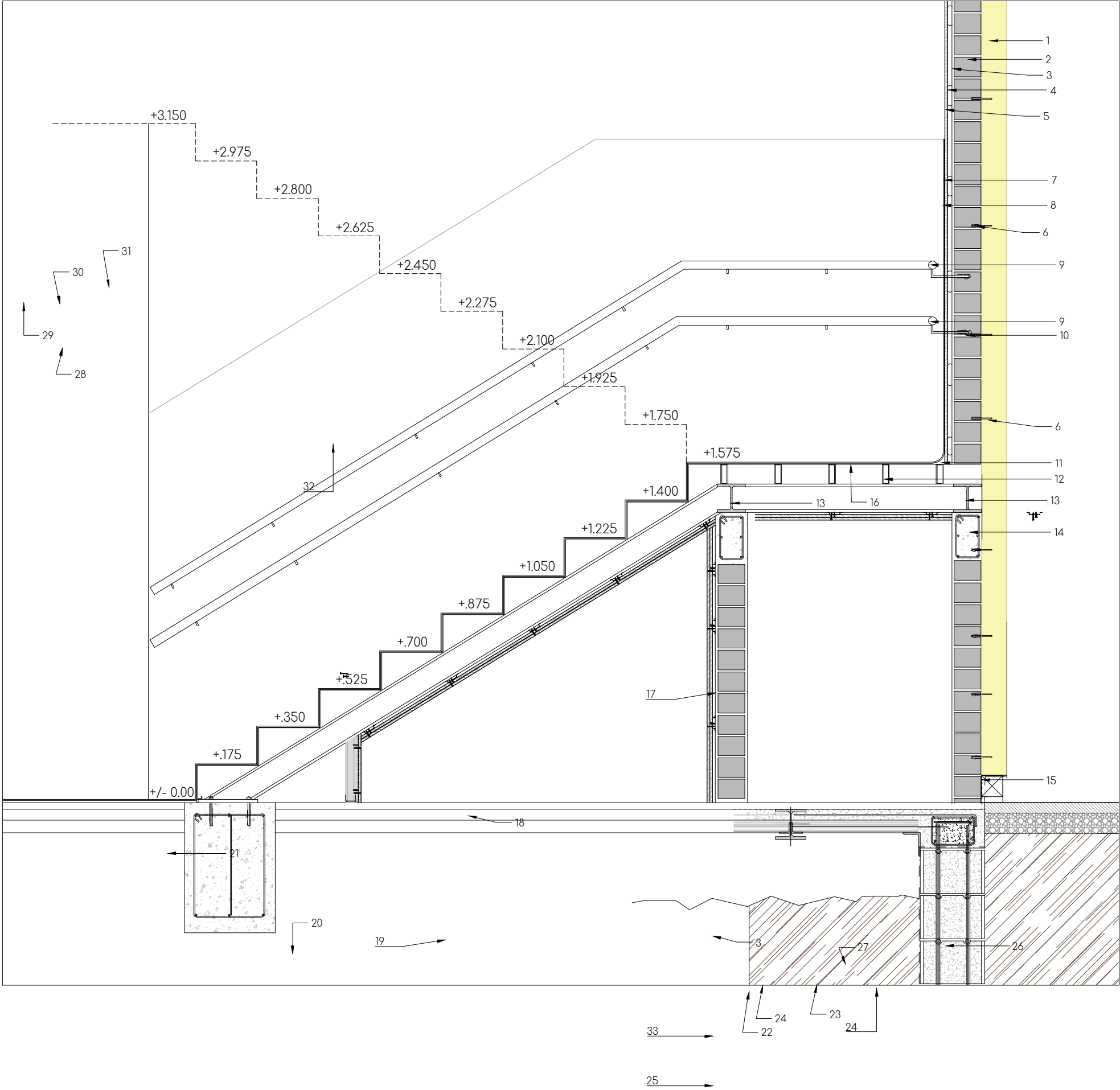
secció escala B-B'
