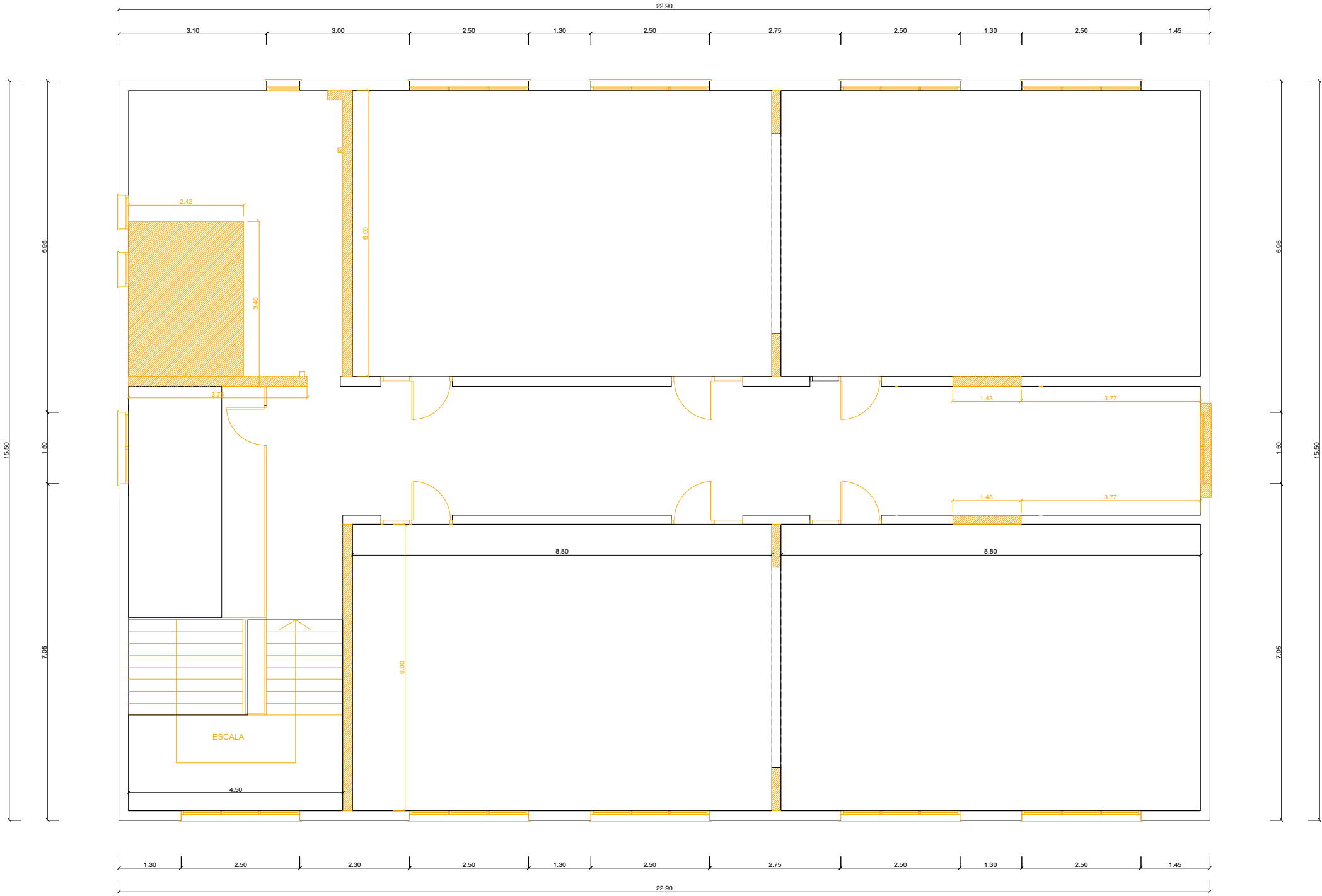
PLANTA PRIMERA
