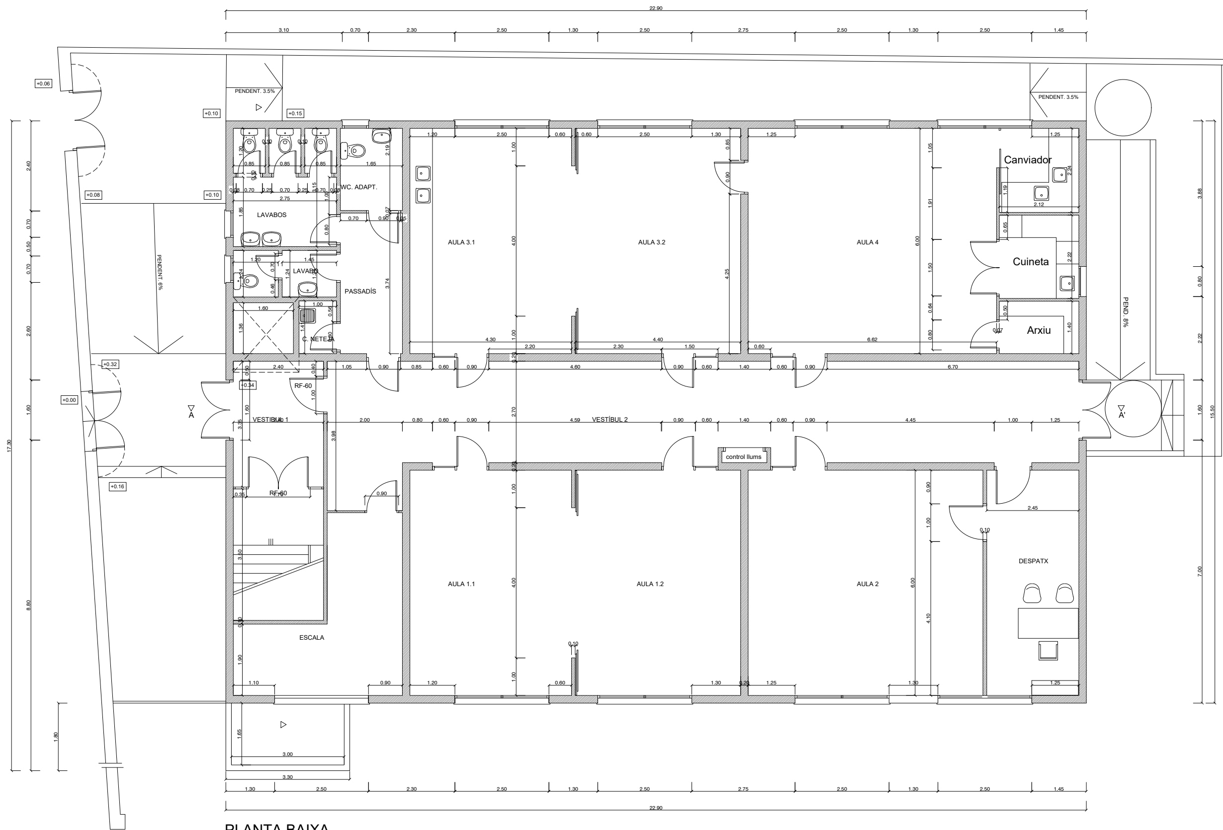
PLANTA BAIXA
