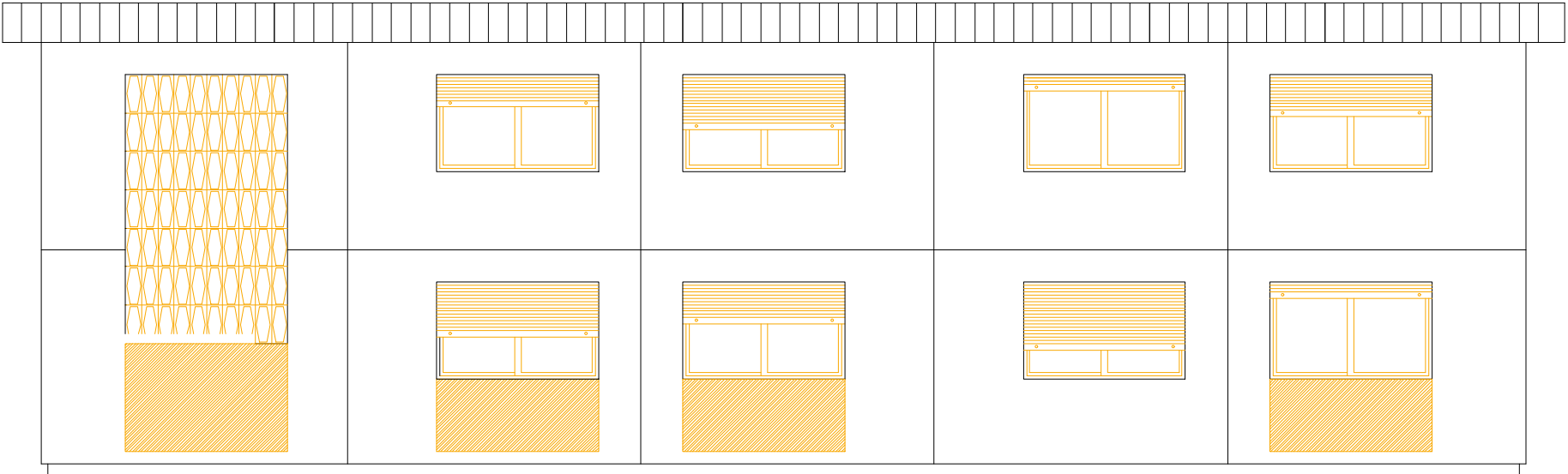
FAÇANA OEST
