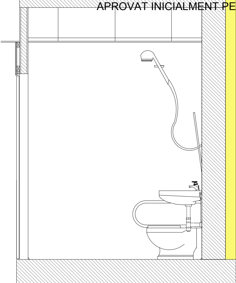
ALÇAT B B'
