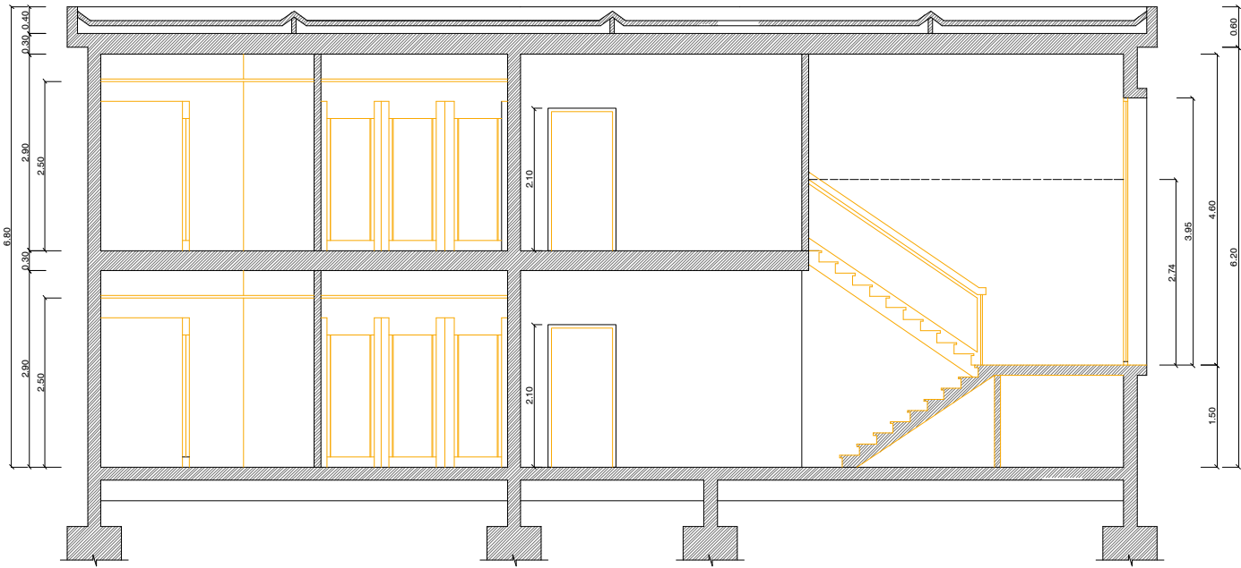
SECCIÓ B-B'
