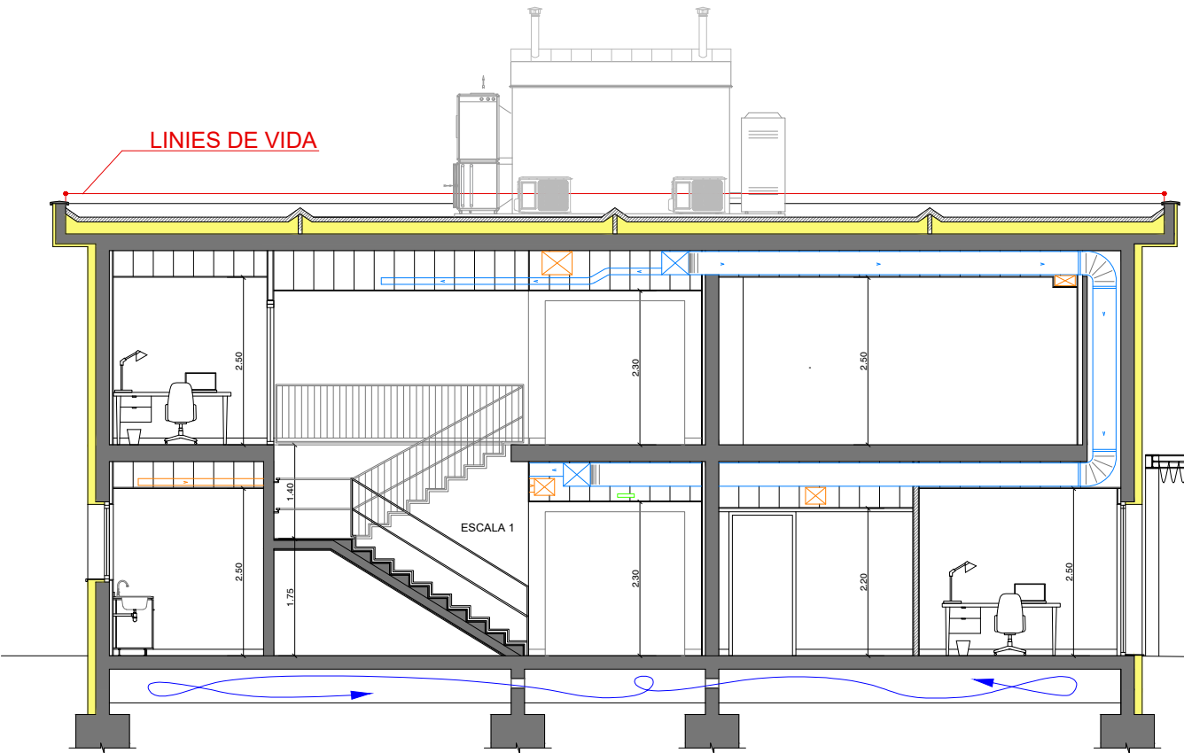
SECCIO A-A'
