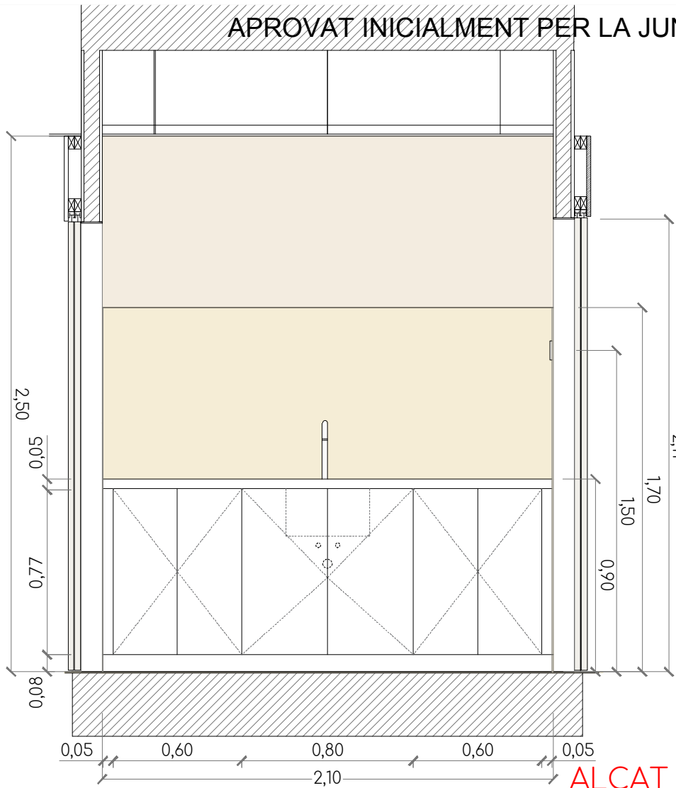
ALÇAT A A'
