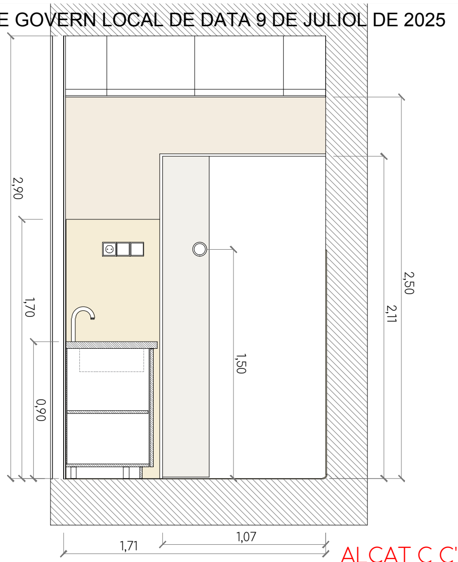
ALÇAT B B'
