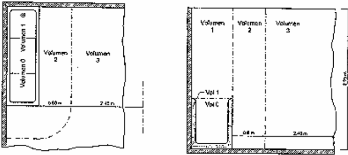
Figura 2 – BAÑERA CON PARED FIJA
