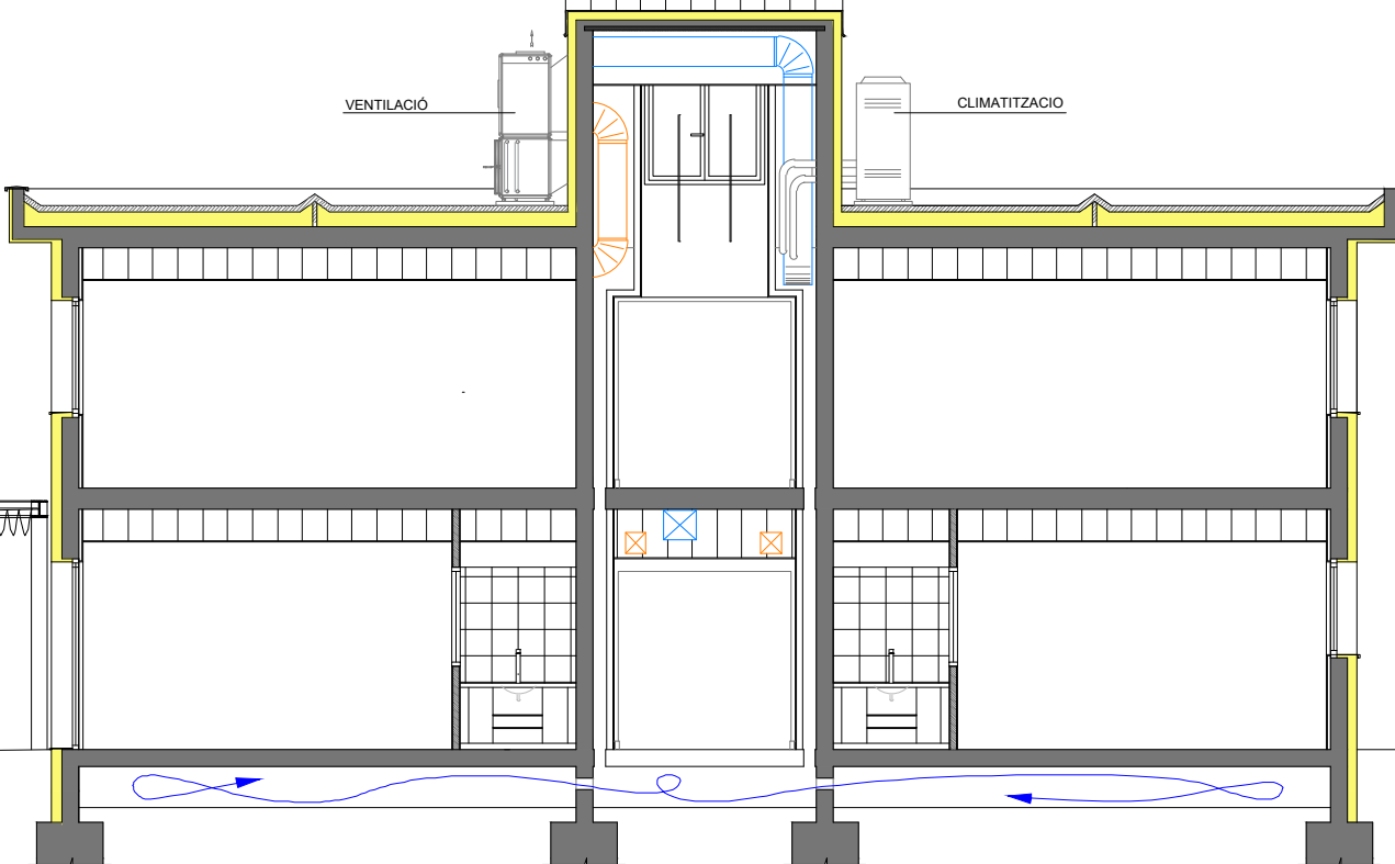
SECCIO F-F'
