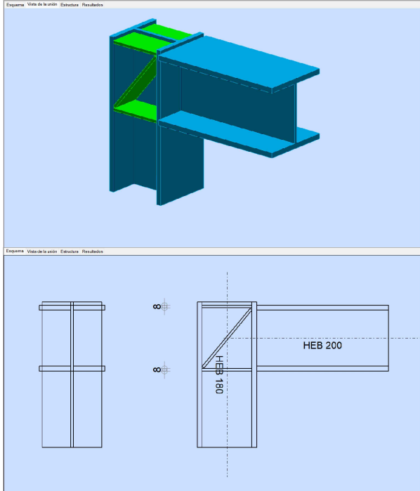
Pilar-jàssera HEB 180 - HEB 200
