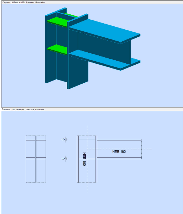
Pilar-jàssera HEB 180 - HEB 180
