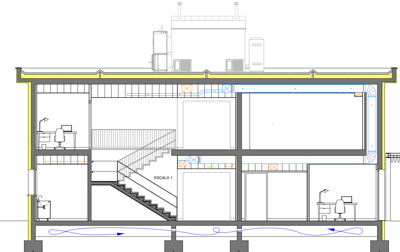
SECCIO A-A'
