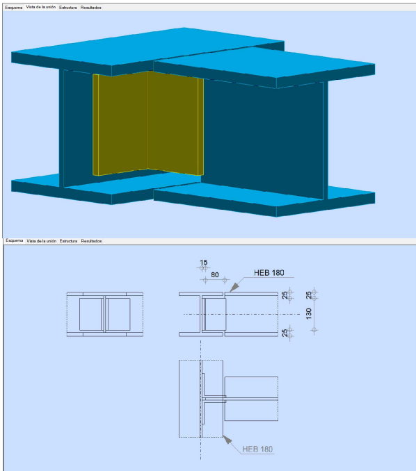
Jou bigues HEB 180
