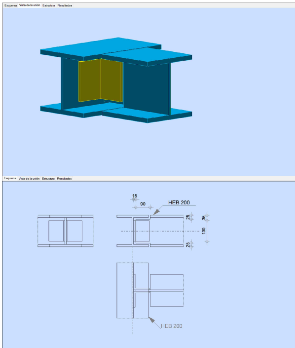
Jou bigues HEB 200
