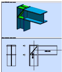
Pilar-jàssera HEB 180 - HEB 200
