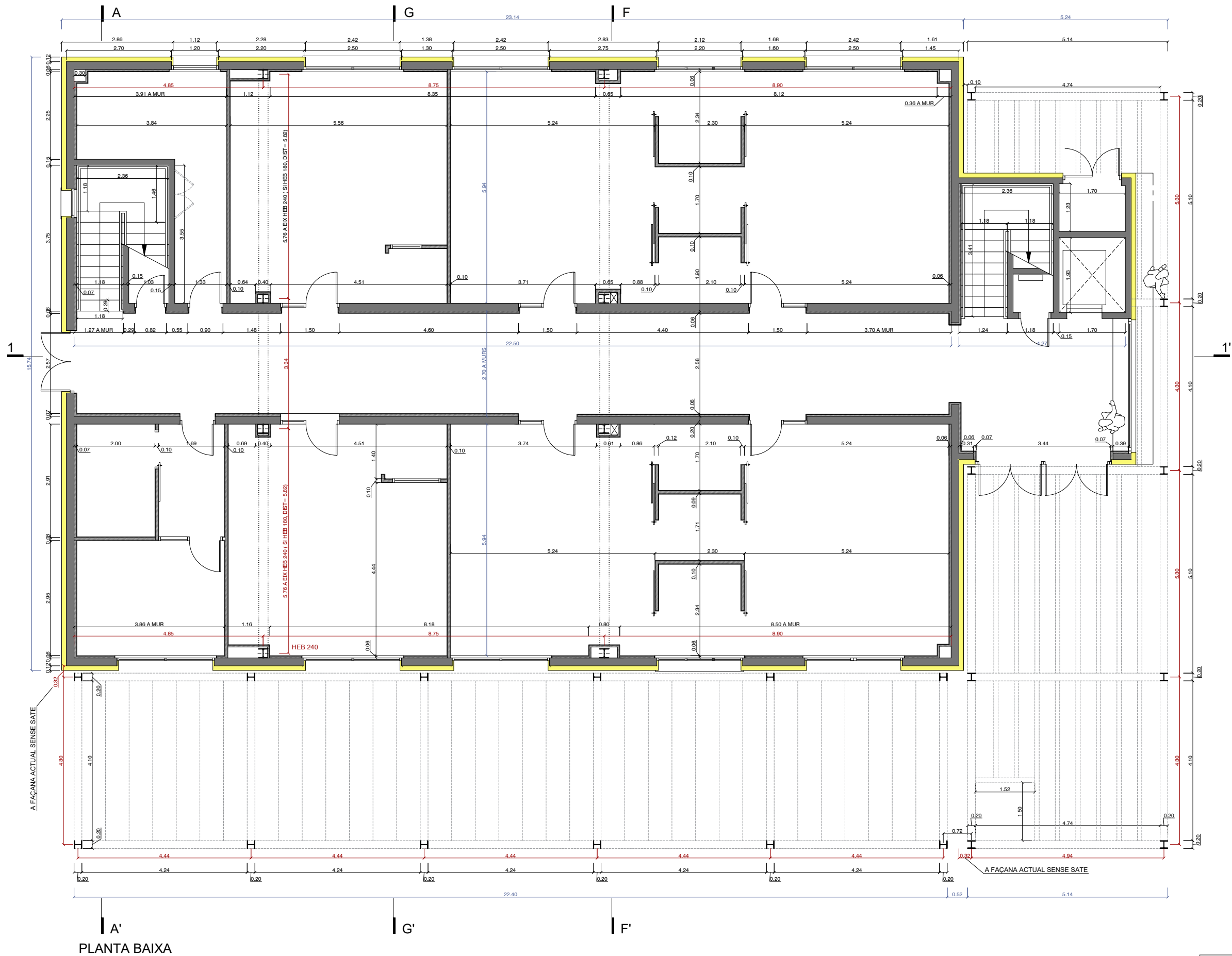
PLANTA BAIXA
