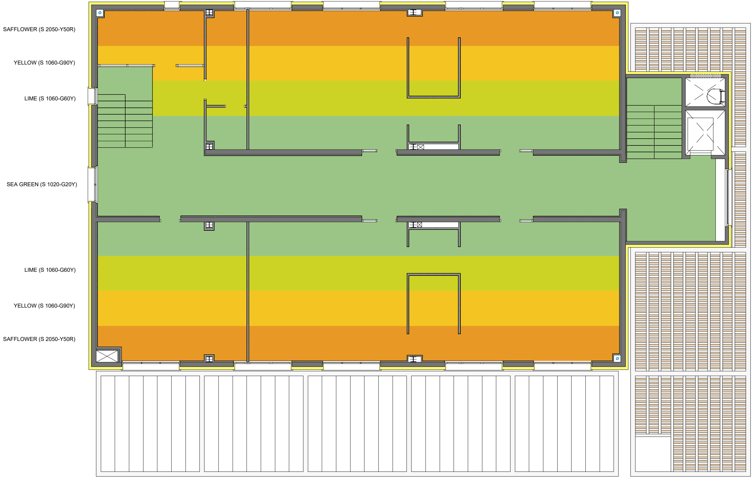
PLANTA PRIMERA
