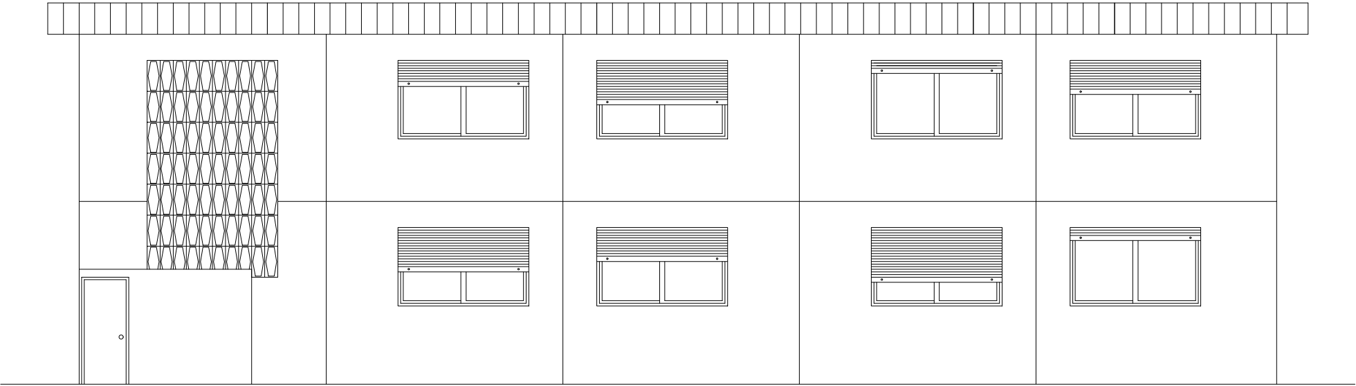
FAÇANA OEST
