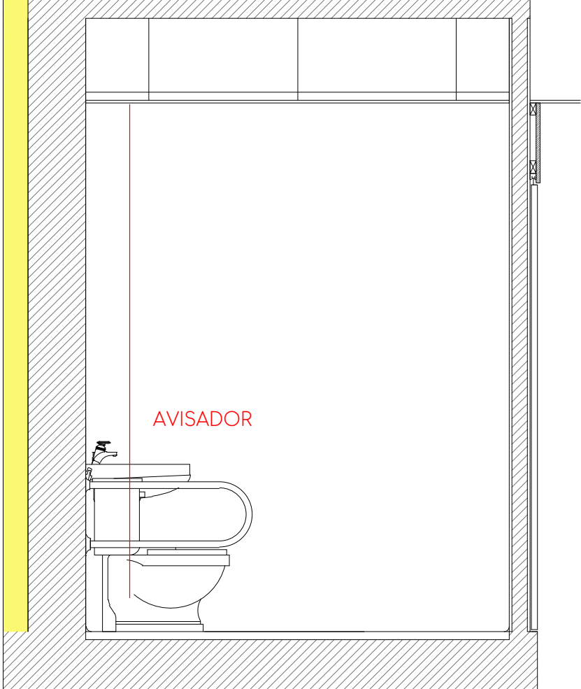
ALÇAT A A'
