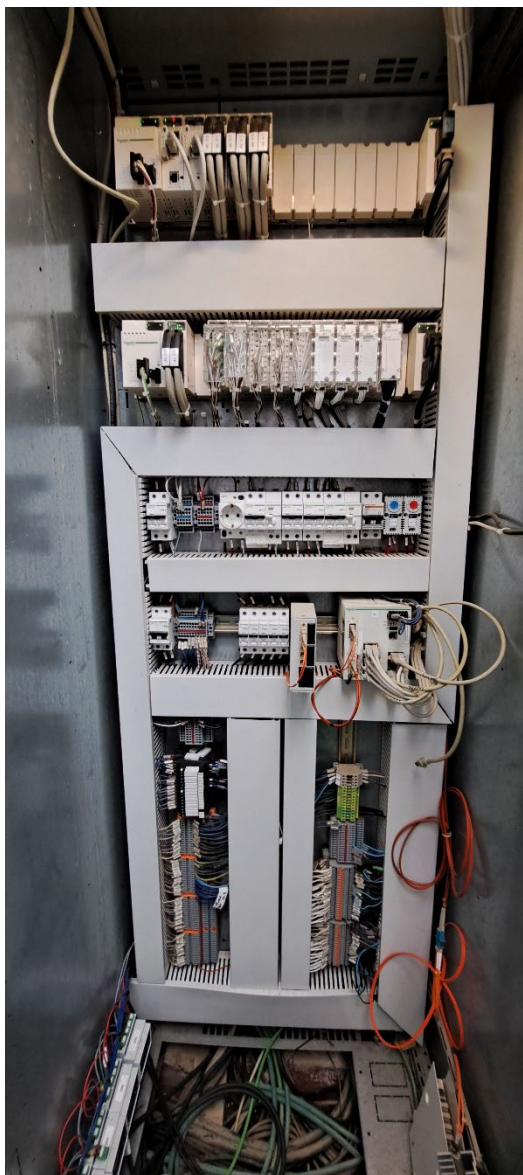
Foto Núm 7: Vista interior del CCM2 on passar els cables de senyals i Ethernet
