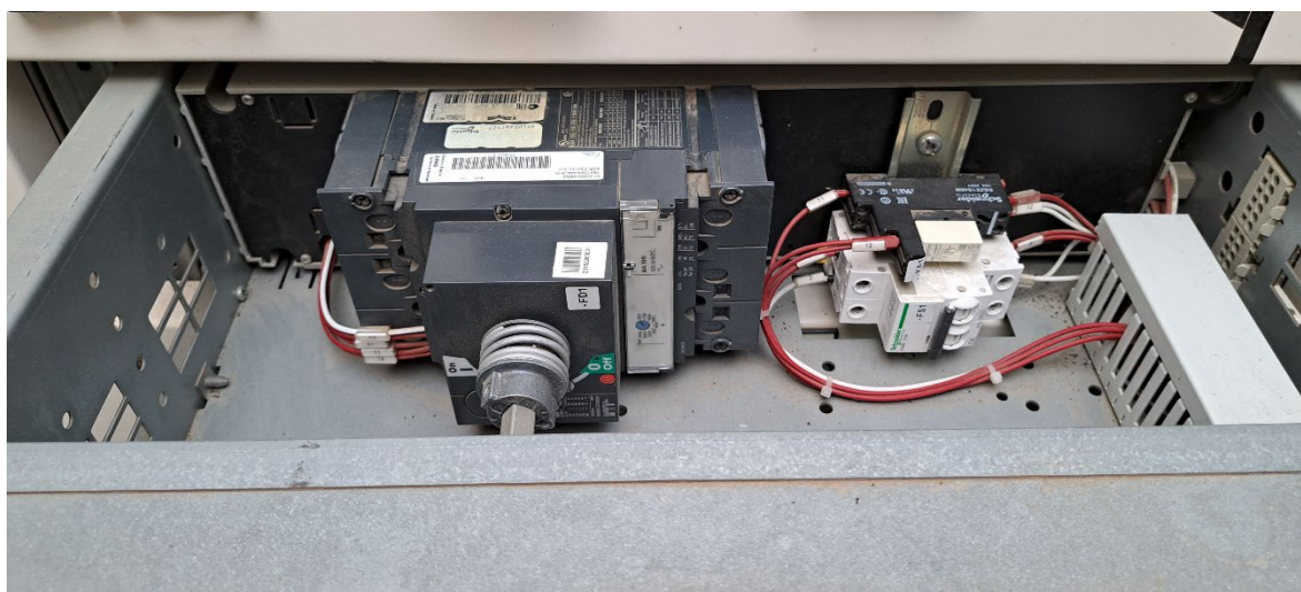
Foto Núm 6: Vista interna del cubicle a modificar.
