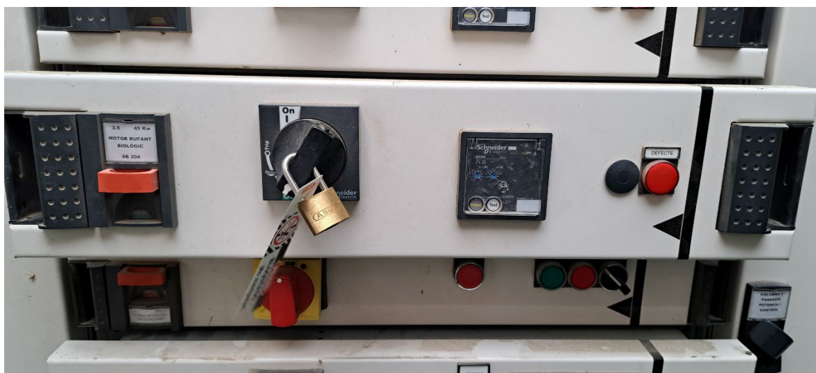
Foto Núm 5: Vista del cubicle a modificar.
