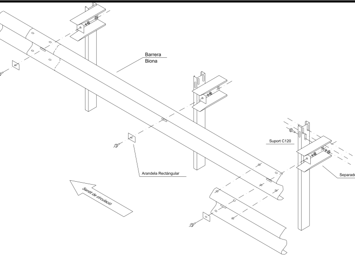
BARRERA METÀL·LICA DE SEGURETAT AMB PERFIL DE DOBLE ONA BMSNA2/C MUNTATGE DE LA BARRERA
