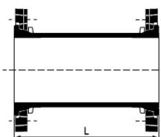
DN 60 a 400 *Bridas orientables
