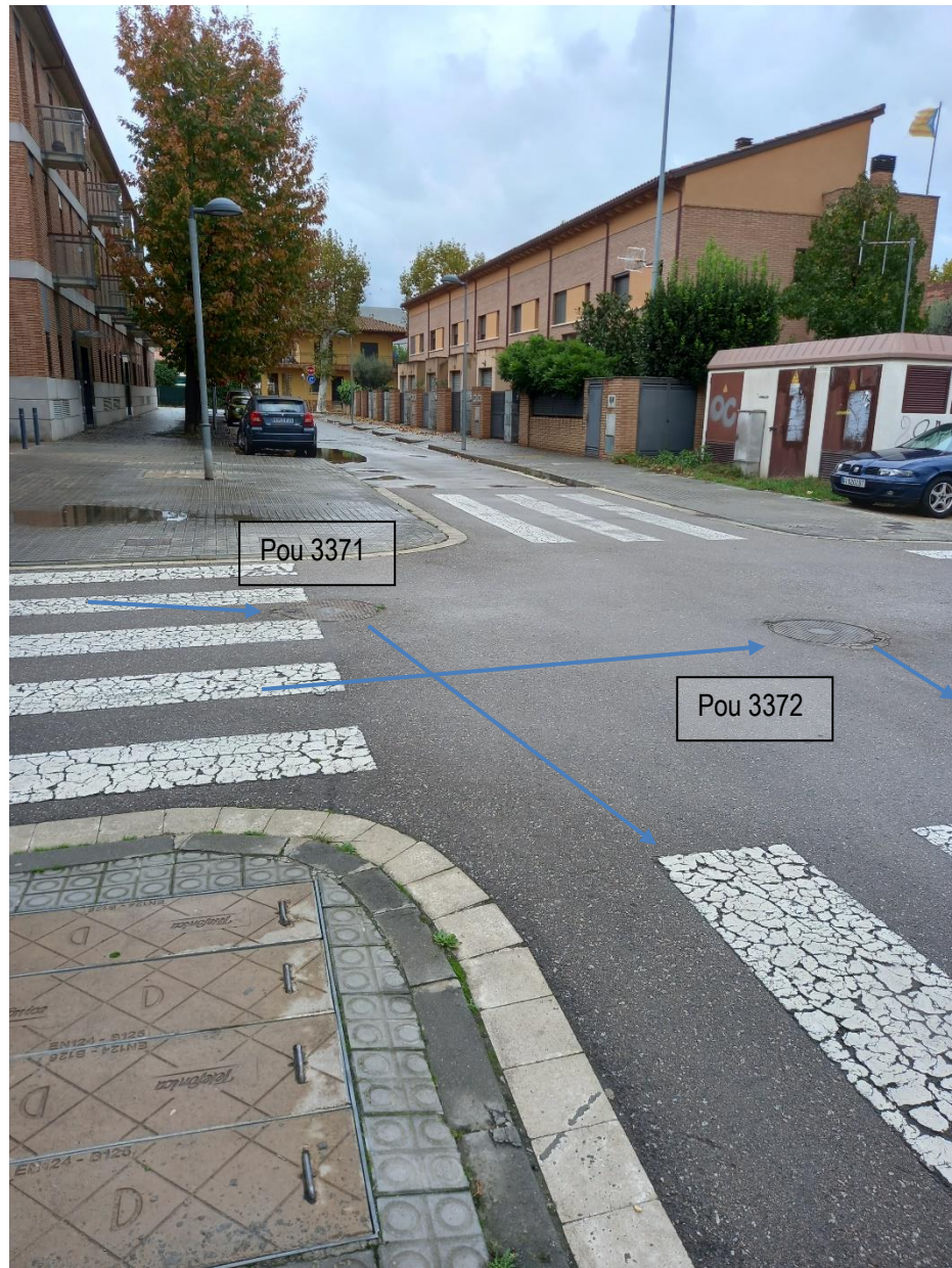
Fotografia 3: Vista cruïlla carrer Lluís Companys amb carrer Can Pàmies, pous 3372 i 3371. Punt on la línia pluvial creua per sota la línia residual on s'ha d'actuar
