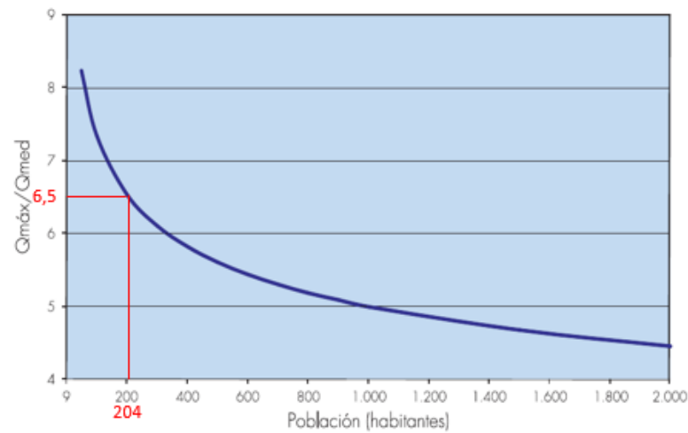
Figura 1.3. Relación entre Q_{max}/Q_{med} y el número de habitantes
