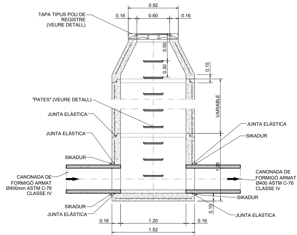
SECCIÓ B-B ESCALA 1/40
