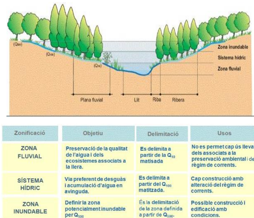
Figura 2. Zonificació de l'espai fluvial
