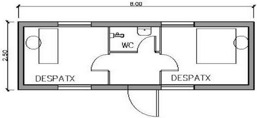
Planta oficines
