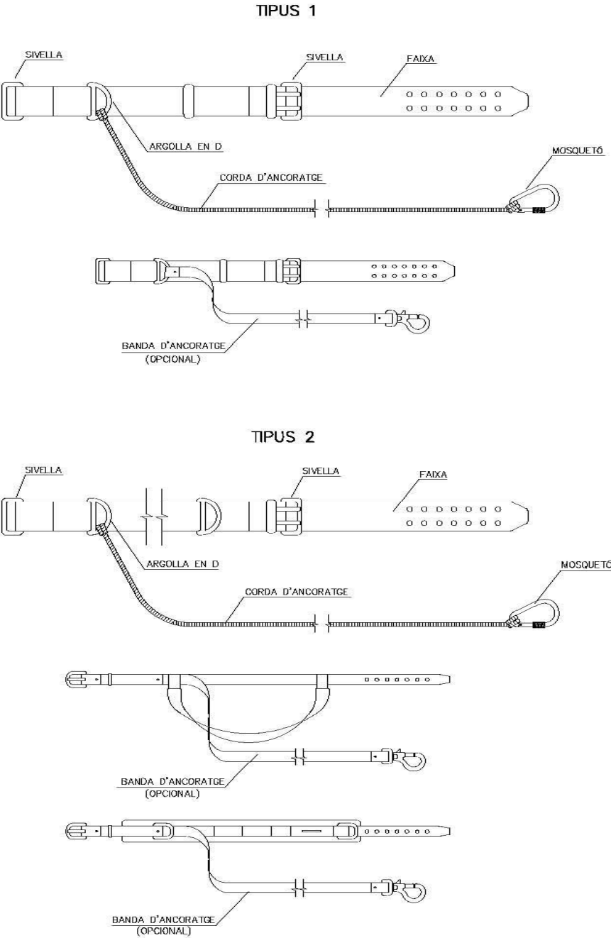
Corretges d'ancoratges
