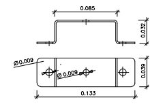
Fabricat en planxa de ferro galvanitzada en calent de 2 mm. d'espessor
