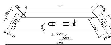
Detall constructiu. Peca d'ancoratge senyal triangular
