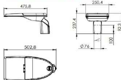
Fijación vertical \varnothing 76 mm (PT1)
