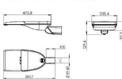
Fijación lateral \varnothing 49/60 mm (SE2)
