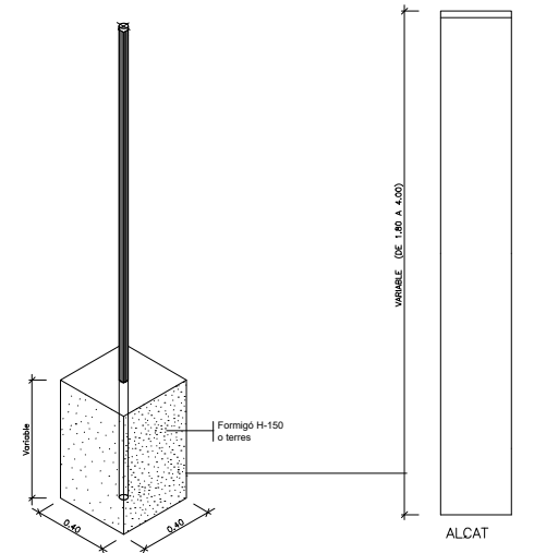
AXONOMÈTRICA
