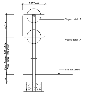
Detall constructiu. Senyal quadrada
