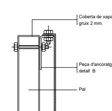
Subjecció amb clau
