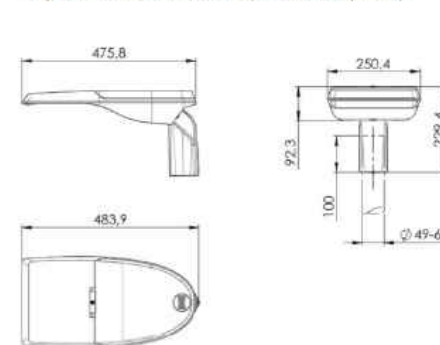
Fijación vertical \varnothing 49/60 mm (PT2)
