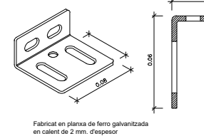
Fabricat en planxa de ferro galvanitzada en calent de 2 mm. d'espessor
