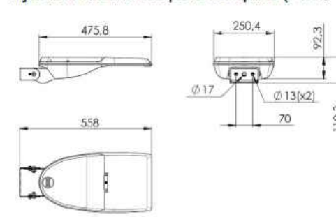
Fijación mural. Incorpora horquilla (FM1)
