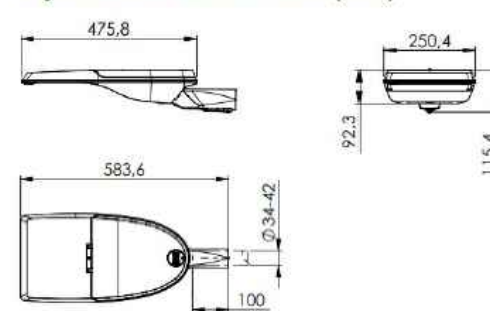
Fijación lateral \varnothing 34/42 mm (SE1)
