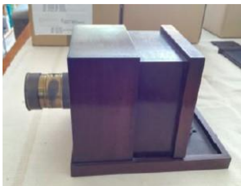
Fig 1. (esquerra) Càmera de daguerrotípia de calaix lliscant. Format mitja placa amb objectiu per a retrat amb tapa.
