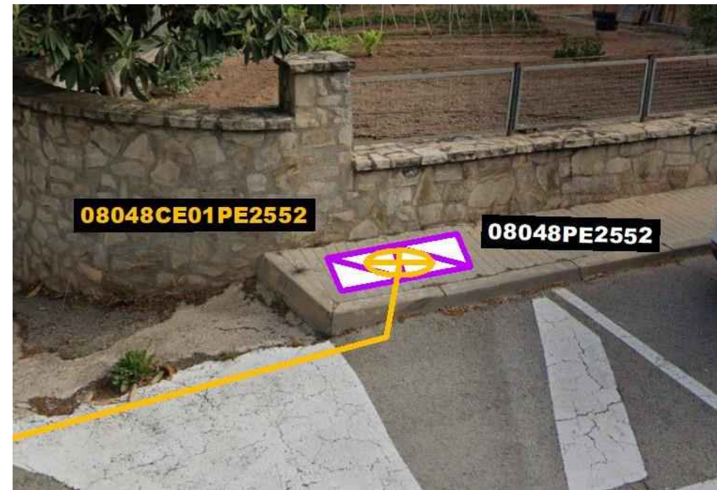
Fig 5: Ubicació caixa d'empalmament 08048CE01PE2552 en pericó 08048PE2552
