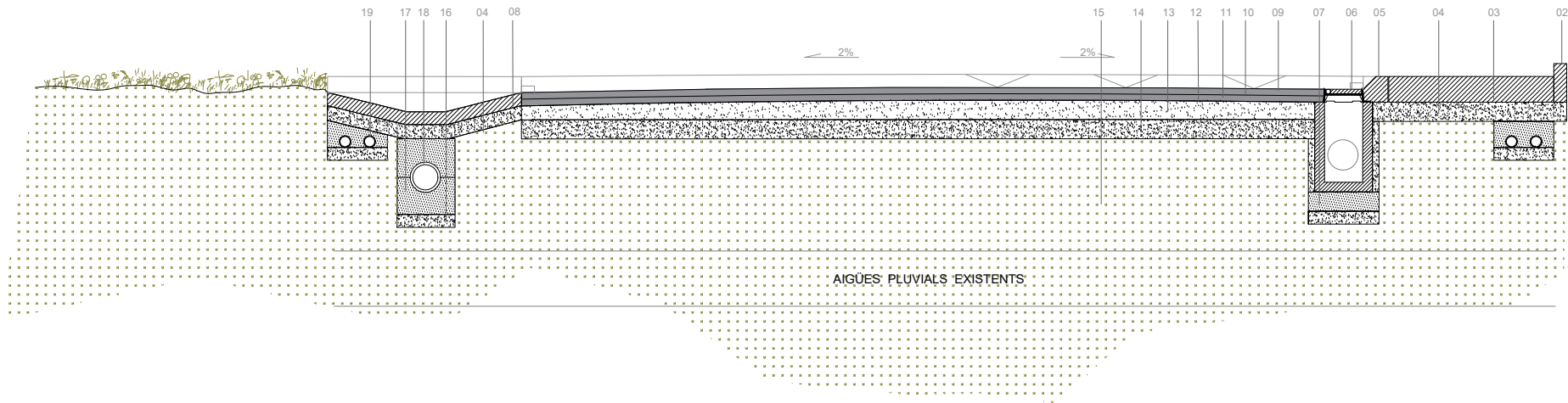
Secció C-C'
