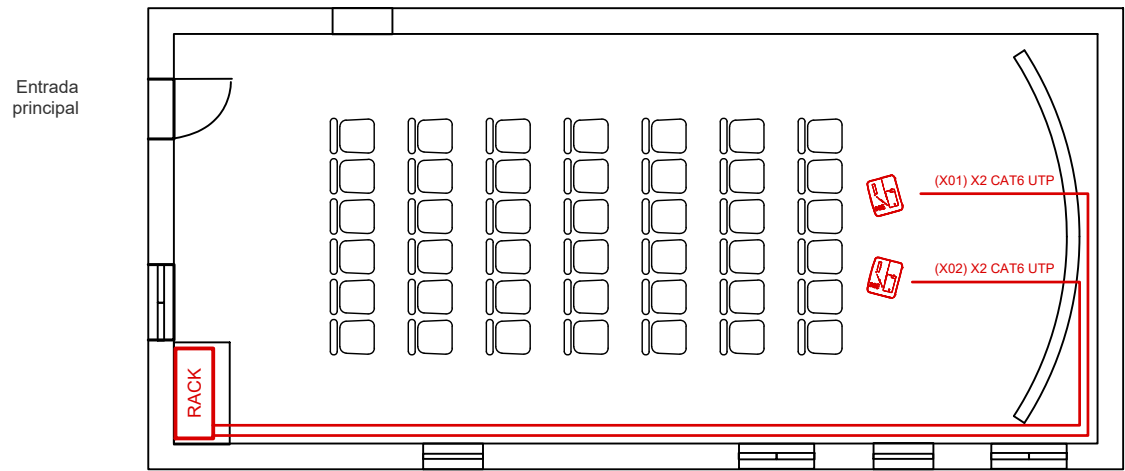
INSTAL.LACIÓ XARXA
