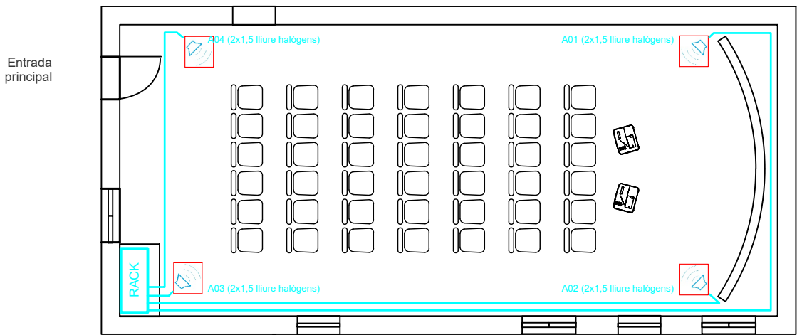
INSTAL.LACIÓ ENLLUMENAT
