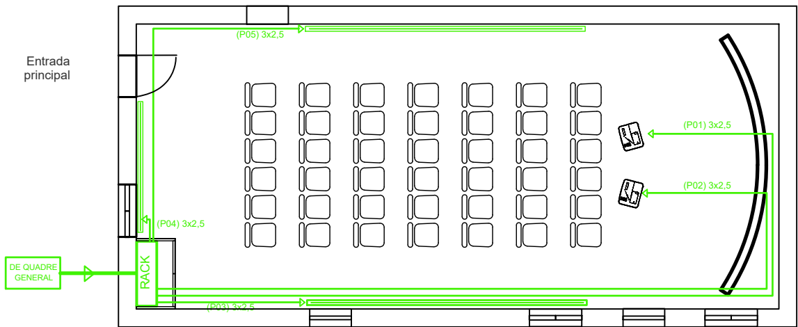
INSTAL.LACIÓ XARXA
