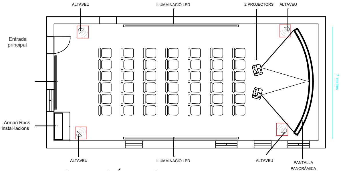
INSTAL.LACIÓ AUDIO
