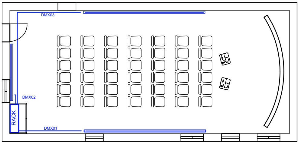
INSTAL.LACIÓ DMX
