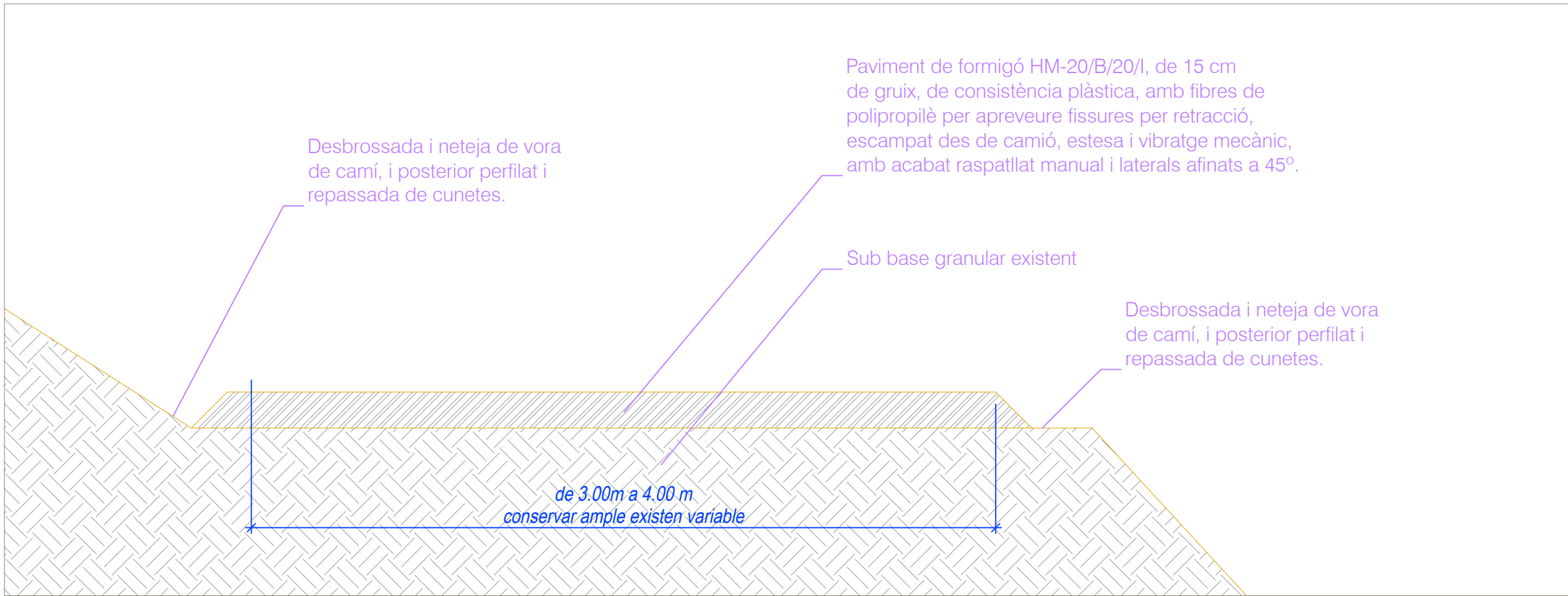
CAMÍ DEL RIU DETALL SECCIÓ FERM | E:1/1500
