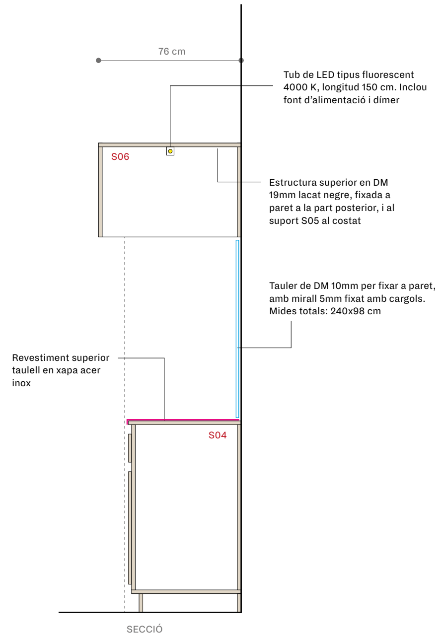
SECCIÓ
