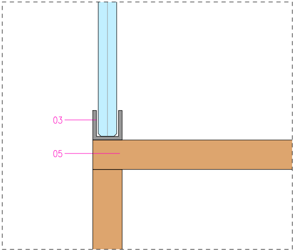
DETALL SECCIÓ VERTICAL - ESC. 1:2
