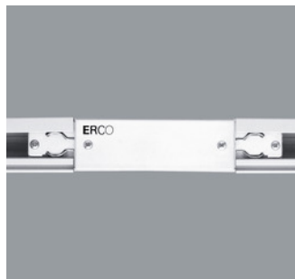
79304.000 Acoplamiento trifásico Material sintético. Alimentación posible. Cableado continuo. Blanco
