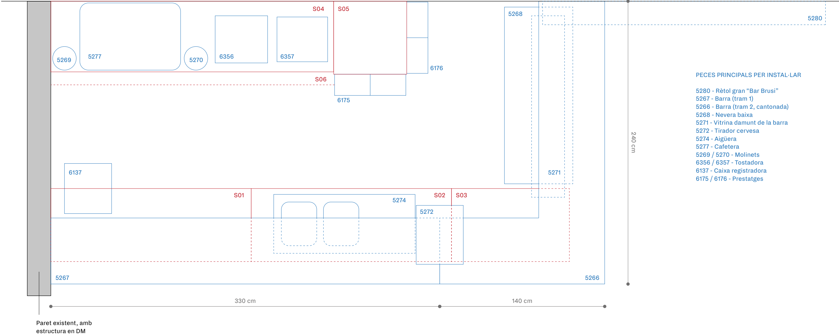
PLANTA DISPOSICIÓ PECES - ESC. 1:20
