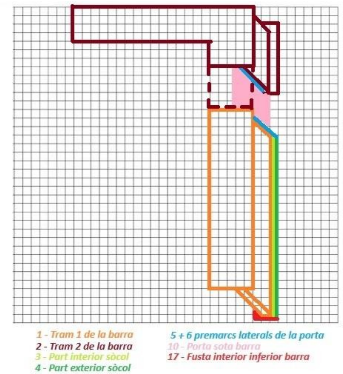
10.6 Croquis amb identificació de peces de la barra:
