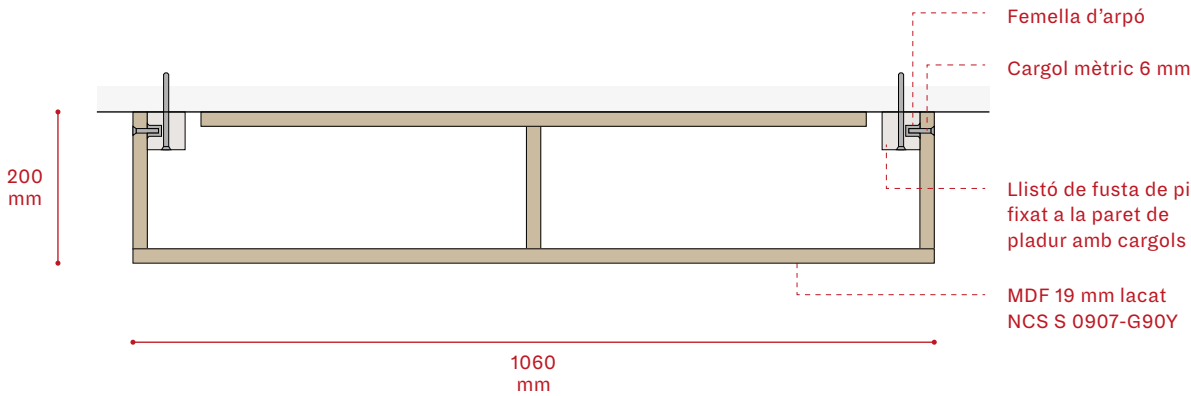
DETALL SECCIÓ HORIZONTAL BASE - ESC. 1:10
