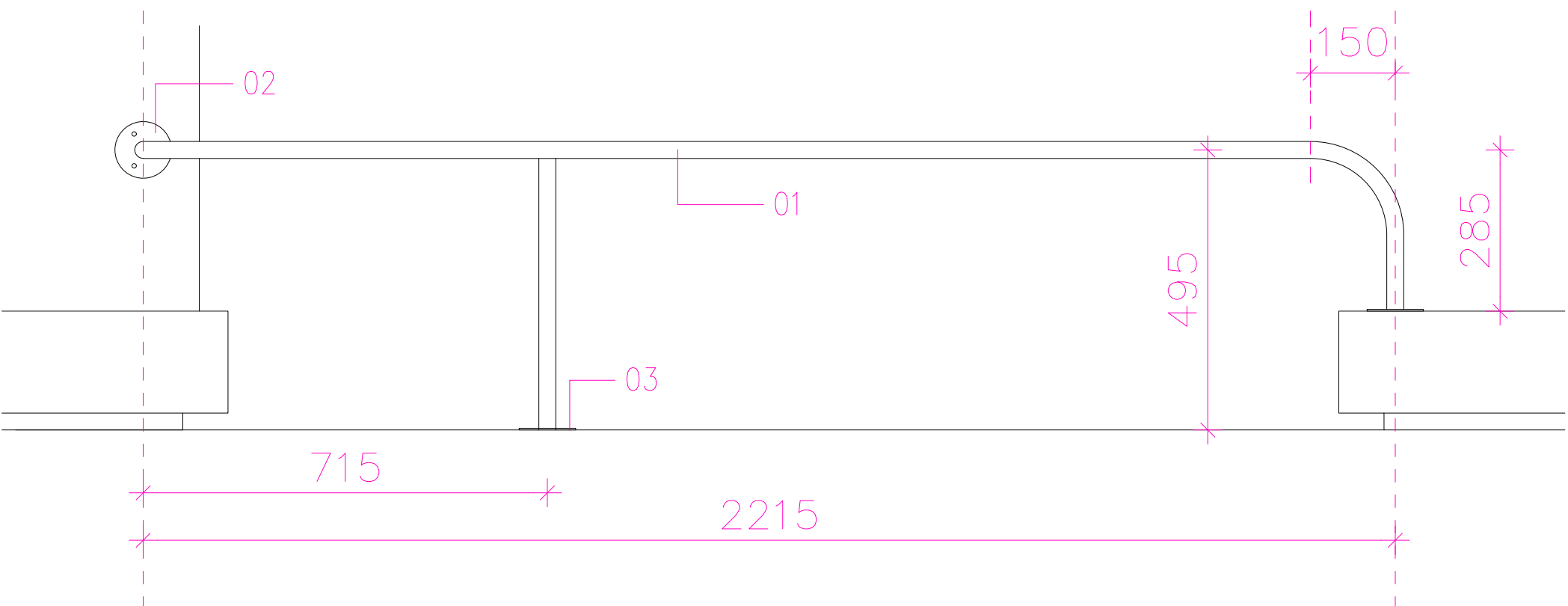
ALÇAT FRONTAL
