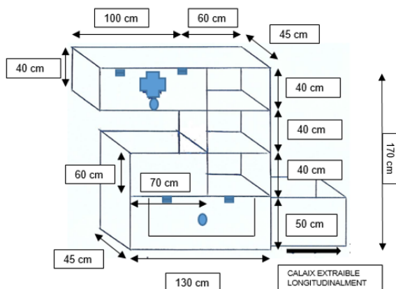
MOBLE LATERAL DRET INTERIOR FURGONETA
