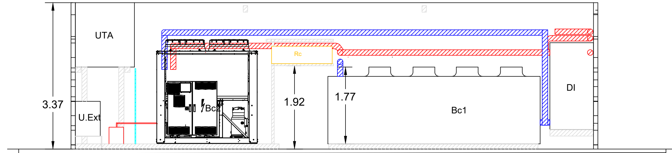
SECCIÓ SALA DE MÀQUINES
