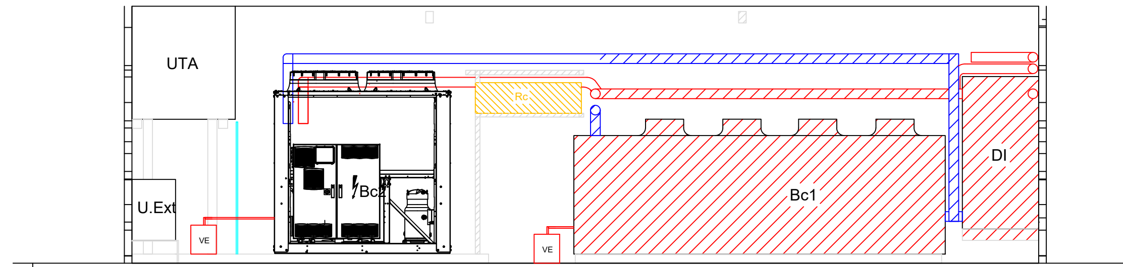
SECCIÓ SALA DE MÀQUINES
