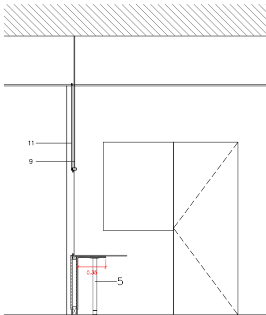
SECCIÓ 2
