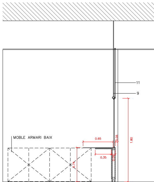
SECCIÓ 1
