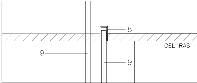
DETALL B
