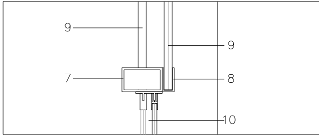
DETALL C
