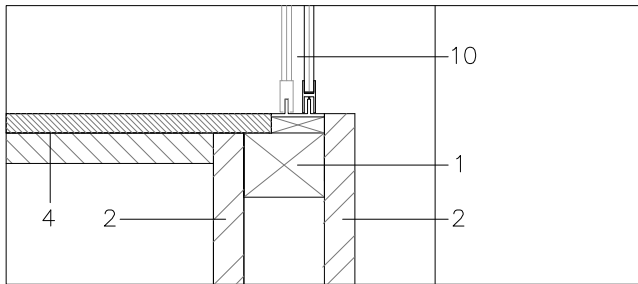
DETALL D
