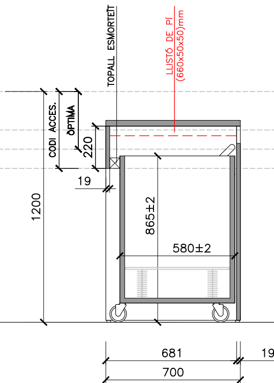
SECCIÓ 1
