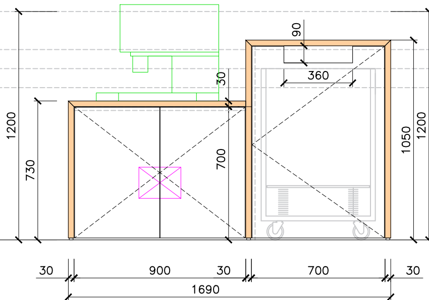
ALÇAT FRONTAL
