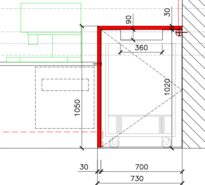
ALÇAT FRONTAL
