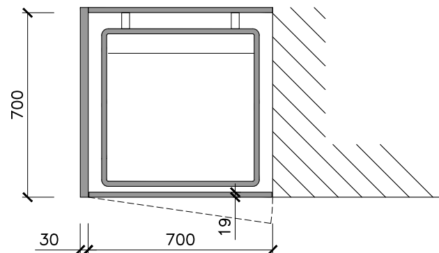
PLANTA SECCIONADA
