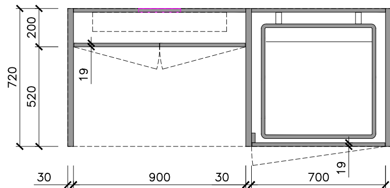
PLANTA SECCIONADA
