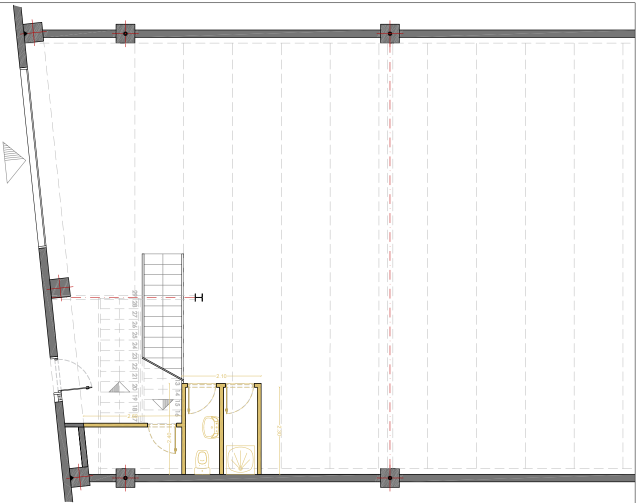
PLANTA ENDERROCS
