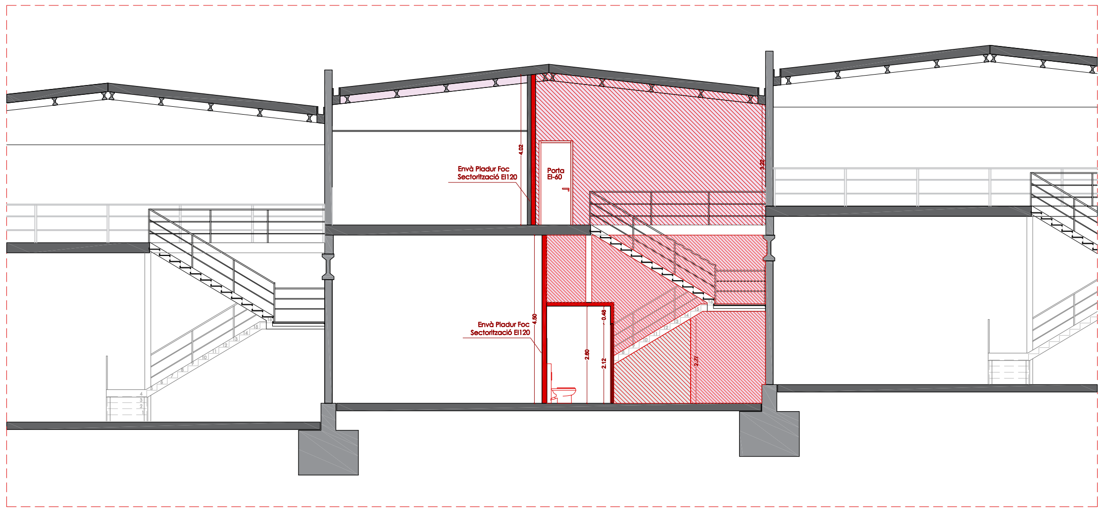
SECCIÓ CC'
