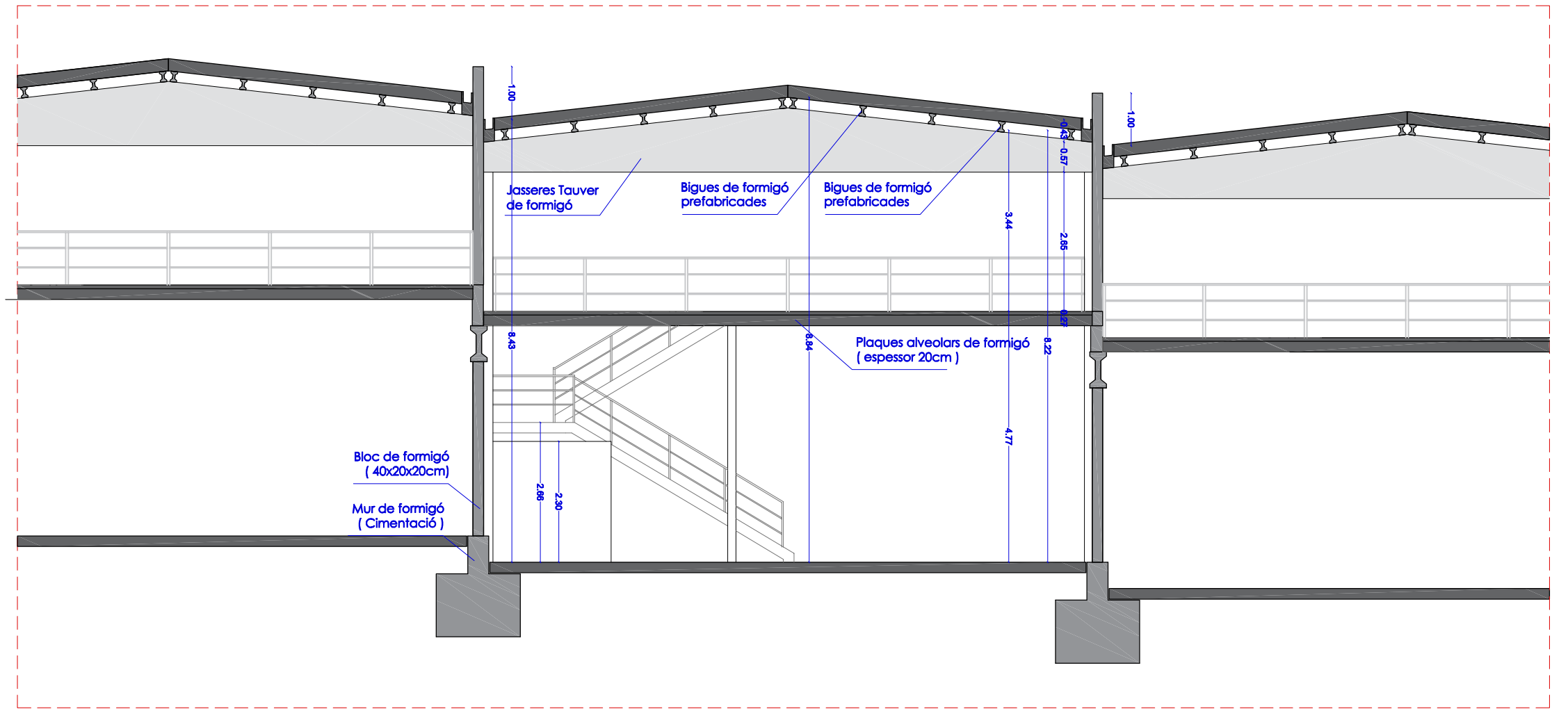
SECCIÓ DD'
