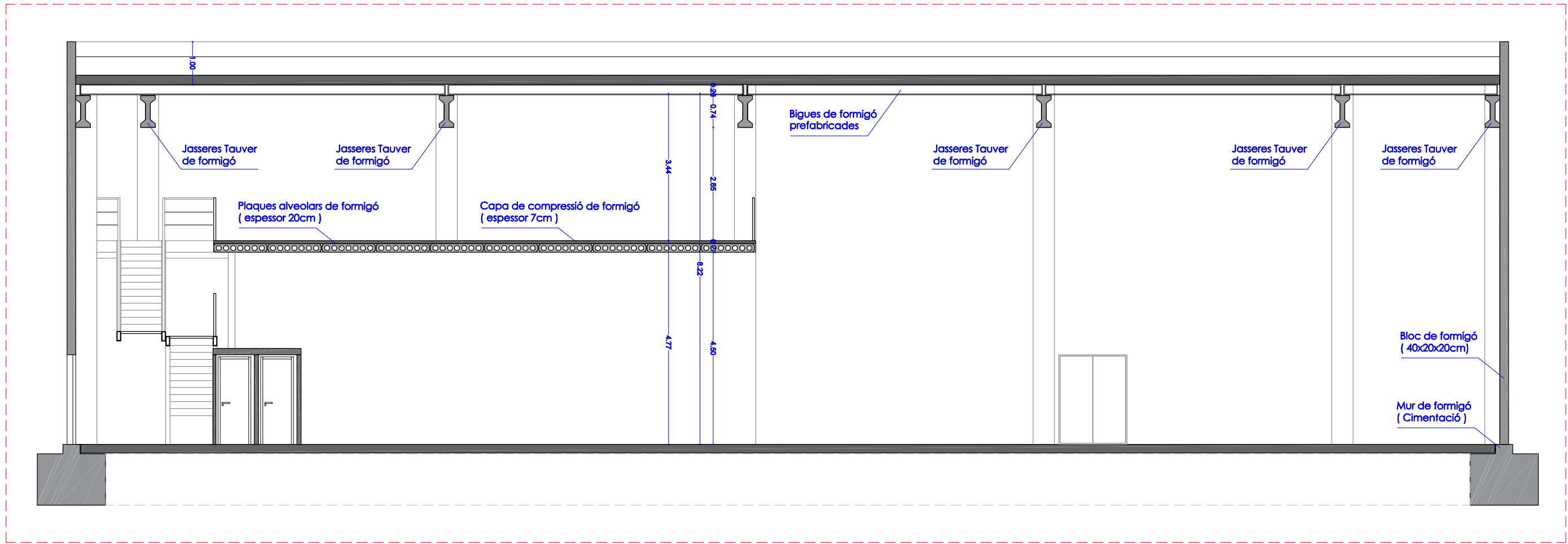
SECCIÓ AA'
