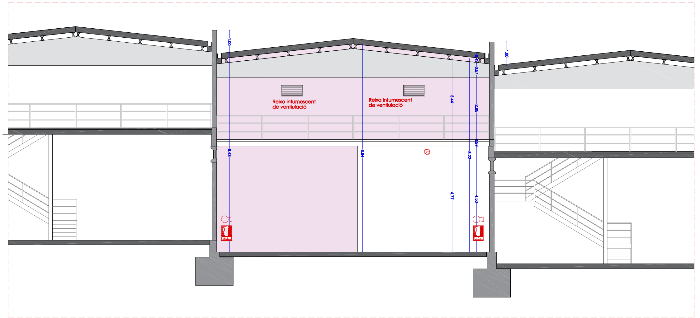
SECCIÓ DD'
