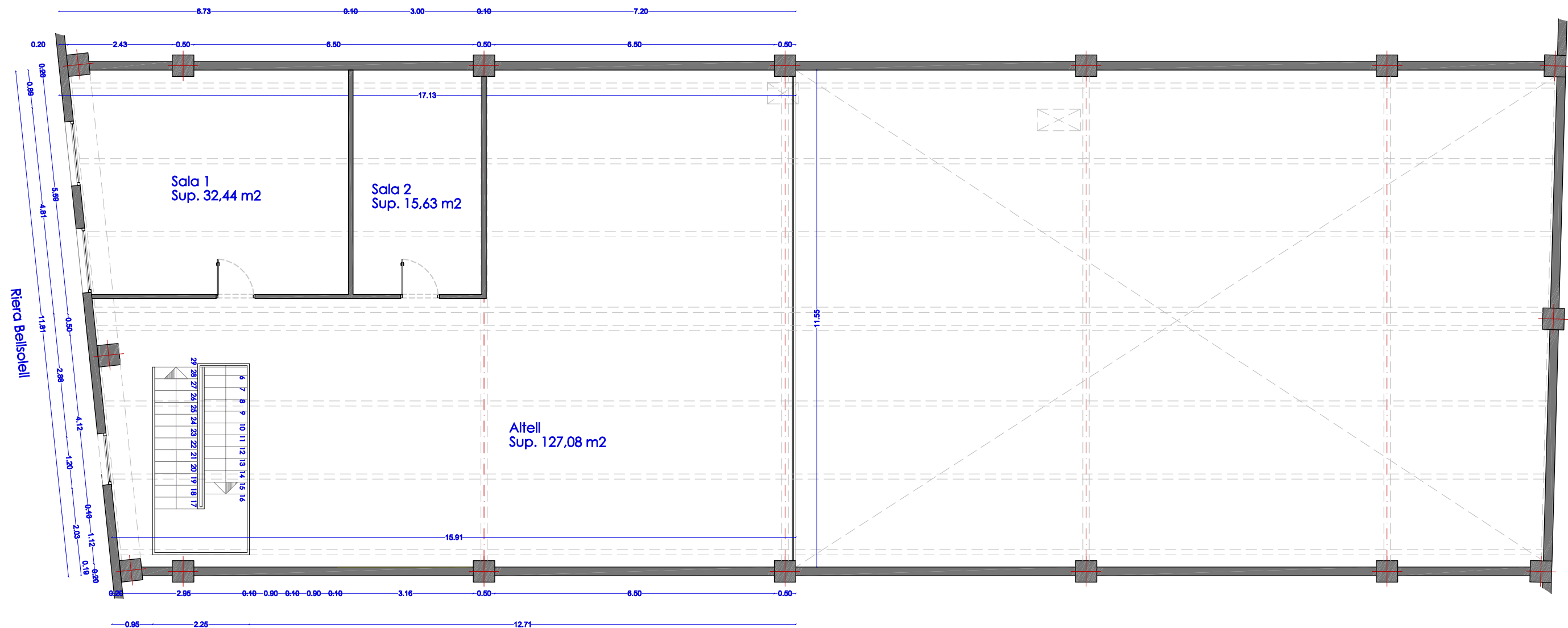
PLANTA ALTELL
