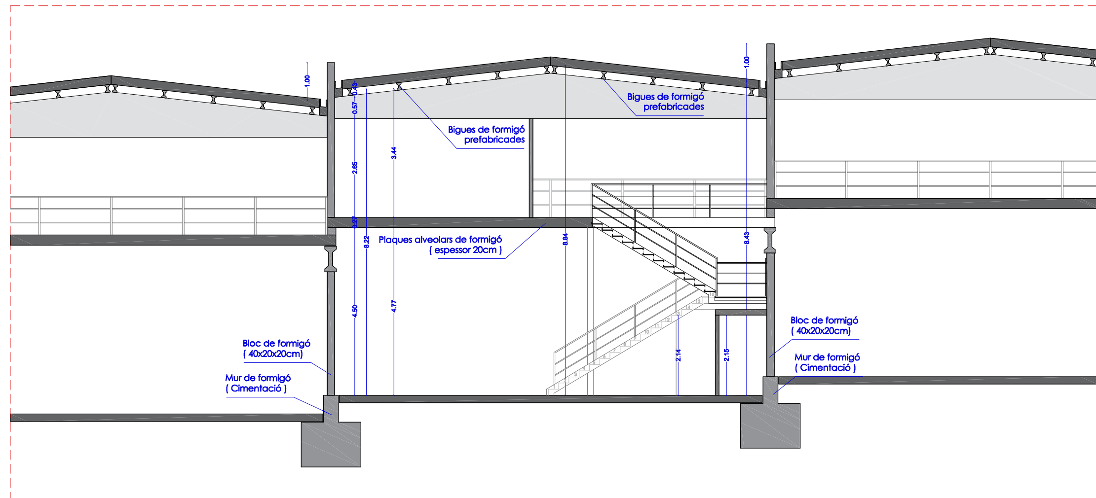
SECCIÓ CC'
