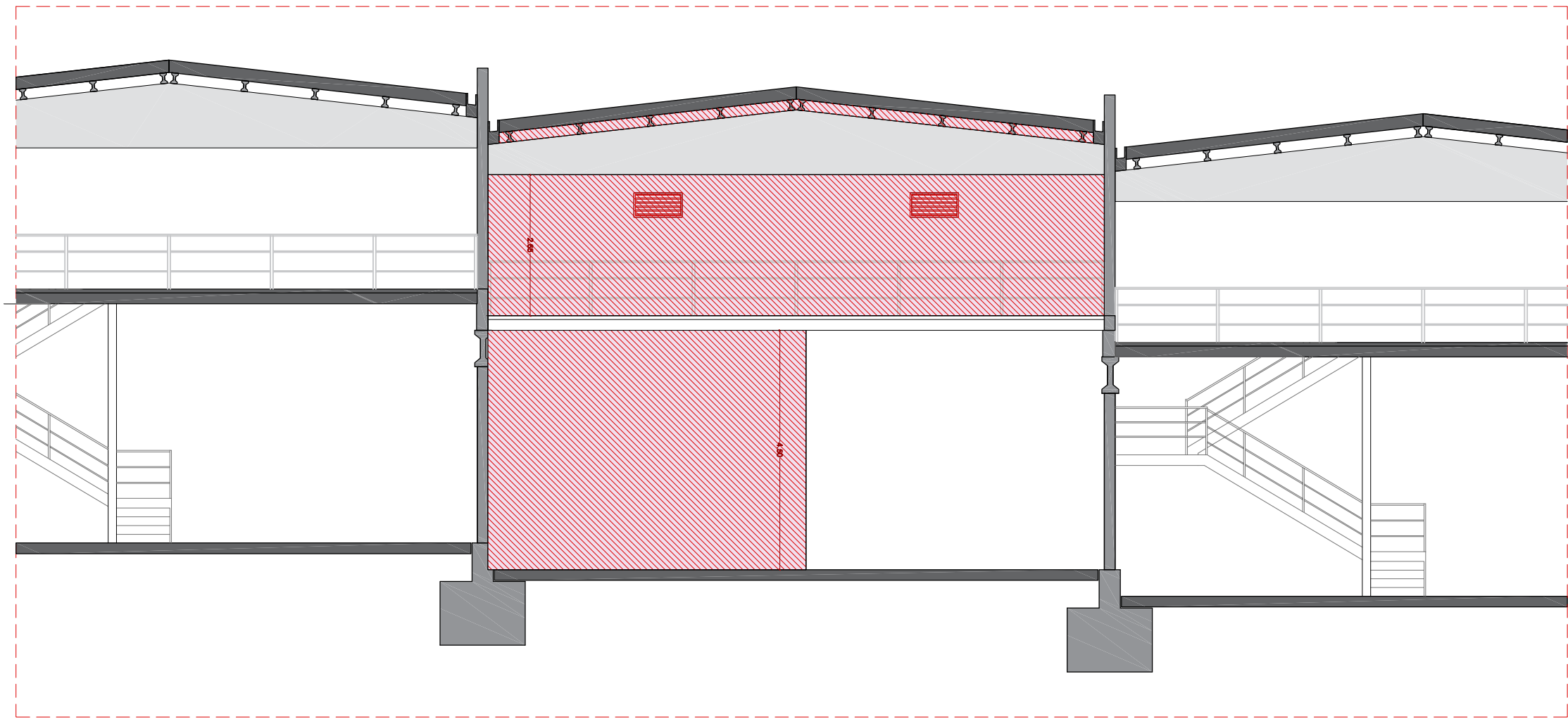
SECCIÓ DD'
