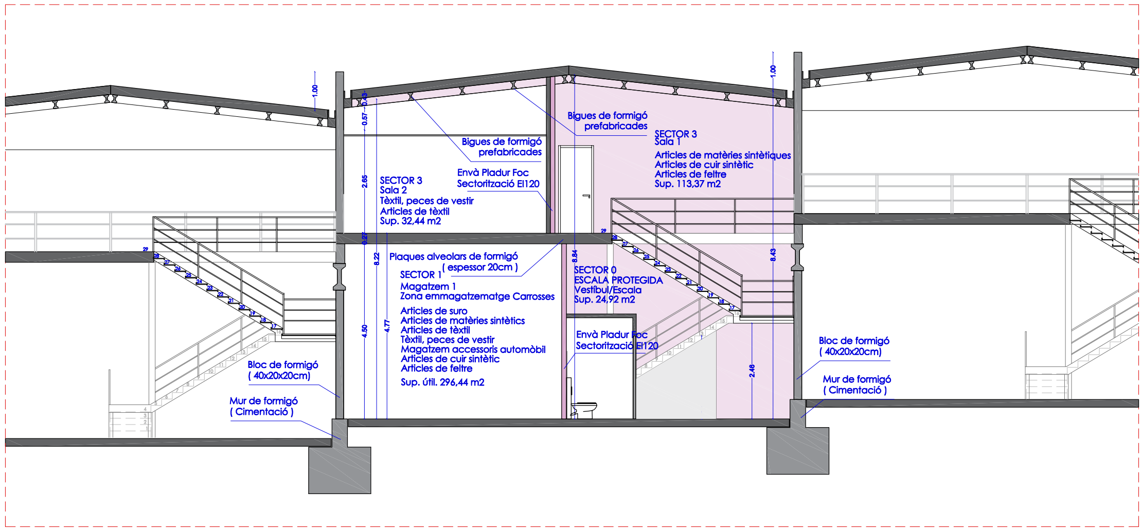
SECCIÓ CC'
