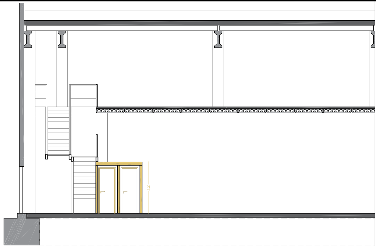
SECCIÓ ENDERROCS
