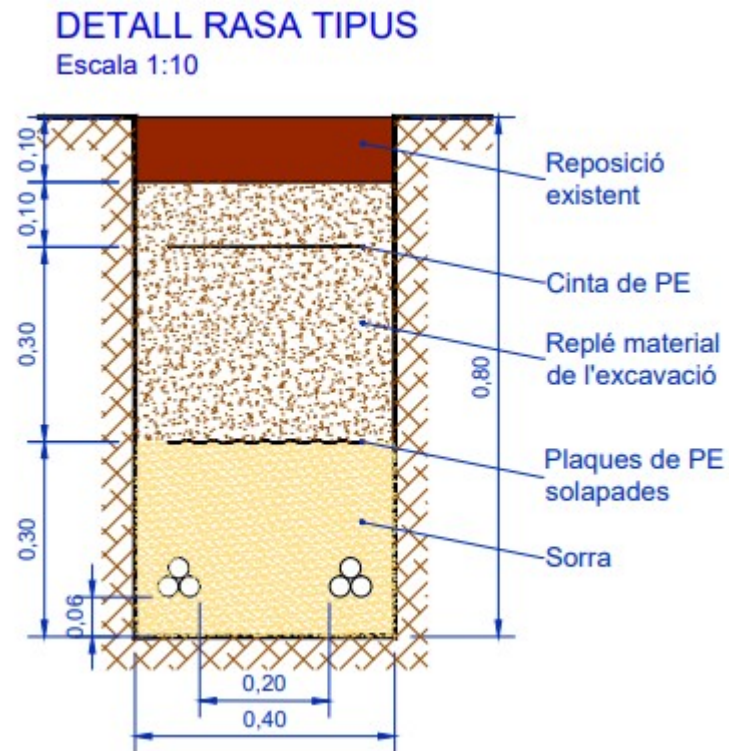
Figura 9.- Detall tipus rasa per cablejat elèctric.
