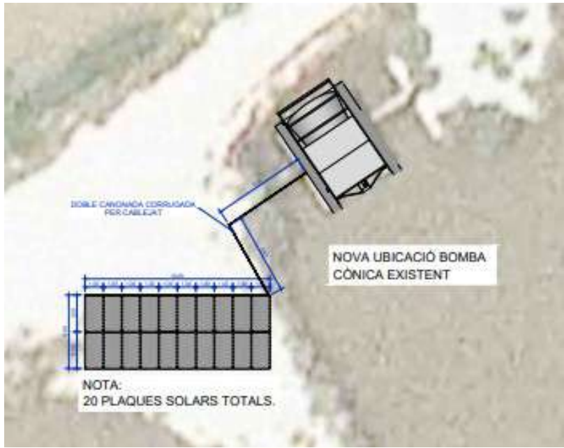
Figura 2.- Emplaçament bombes Circumval·lació . Bomba a traslladar.
