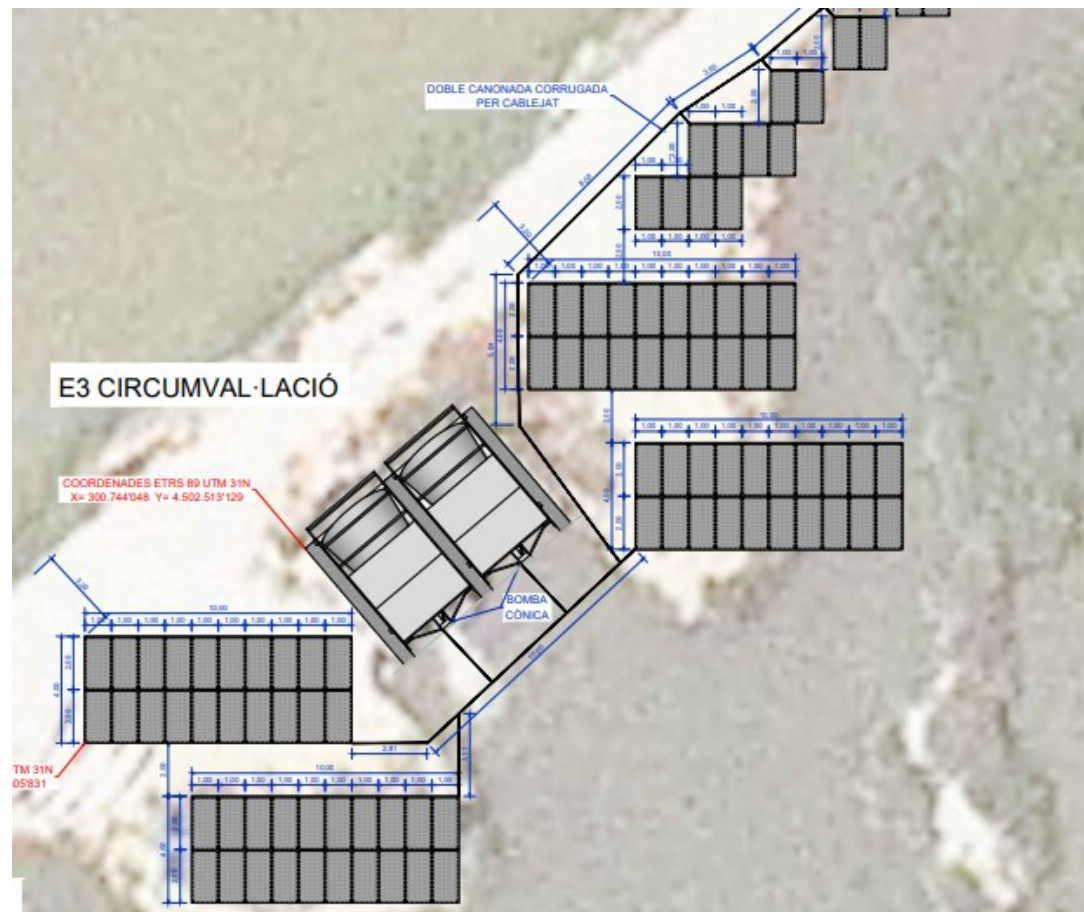
Figura 3.- Nou sistema de bombeig E3 Circumval·lació.
