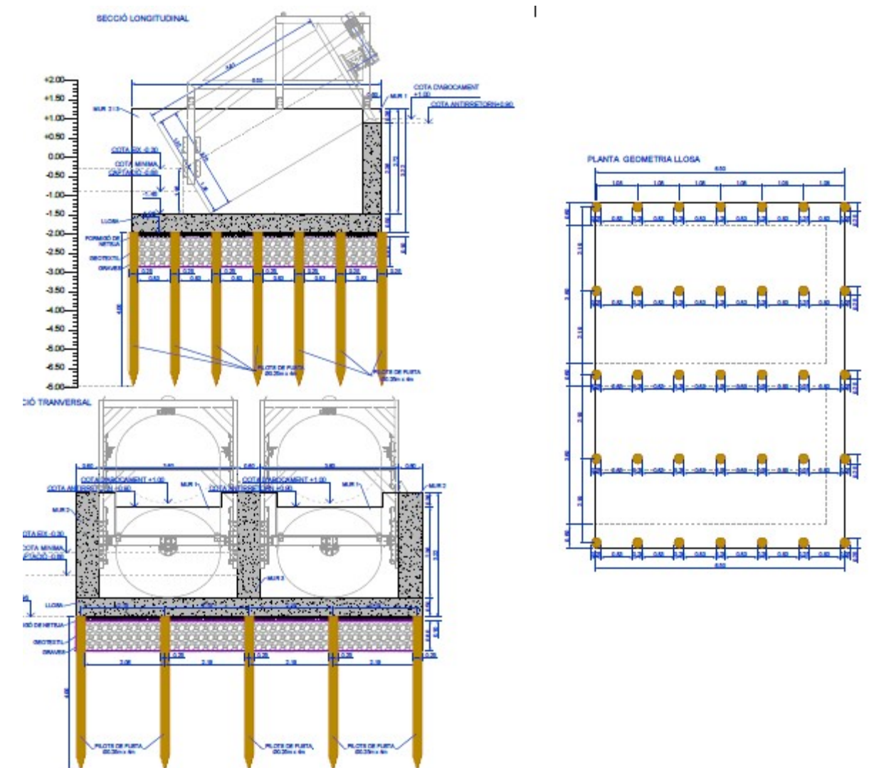
Figura 8.- Estructura de formigó i pilotatge E2 Olles.
