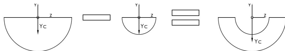
Figura 9.- Càlcul del centroides.
