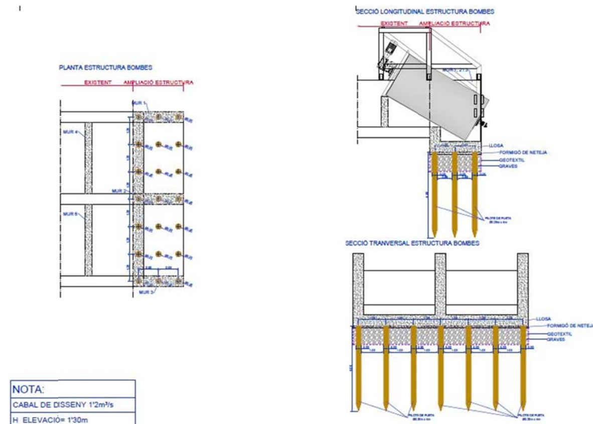
Figura 15.- Estructura de formigó i pilotatge E2 Olles.
