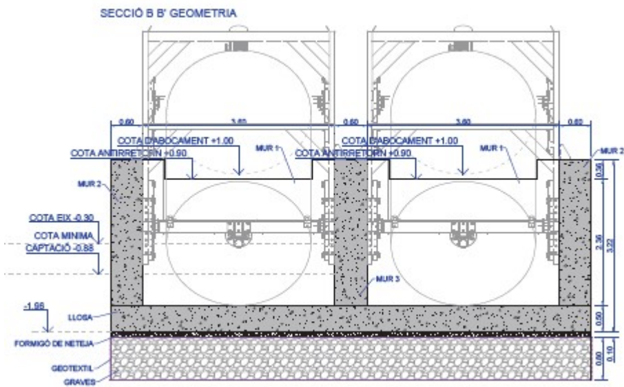
Figura 1.- Estructura bombes.
