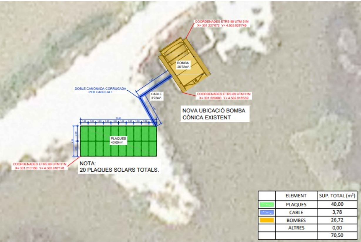
Figura 2.- Sistema de bombeig existent en ubicació definitiva.
