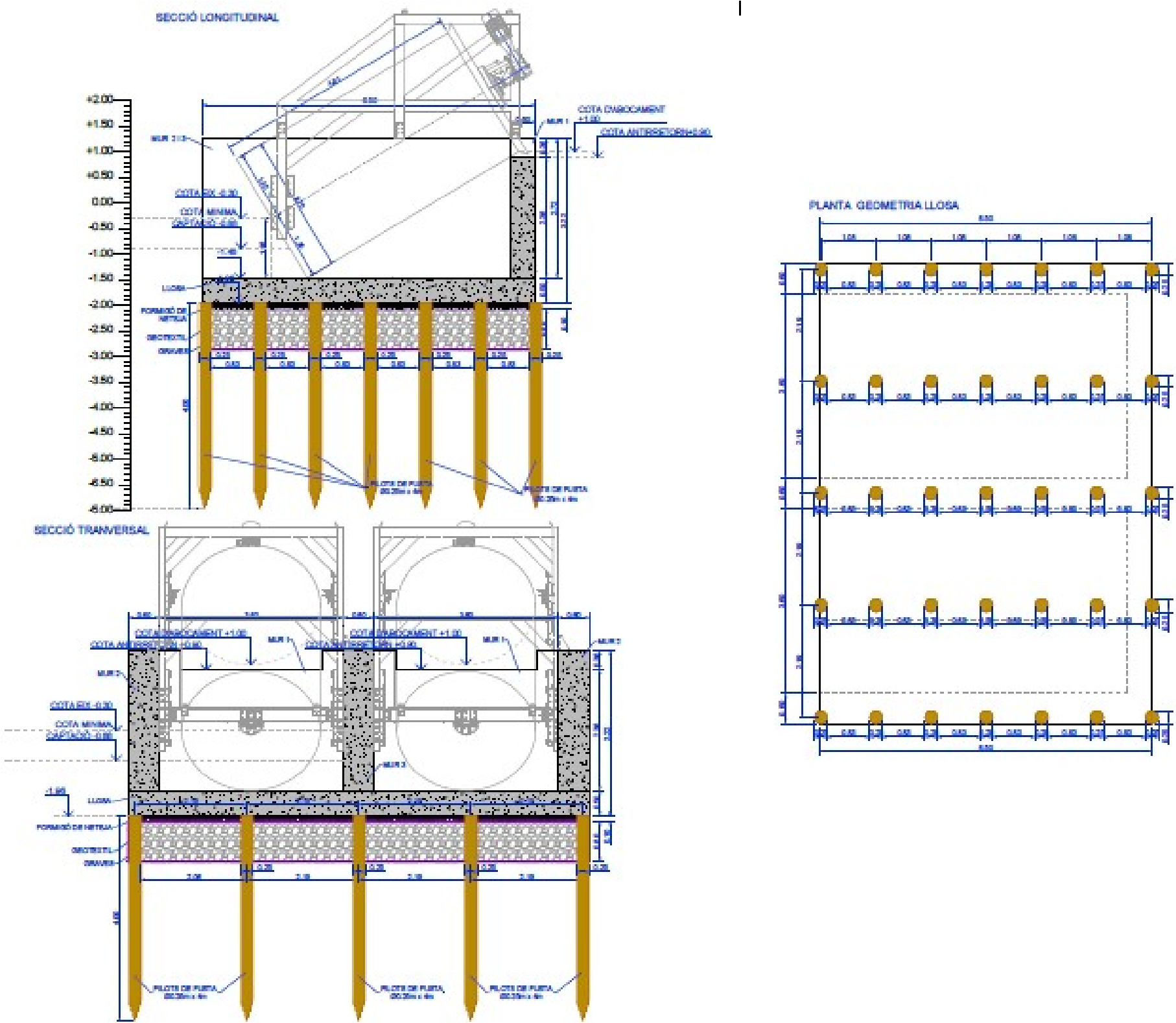
Figura 4.- Pilotatges estructura bombes.
