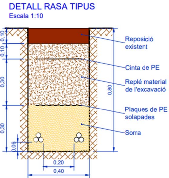
Figura 16.- Detall tipus rasa per cablejat elèctric.
