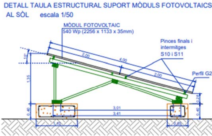
Figura 12.- Plaques solars i estructura.
