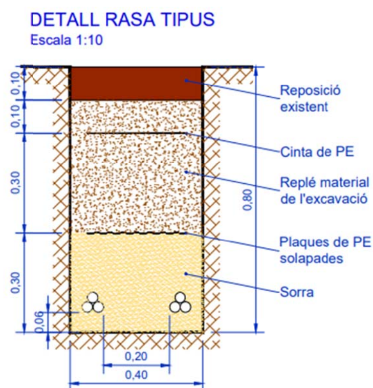
Figura 13.- Detall tipus rasa per cablejat elèctric.
