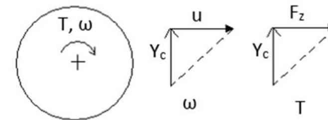
Figura 8.- Velocitat angular i par a l'eix.
