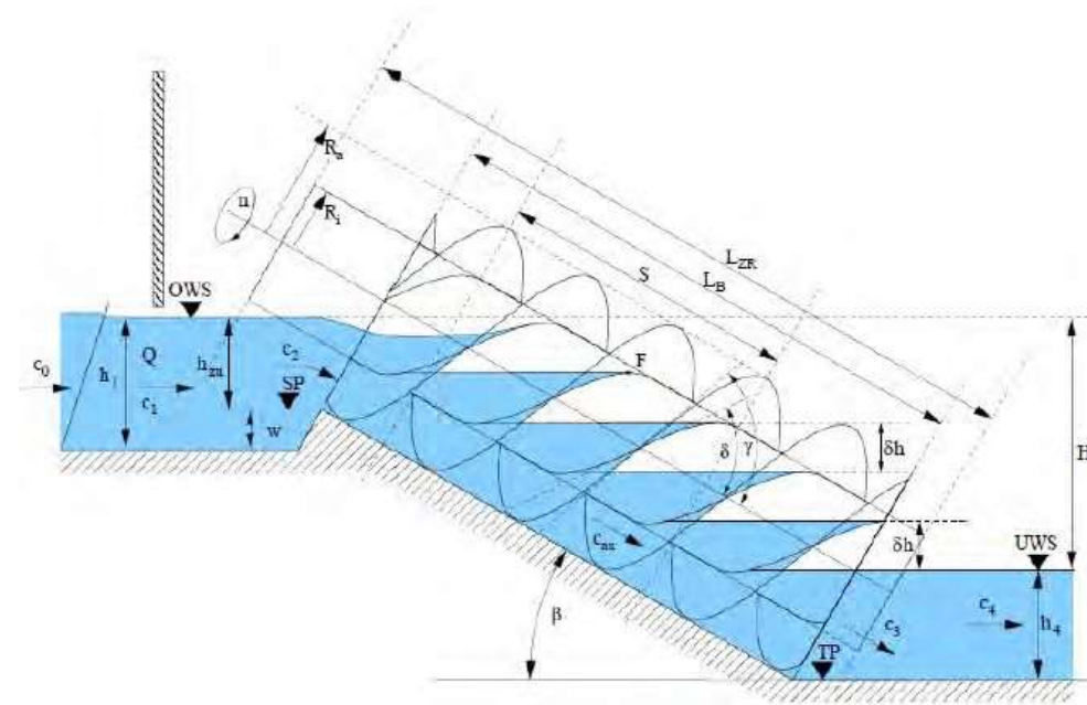
Figura 2.- Vista de perfil d'un cargol d'Arquímedes.
