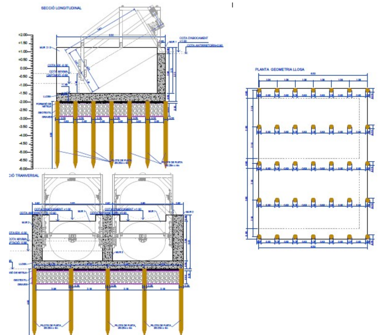
Figura 4.- Estructura de formigó i pilotatge E3 Circumval·lació.
