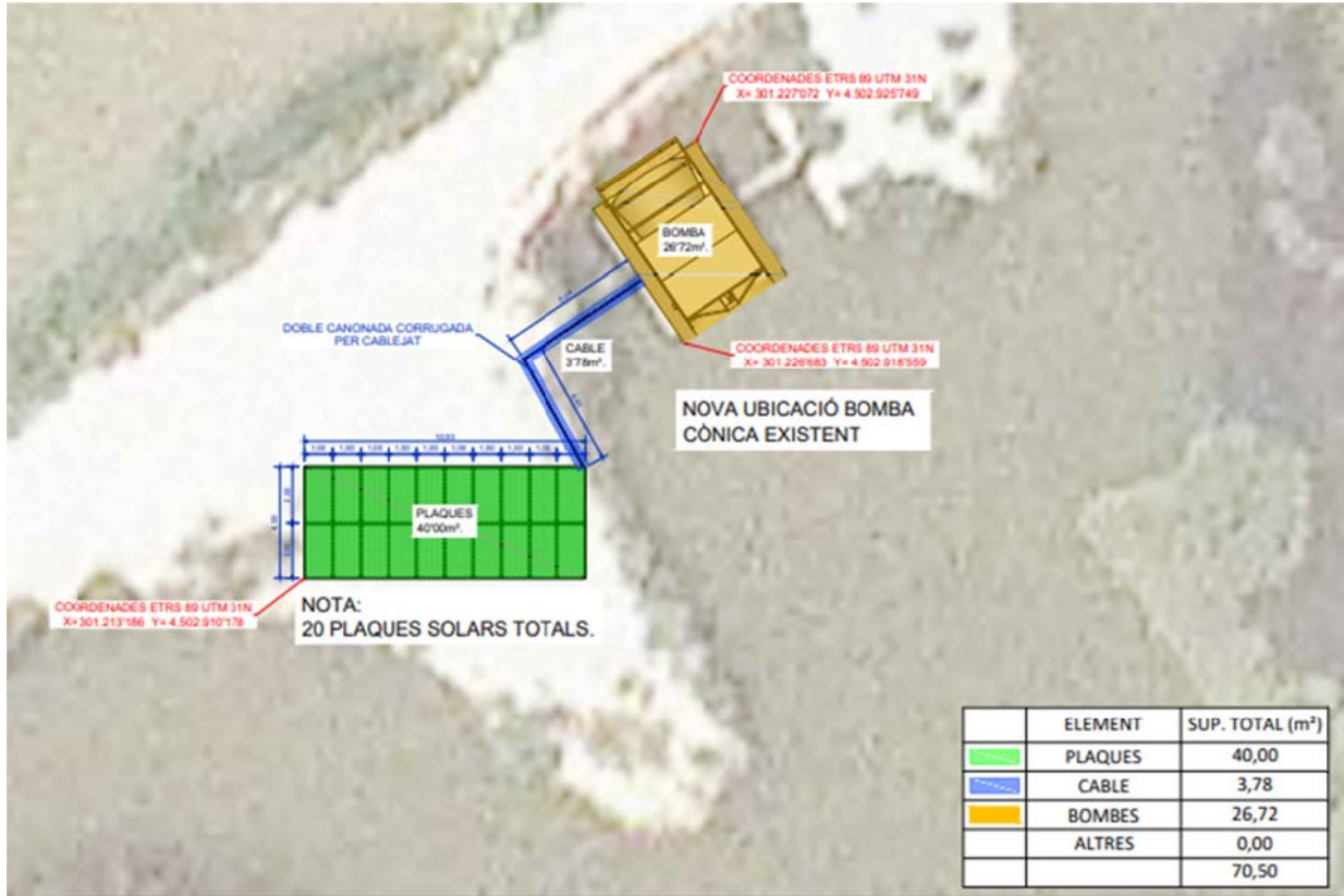
Figura 9.- Sistema de bombeig existent en ubicació definitiva.
