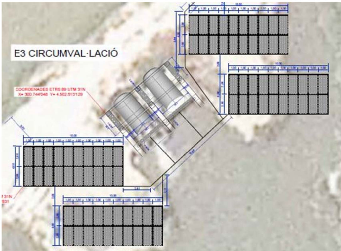
Figura 10.- Nou sistema de bombeig E3 Circumval·lació.
