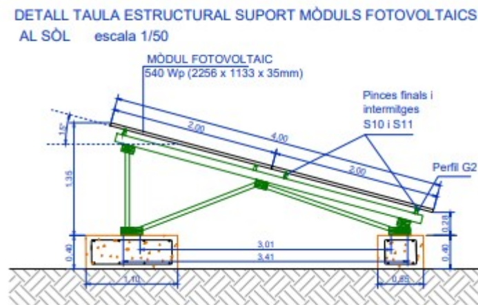
Figura 5.- Plaques solars i estructura..
