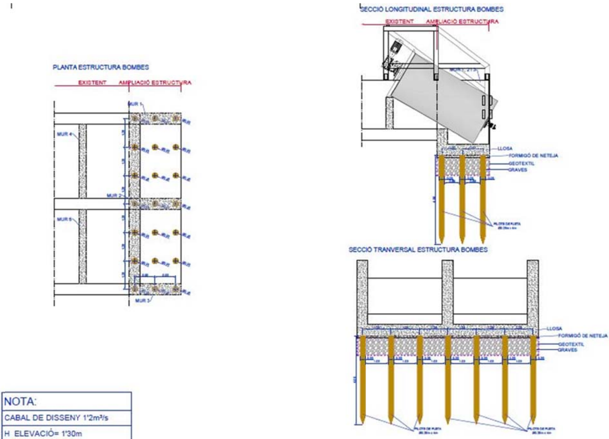
Figura 11.- Estructura de formigó i pilotatge E3 Circumval·lació.
