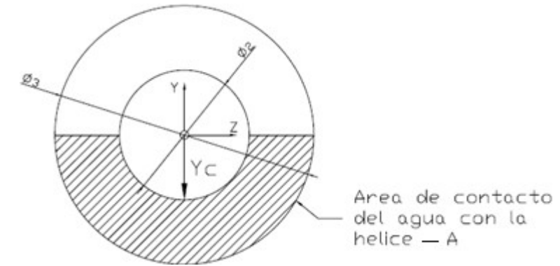
Figura 7.- 50% d'aigua a l'hèlix.
