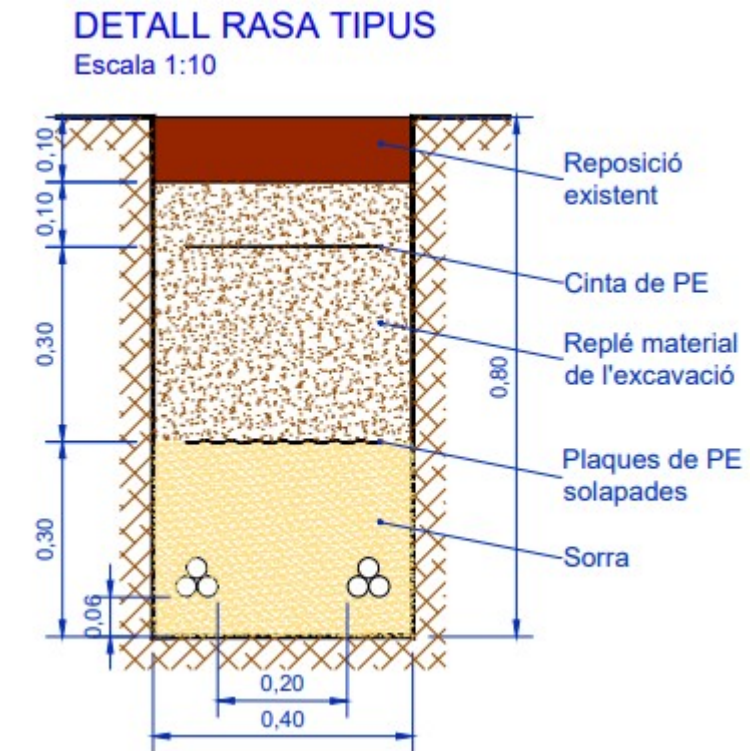
Figura 6.- Detall tipus rasa per cablejat elèctric.
