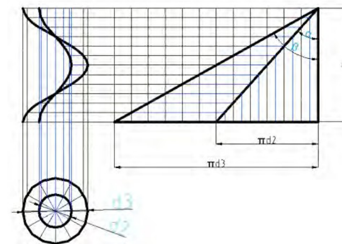
Figura 6.- Desarrollo de les hèlix d'un cargol d'Arquímedes.
