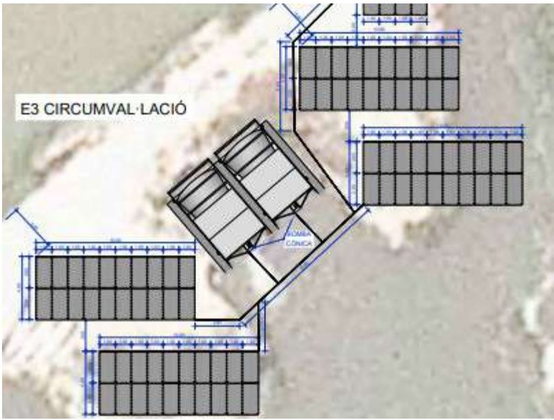
Figura 3.- Emplaçament bombes Circumval·lació. Nou sistema de bombeig.
