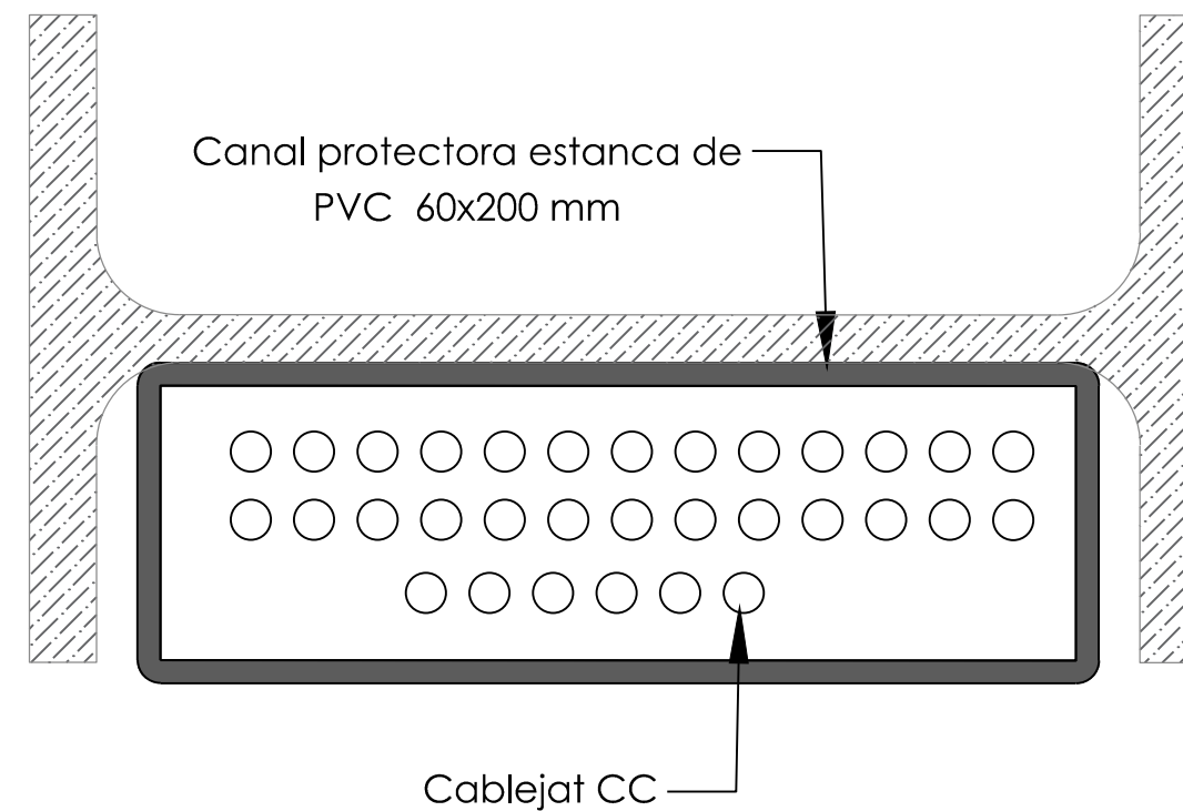
Secció A-A'
