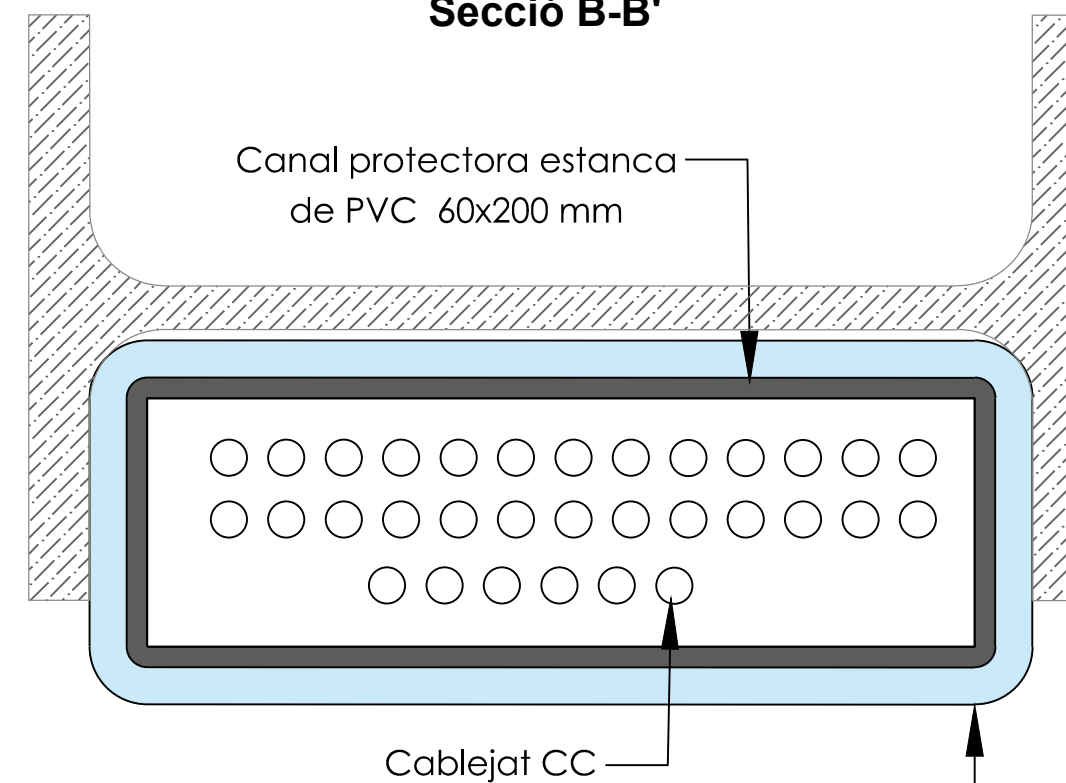
Secció B-B'
