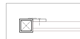
UNIONS PLAFÓ DE MDF I ESTRUCTURA TUBULAR A3 1:5
