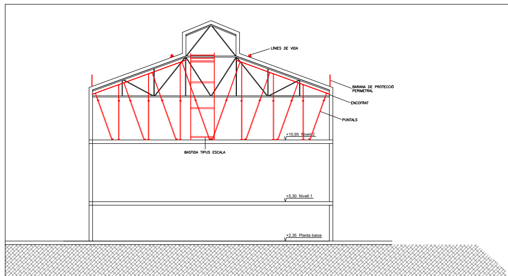
SECCIÓ B-B'
