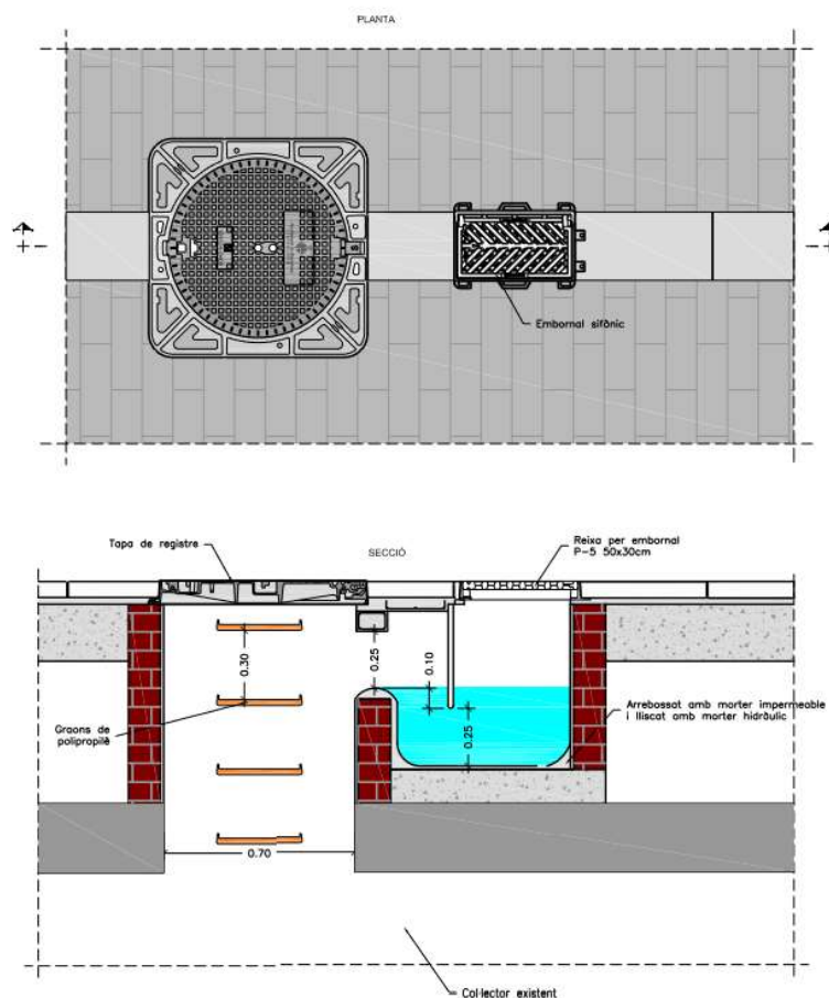
Figura 4. Detall de connexió d'embornal sifònic sobre la vertical del col·lector
