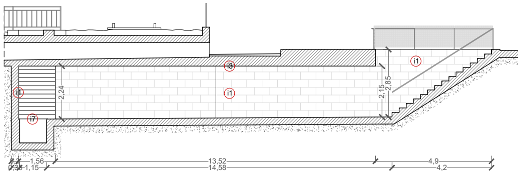
SECCIÓ A
