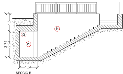
SECCIÓ B
