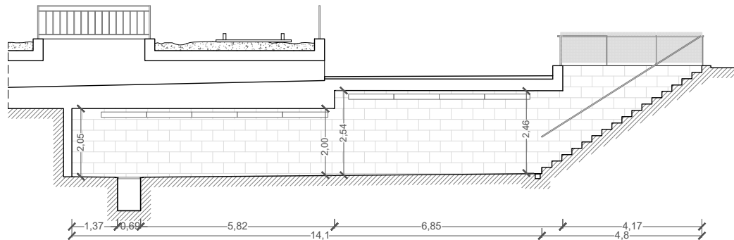
SECCIÓ A
