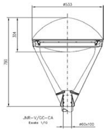
Junior con cúpula alta y vidrio lenticular
