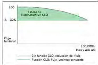
Gráfico de flujo luminoso
