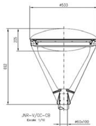
Junior con cúpula baja y vidrio lenticular
