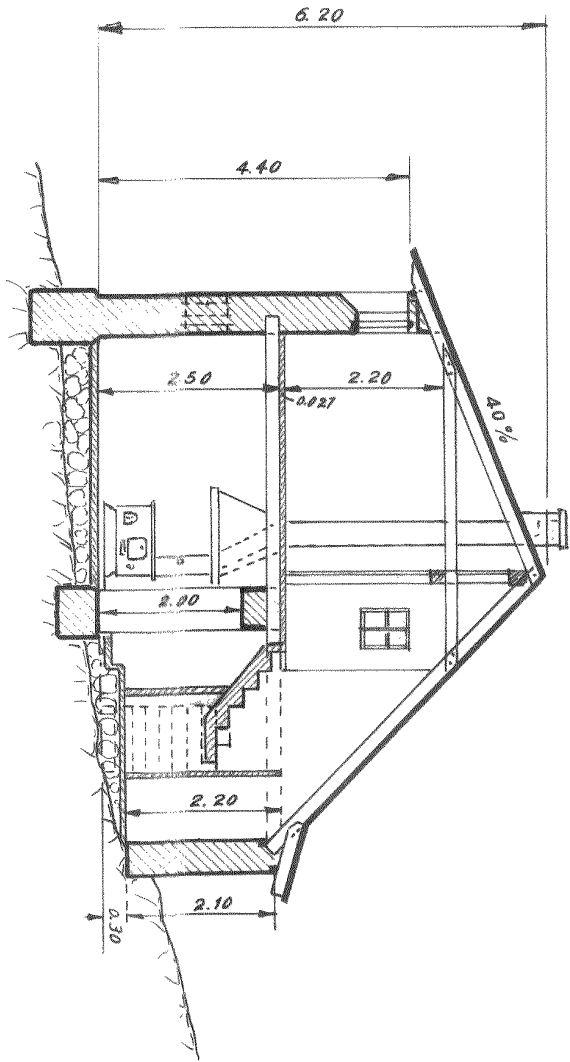
SECCIÓ C-C
