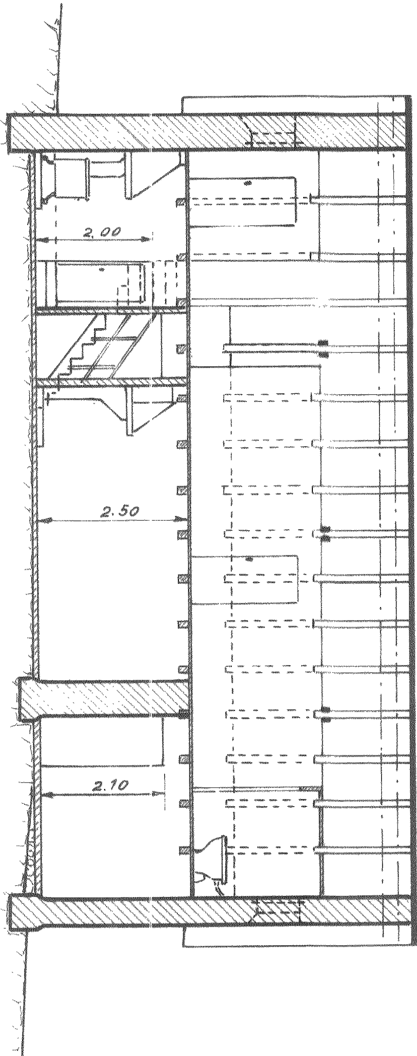
SECCIÓ LONGITUDINAL B-B
