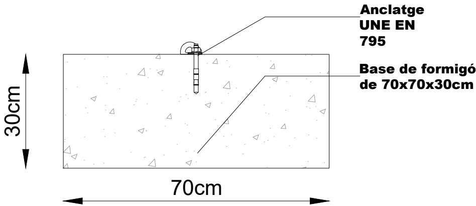
SECCIÒ
