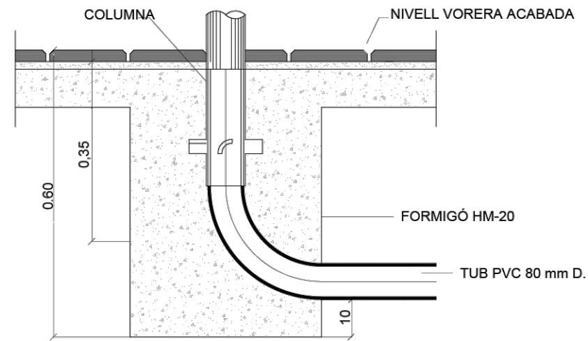
ALÇAT-SECCIÓ
