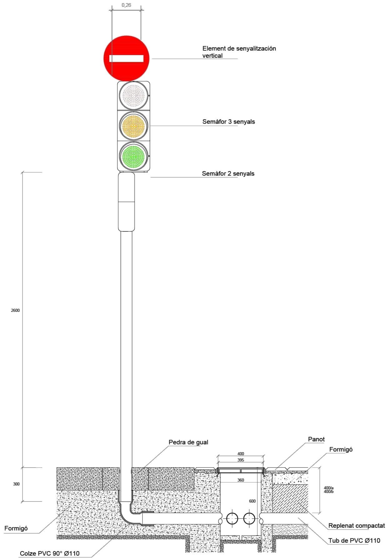
CIMENTACIONS I ANCORATGES DE COLUMNS EN GUAL DE PEDRA EXEMPLE D'ELEMENT ADOSSAT A SEMÀFOR
