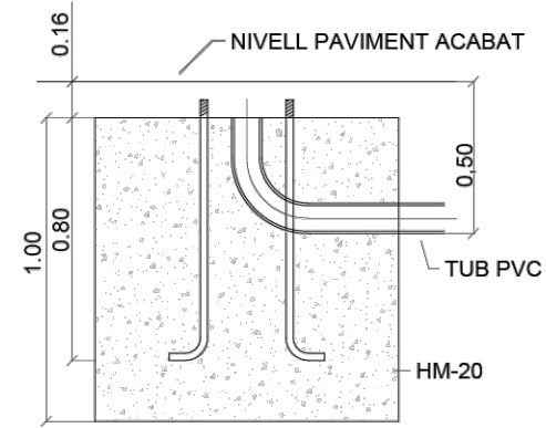
ALÇAT-SECCIÓ
