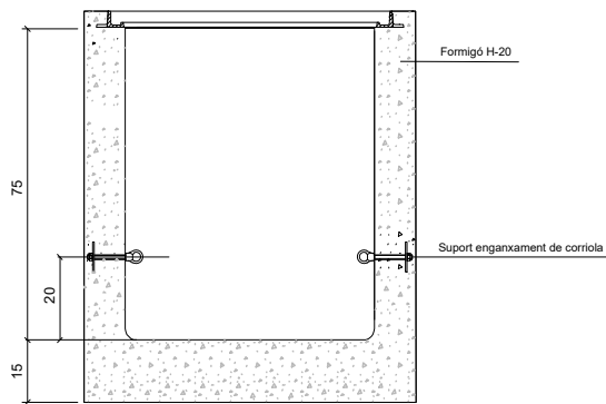
ALÇAT
