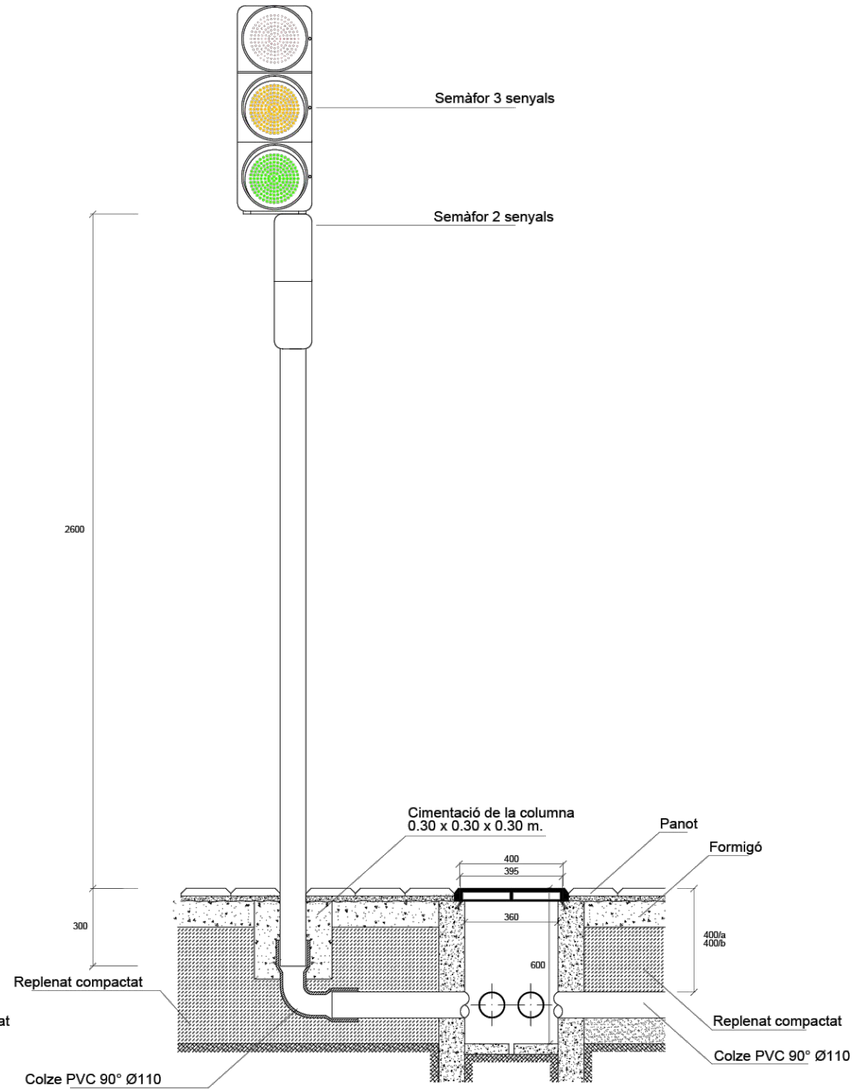
CIMENTACIÓ Y ANCORATGE DE COLUMNS EN PAVIMENT DE PANOT
