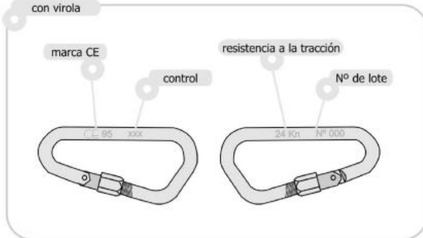
con virola
