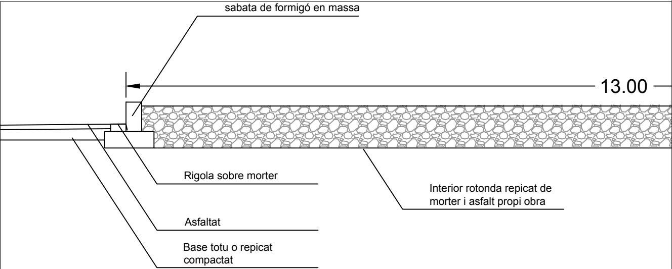
Detall Rotonda Carrer Victor Català
