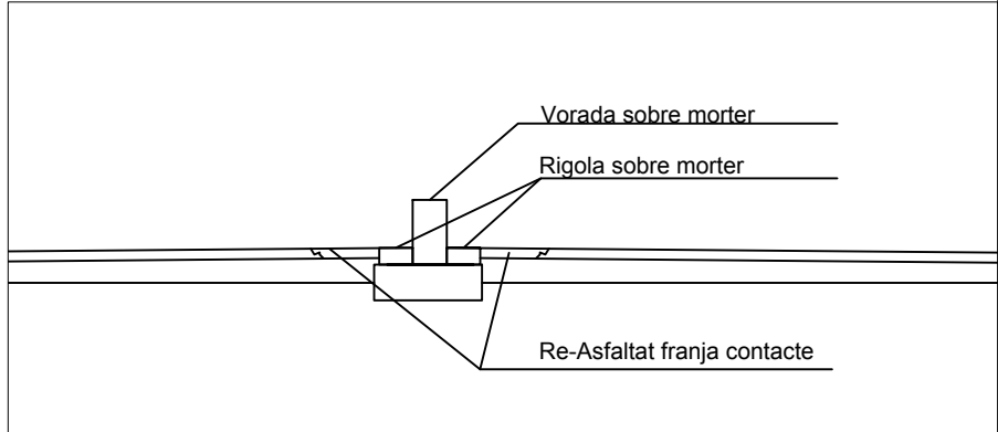
Detall noves separaficions entre calçades
